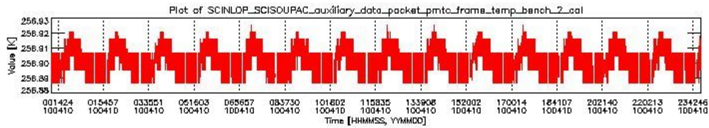
sciamachy_daily_report_level0_Any_version_20100410_1.PNG
