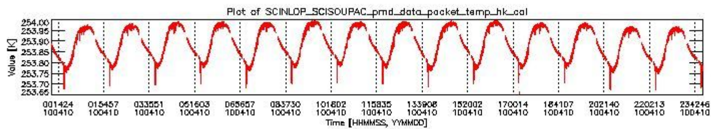
sciamachy_daily_report_level0_Any_version_20100410_3.PNG
