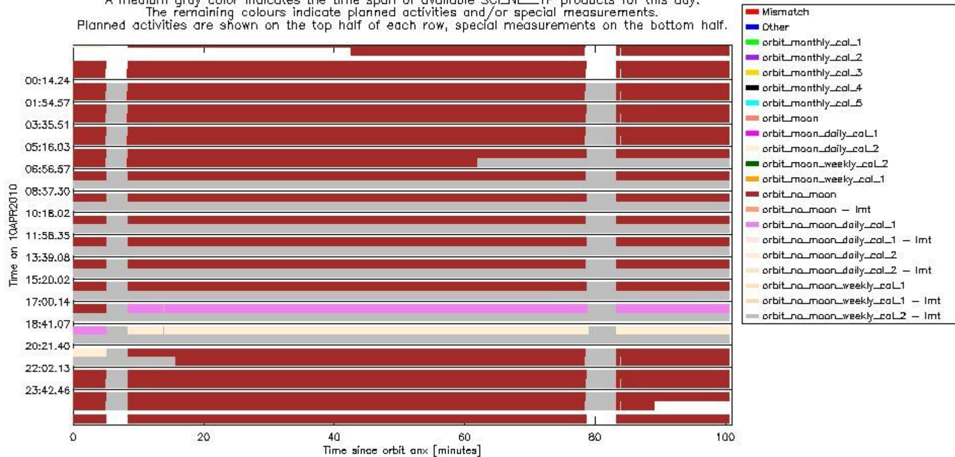
sciamachy_daily_report_level0_Any_version_20100410_6.PNG
