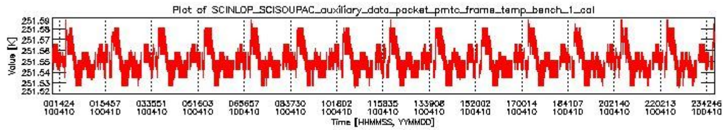
sciamachy_daily_report_level0_Any_version_20100410_0.PNG
