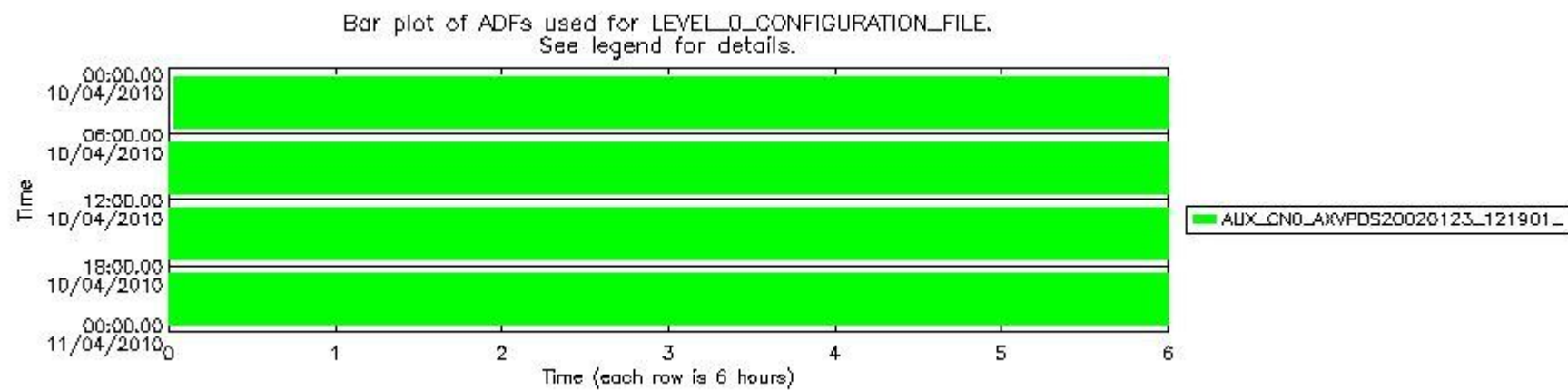
sciamachy_daily_report_level0_Any_version_20100410_7.PNG
