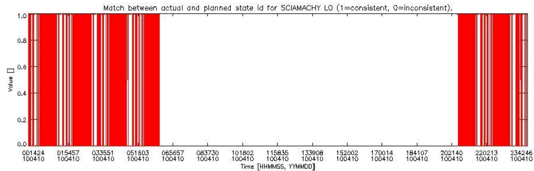
sciamachy_daily_report_level0_Any_version_20100410_5.PNG
