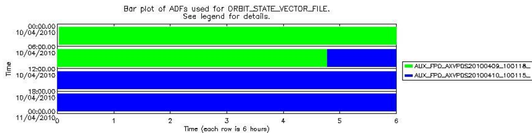
sciamachy_daily_report_level0_Any_version_20100410_8.PNG
