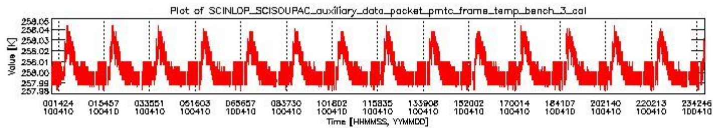
sciamachy_daily_report_level0_Any_version_20100410_2.PNG
