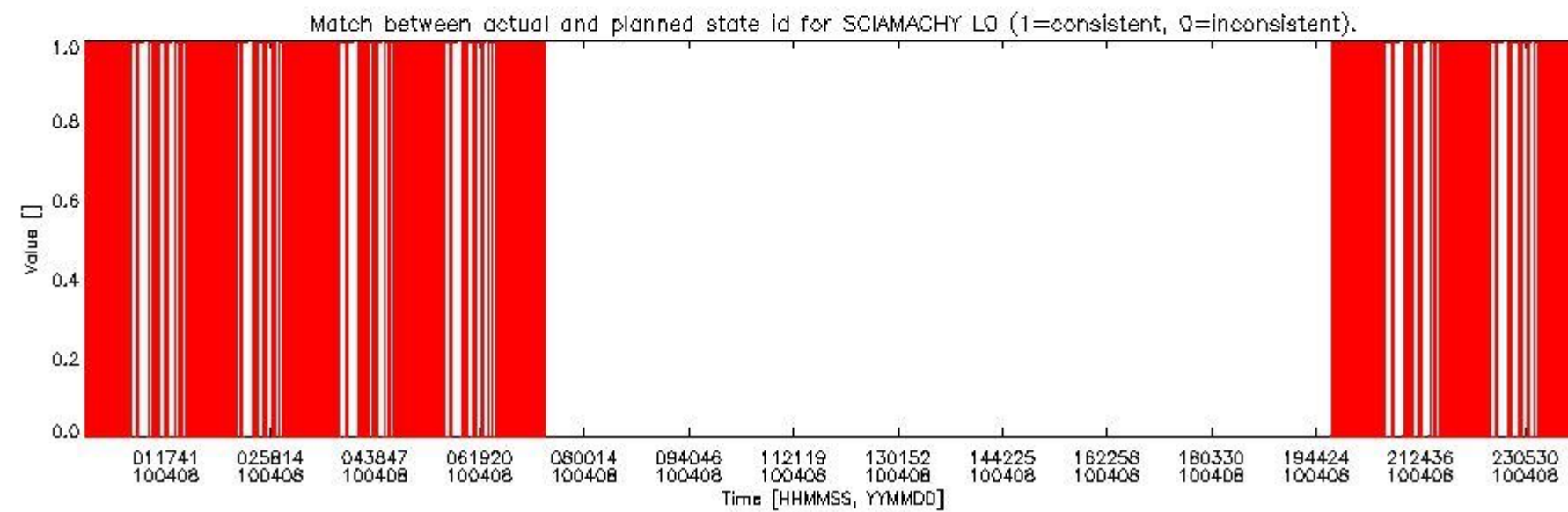
sciamachy_daily_report_level0_Any_version_20100408_5.PNG
