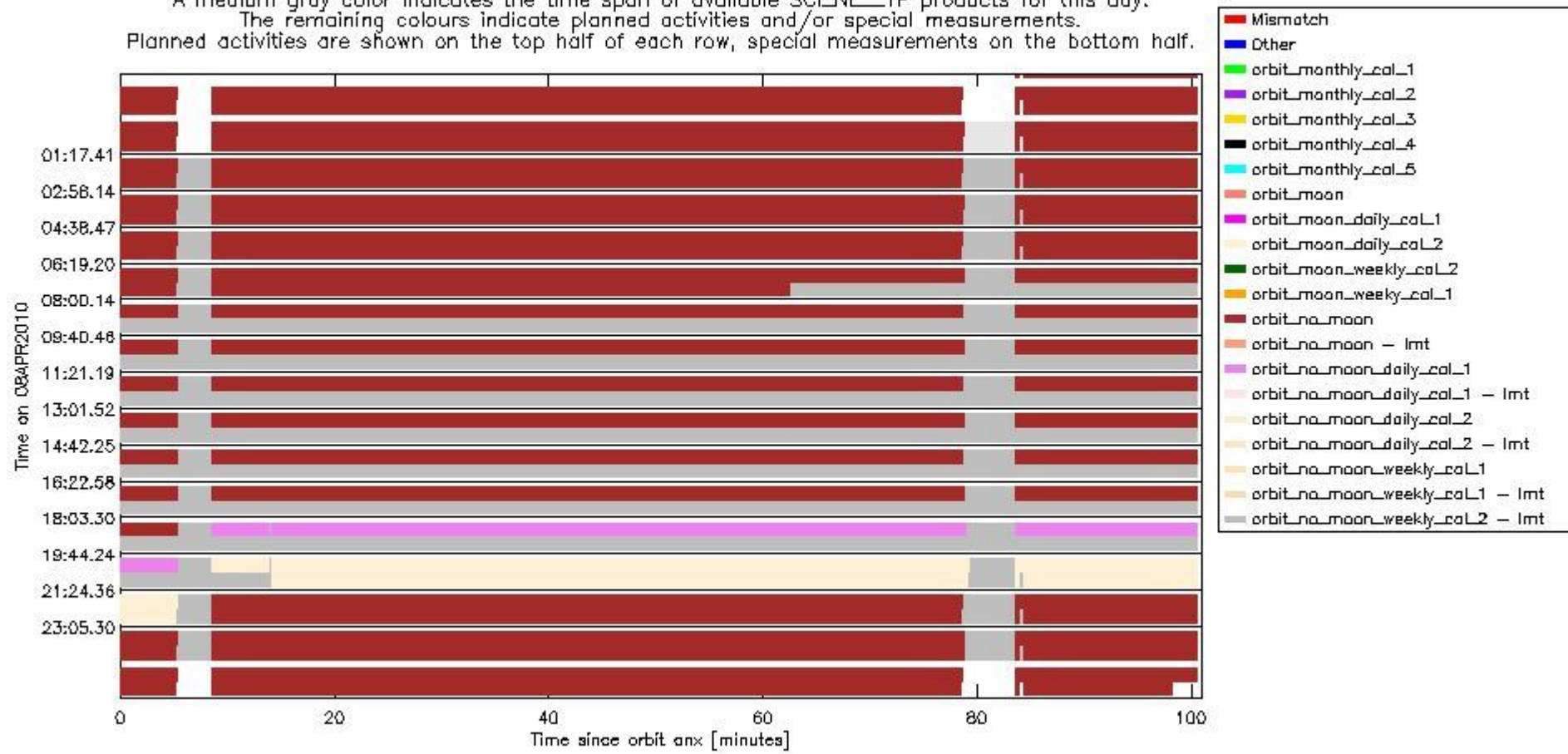
sciamachy_daily_report_level0_Any_version_20100408_6.PNG
