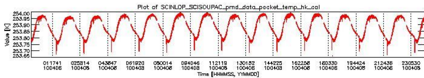
sciamachy_daily_report_level0_Any_version_20100408_3.PNG
