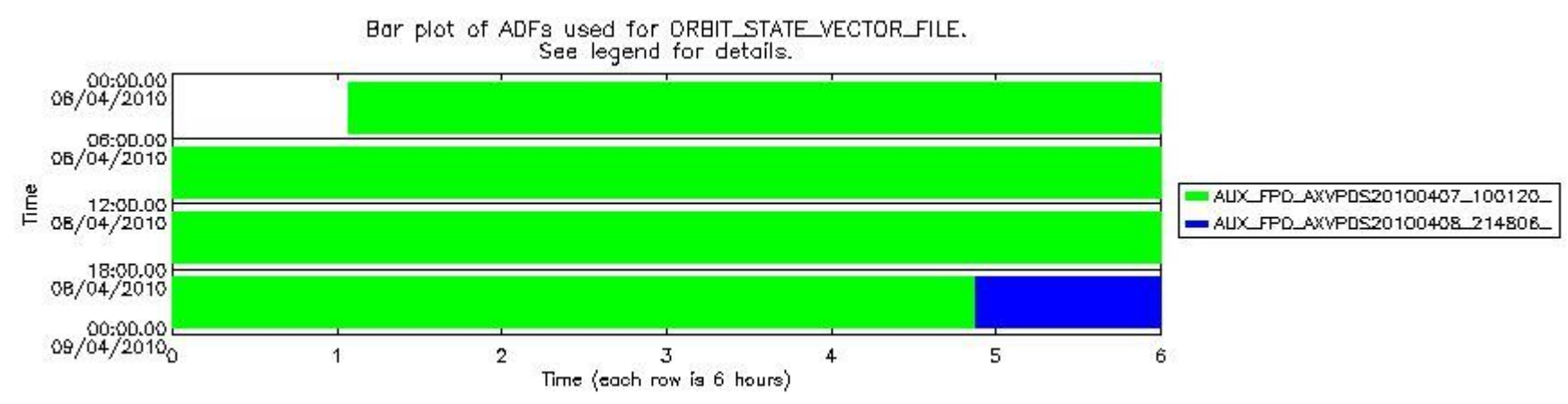
sciamachy_daily_report_level0_Any_version_20100408_8.PNG
