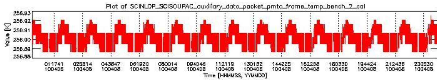
sciamachy_daily_report_level0_Any_version_20100408_1.PNG
