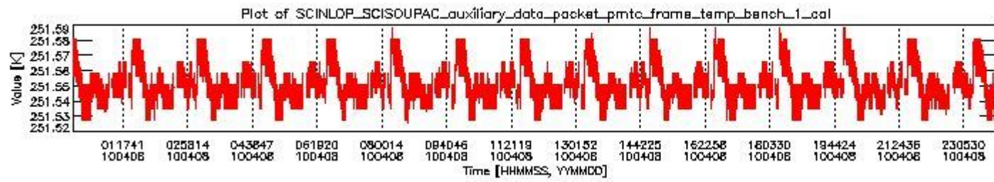
sciamachy_daily_report_level0_Any_version_20100408_0.PNG
