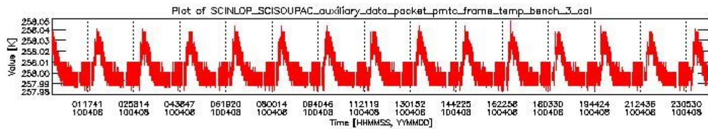
sciamachy_daily_report_level0_Any_version_20100408_2.PNG
