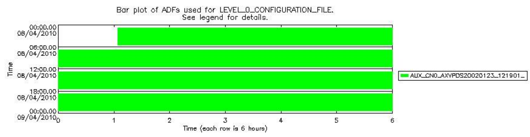
sciamachy_daily_report_level0_Any_version_20100408_7.PNG
