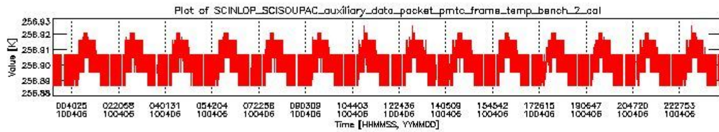
sciamachy_daily_report_level0_Any_version_20100406_1.PNG
