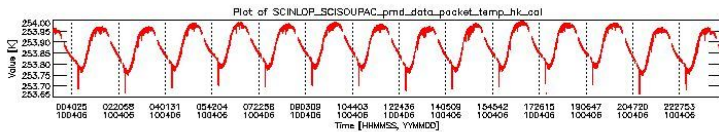
sciamachy_daily_report_level0_Any_version_20100406_3.PNG
