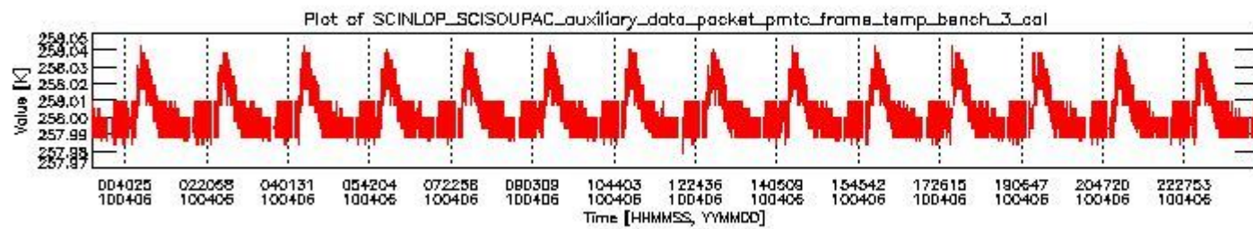
sciamachy_daily_report_level0_Any_version_20100406_2.PNG
