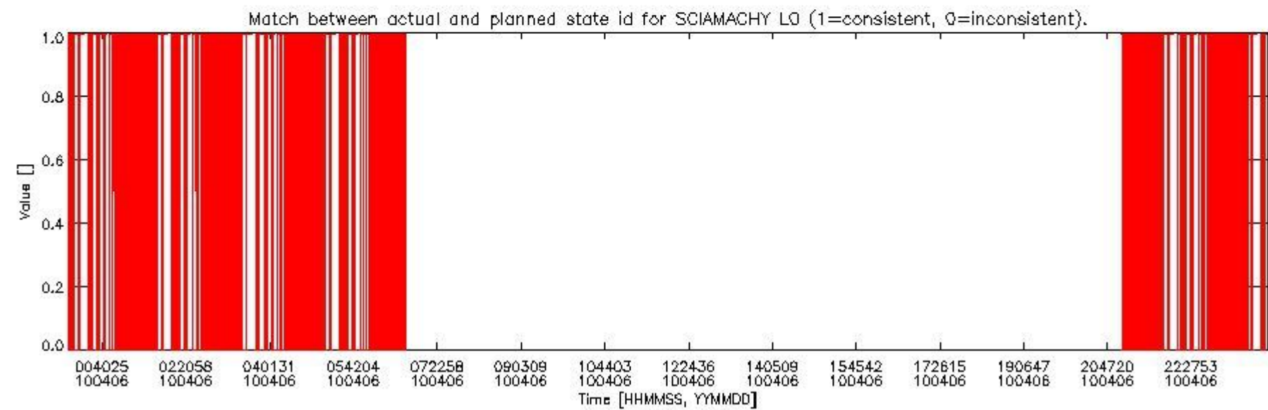
sciamachy_daily_report_level0_Any_version_20100406_5.PNG
