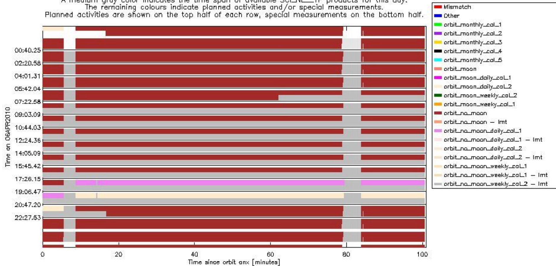
sciamachy_daily_report_level0_Any_version_20100406_6.PNG
