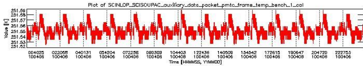
sciamachy_daily_report_level0_Any_version_20100406_0.PNG
