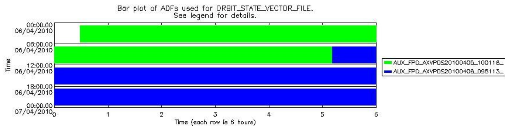
sciamachy_daily_report_level0_Any_version_20100406_8.PNG
