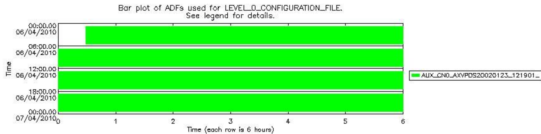
sciamachy_daily_report_level0_Any_version_20100406_7.PNG
