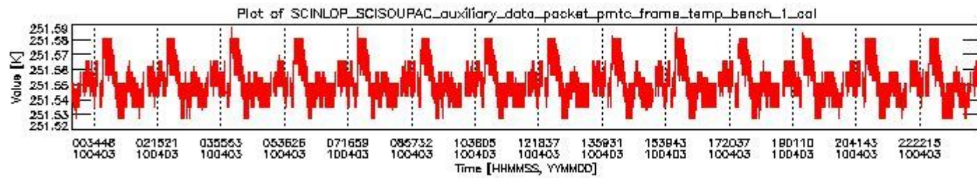
sciamachy_daily_report_level0_Any_version_20100403_0.PNG
