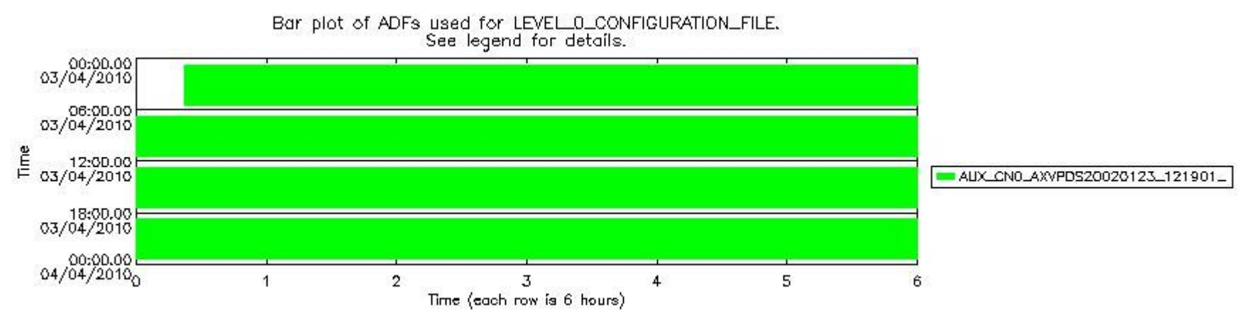
sciamachy_daily_report_level0_Any_version_20100403_7.PNG
