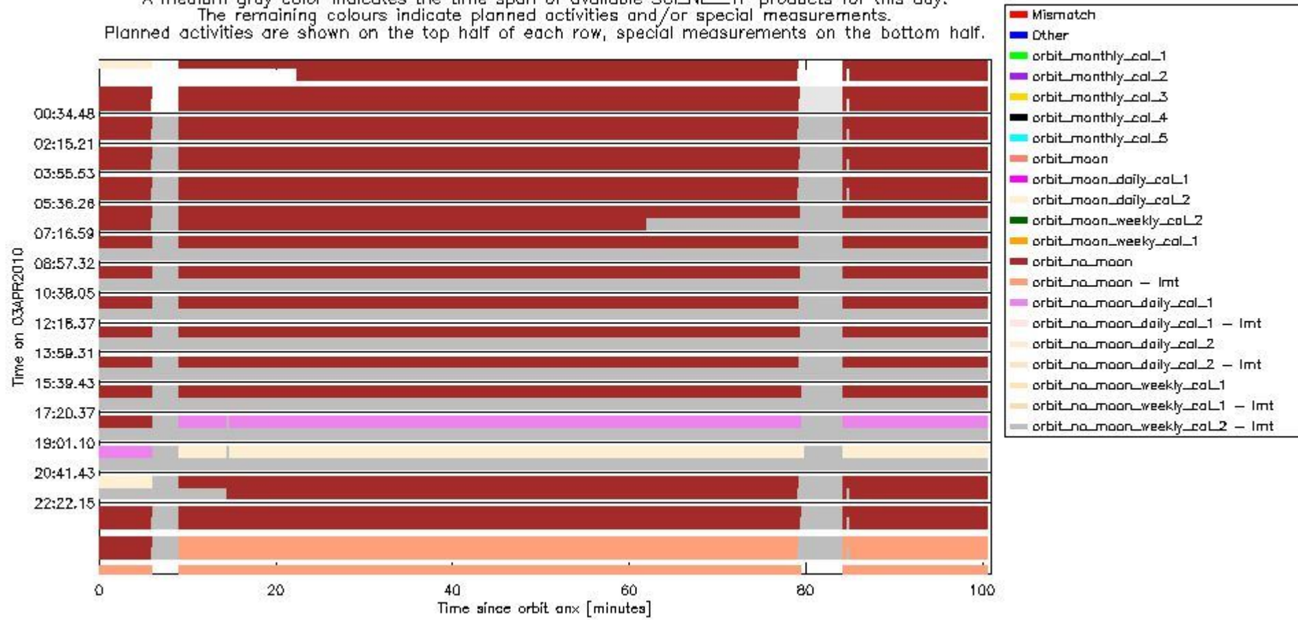
sciamachy_daily_report_level0_Any_version_20100403_6.PNG
