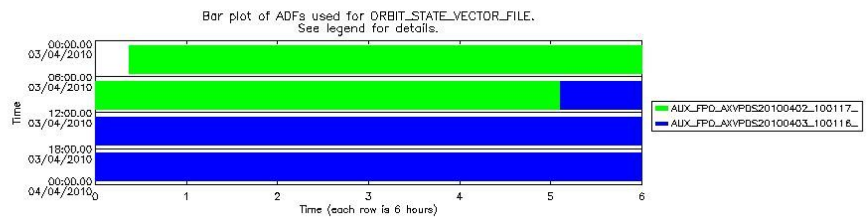
sciamachy_daily_report_level0_Any_version_20100403_8.PNG
