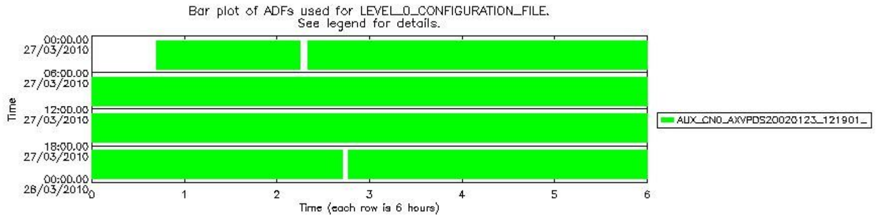
sciamachy_daily_report_level0_Any_version_20100327_7.PNG
