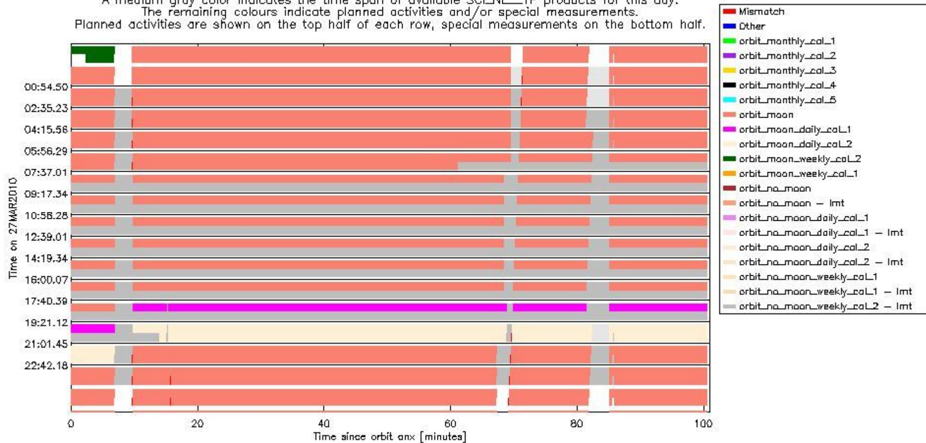
sciamachy_daily_report_level0_Any_version_20100327_6.PNG
