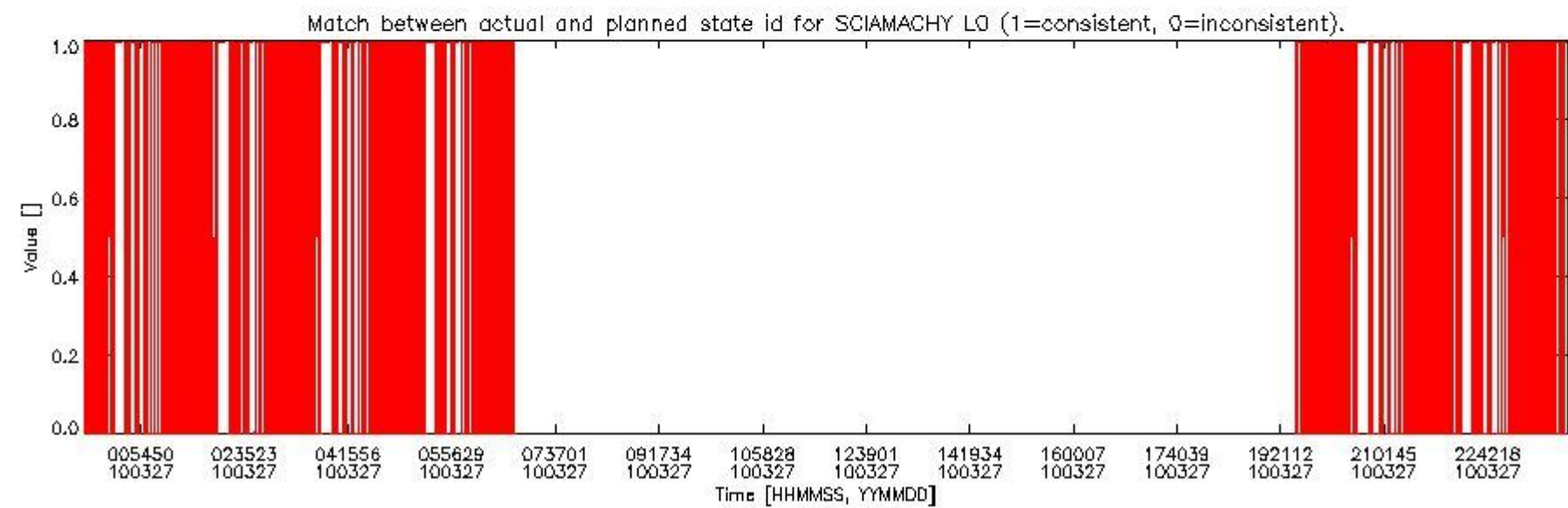
sciamachy_daily_report_level0_Any_version_20100327_5.PNG
