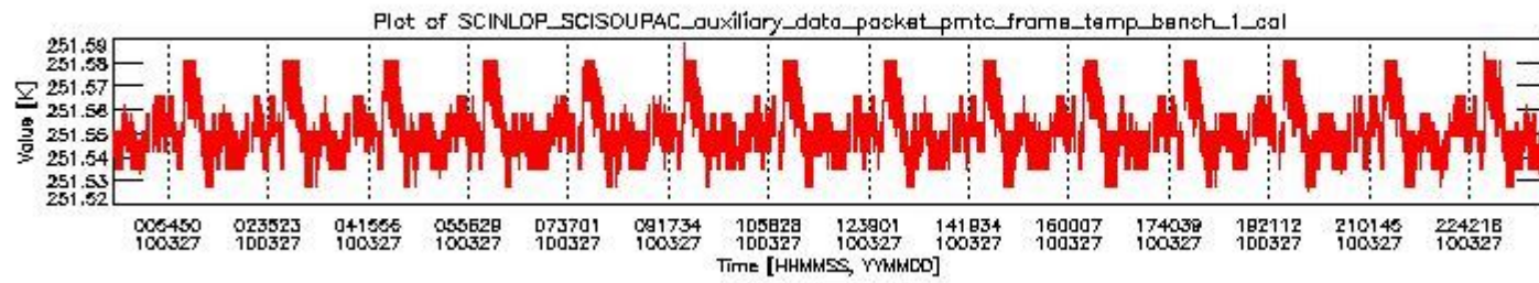
sciamachy_daily_report_level0_Any_version_20100327_0.PNG
