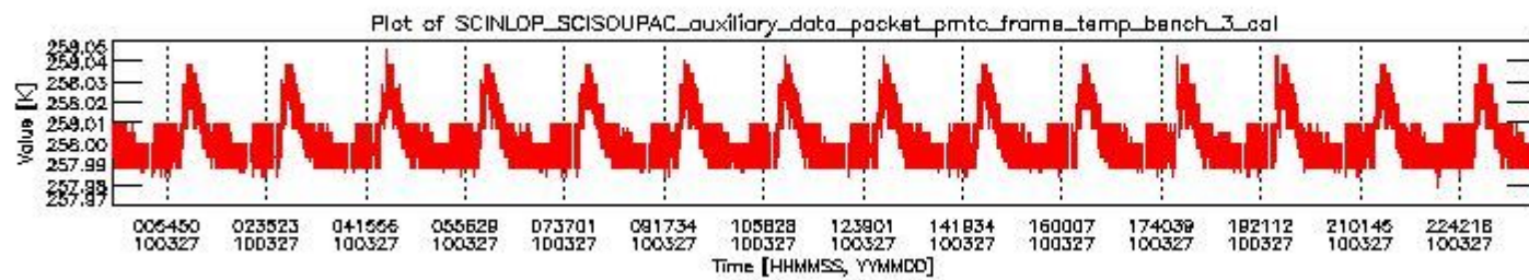
sciamachy_daily_report_level0_Any_version_20100327_2.PNG
