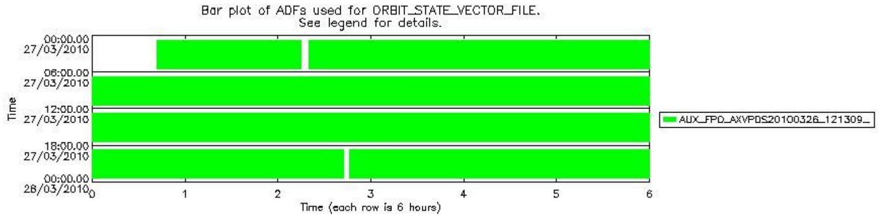
sciamachy_daily_report_level0_Any_version_20100327_8.PNG
