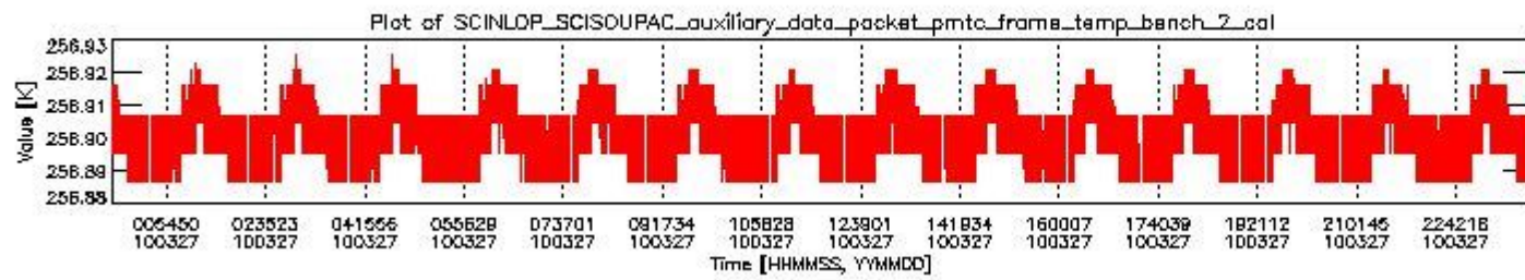
sciamachy_daily_report_level0_Any_version_20100327_1.PNG
