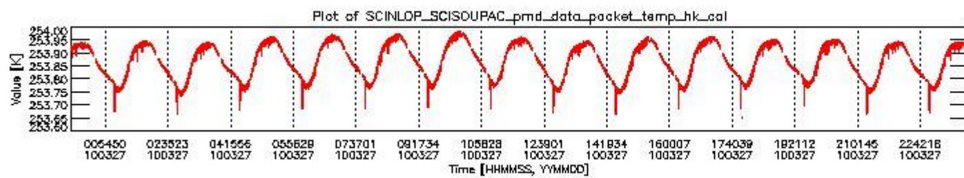
sciamachy_daily_report_level0_Any_version_20100327_3.PNG
