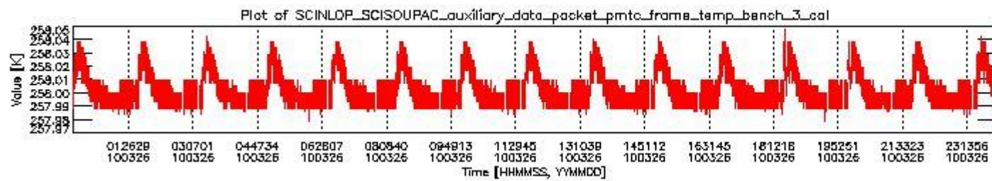
sciamachy_daily_report_level0_Any_version_20100326_2.PNG
