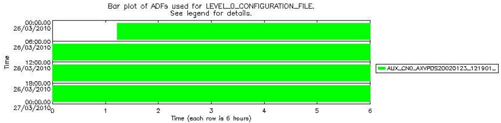
sciamachy_daily_report_level0_Any_version_20100326_7.PNG
