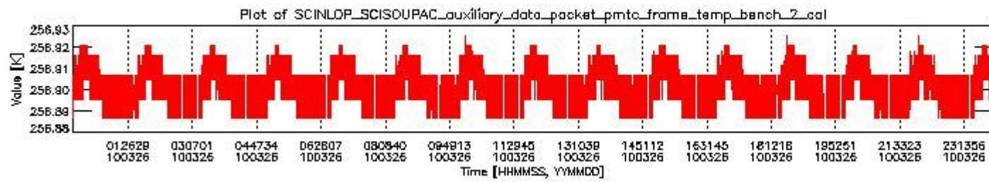
sciamachy_daily_report_level0_Any_version_20100326_1.PNG
