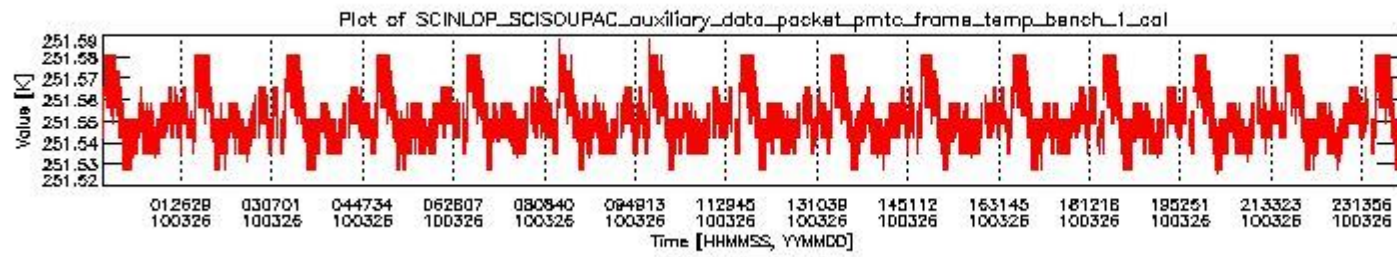
sciamachy_daily_report_level0_Any_version_20100326_0.PNG
