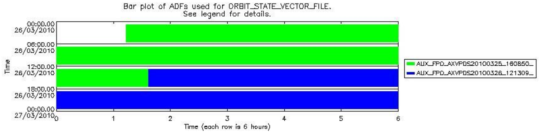
sciamachy_daily_report_level0_Any_version_20100326_8.PNG
