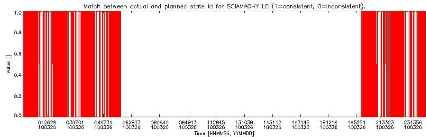
sciamachy_daily_report_level0_Any_version_20100326_5.PNG
