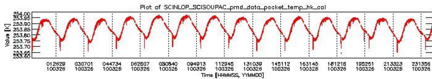
sciamachy_daily_report_level0_Any_version_20100326_3.PNG
