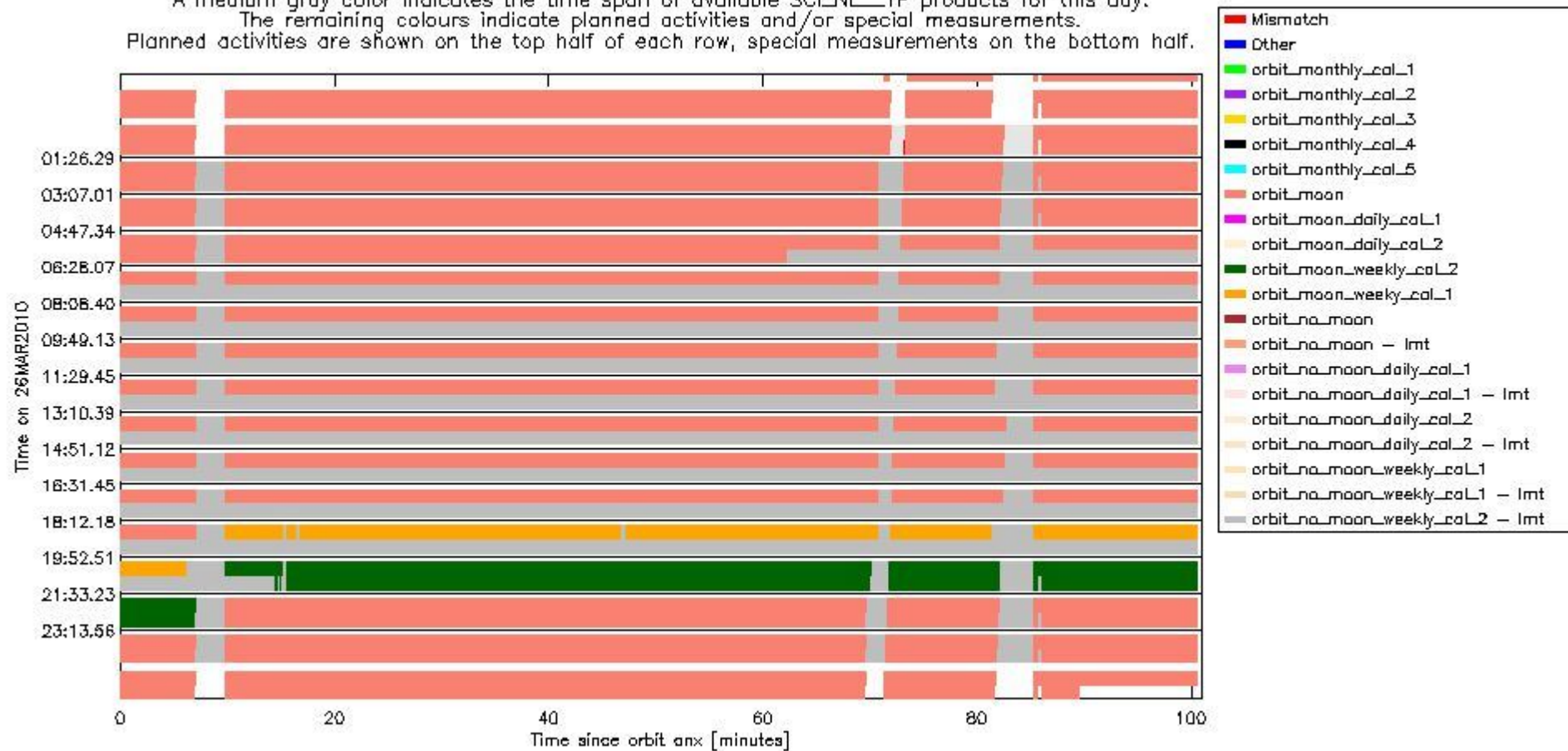
sciamachy_daily_report_level0_Any_version_20100326_6.PNG
