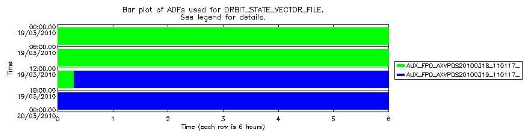
sciamachy_daily_report_level0_KSPT_L0_4303_N_20100319_8.PNG
