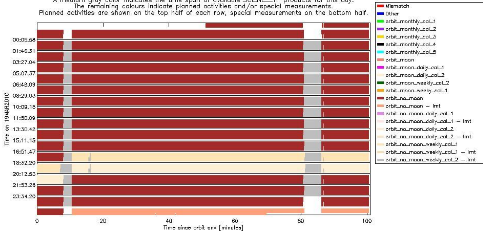
sciamachy_daily_report_level0_KSPT_L0_4303_N_20100319_6.PNG
