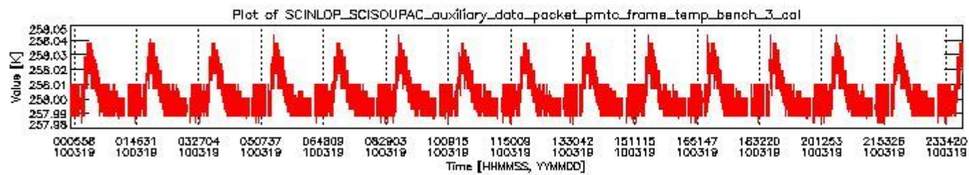
sciamachy_daily_report_level0_KSPT_L0_4303_N_20100319_2.PNG
