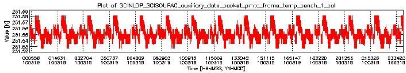
sciamachy_daily_report_level0_KSPT_L0_4303_N_20100319_0.PNG
