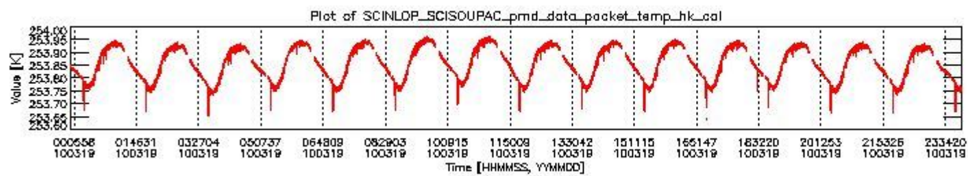
sciamachy_daily_report_level0_KSPT_L0_4303_N_20100319_3.PNG
