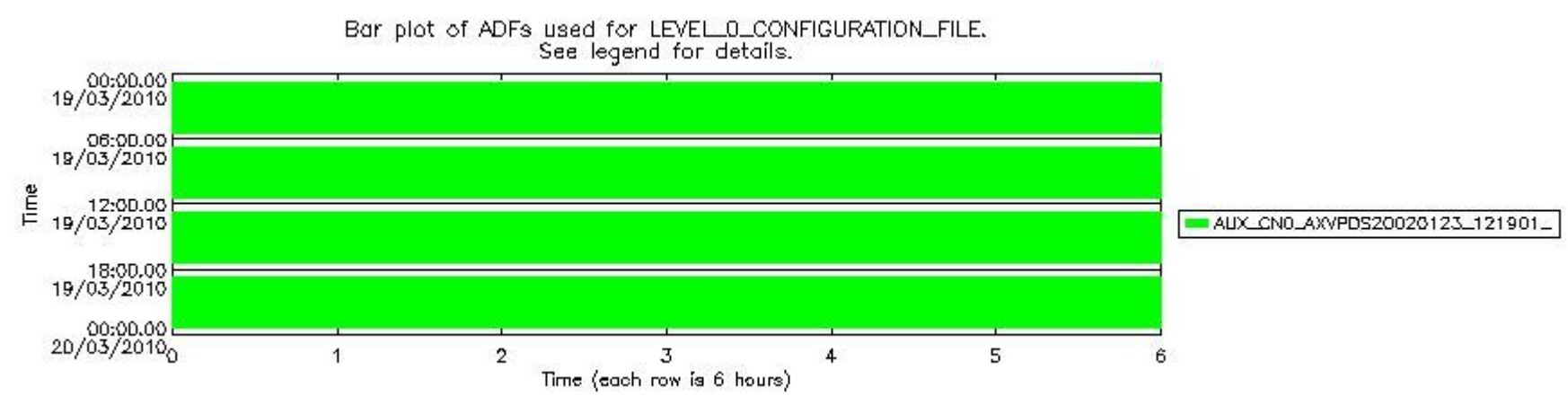
sciamachy_daily_report_level0_KSPT_L0_4303_N_20100319_7.PNG
