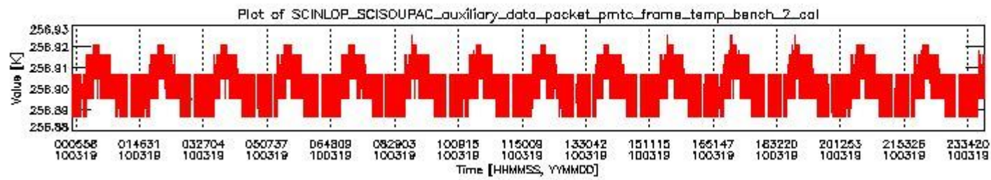
sciamachy_daily_report_level0_KSPT_L0_4303_N_20100319_1.PNG
