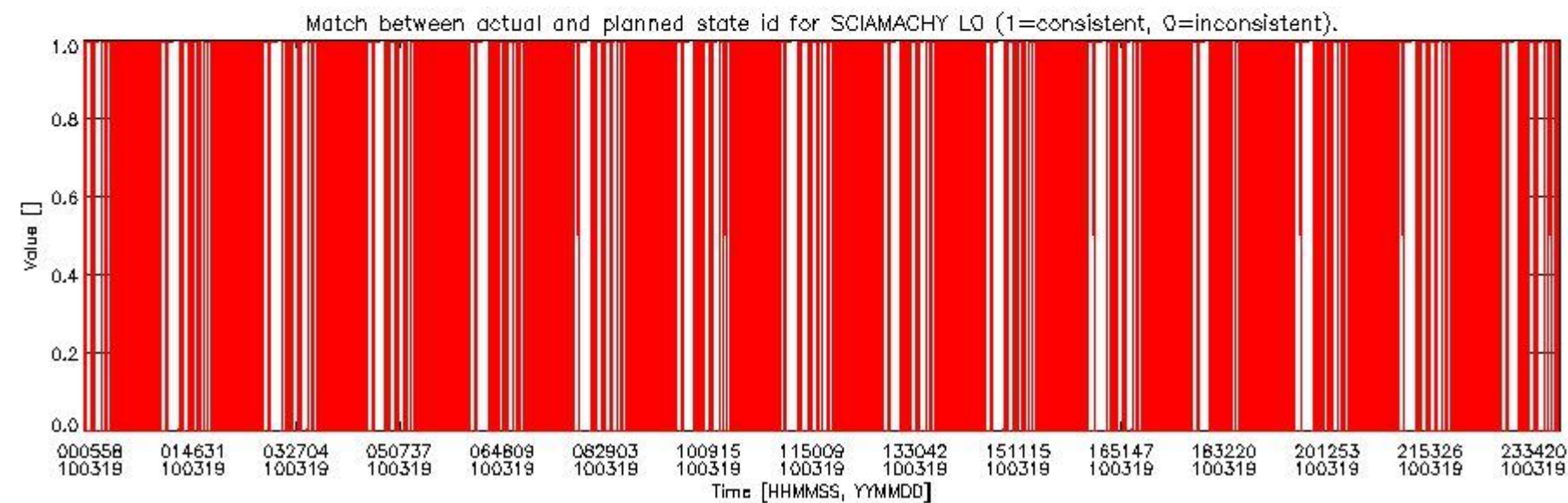
sciamachy_daily_report_level0_KSPT_L0_4303_N_20100319_5.PNG
