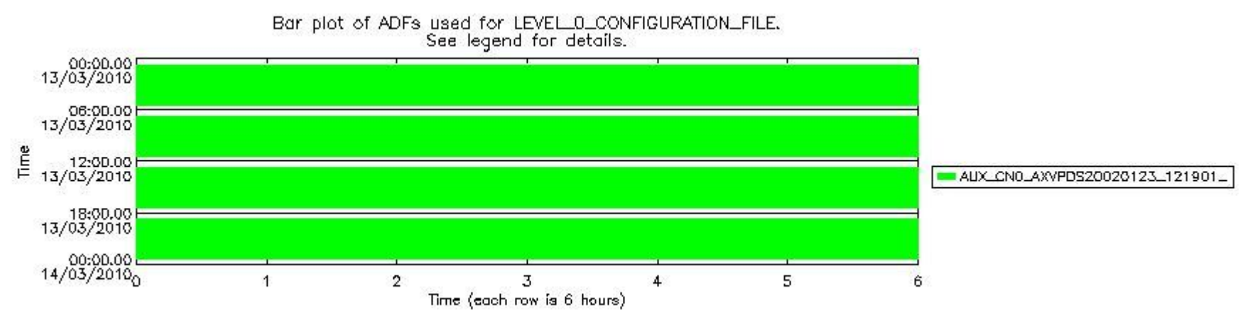
sciamachy_daily_report_level0_KSPT_L0_4303_N_20100313_7.PNG
