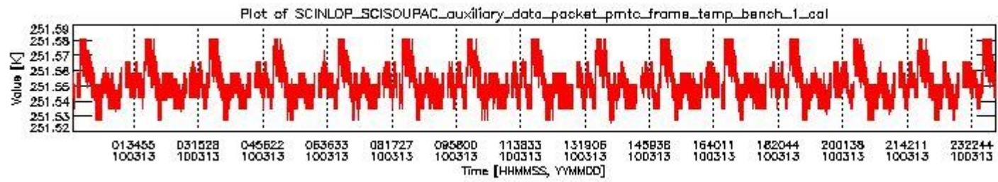
sciamachy_daily_report_level0_KSPT_L0_4303_N_20100313_0.PNG
