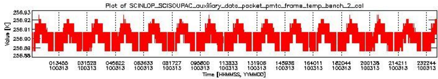
sciamachy_daily_report_level0_KSPT_L0_4303_N_20100313_1.PNG
