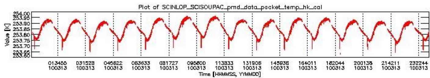
sciamachy_daily_report_level0_KSPT_L0_4303_N_20100313_3.PNG
