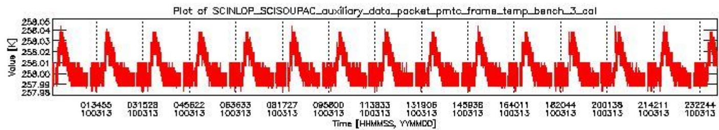
sciamachy_daily_report_level0_KSPT_L0_4303_N_20100313_2.PNG
