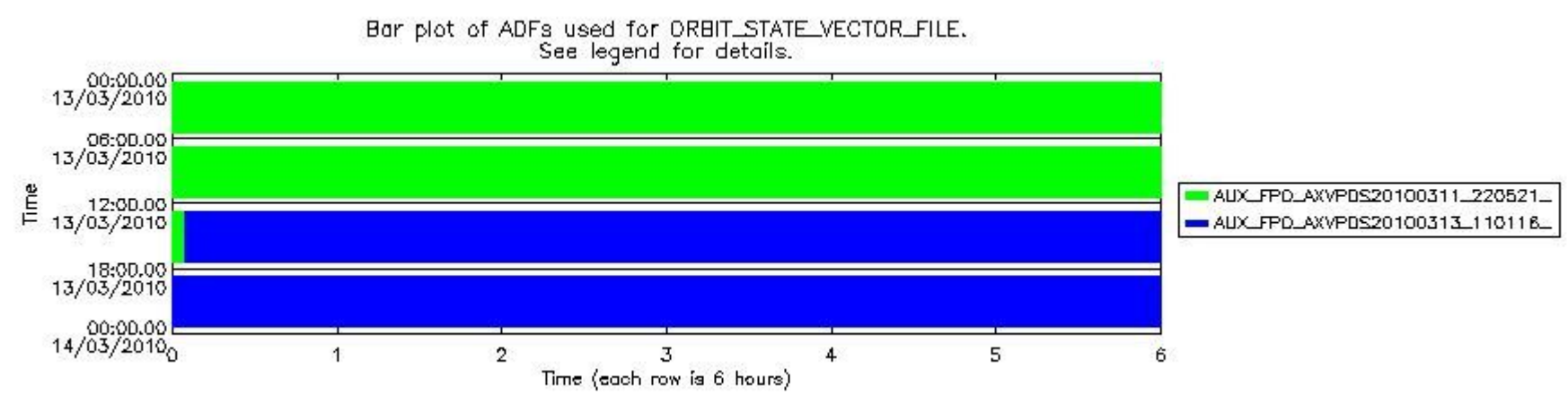
sciamachy_daily_report_level0_KSPT_L0_4303_N_20100313_8.PNG
