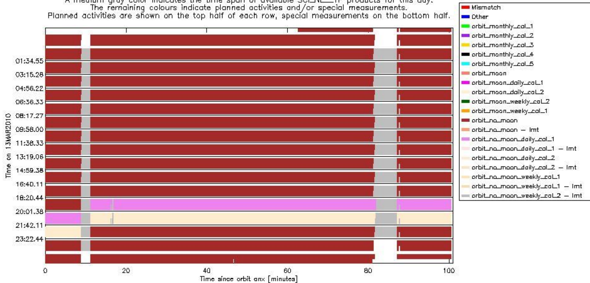
sciamachy_daily_report_level0_KSPT_L0_4303_N_20100313_6.PNG
