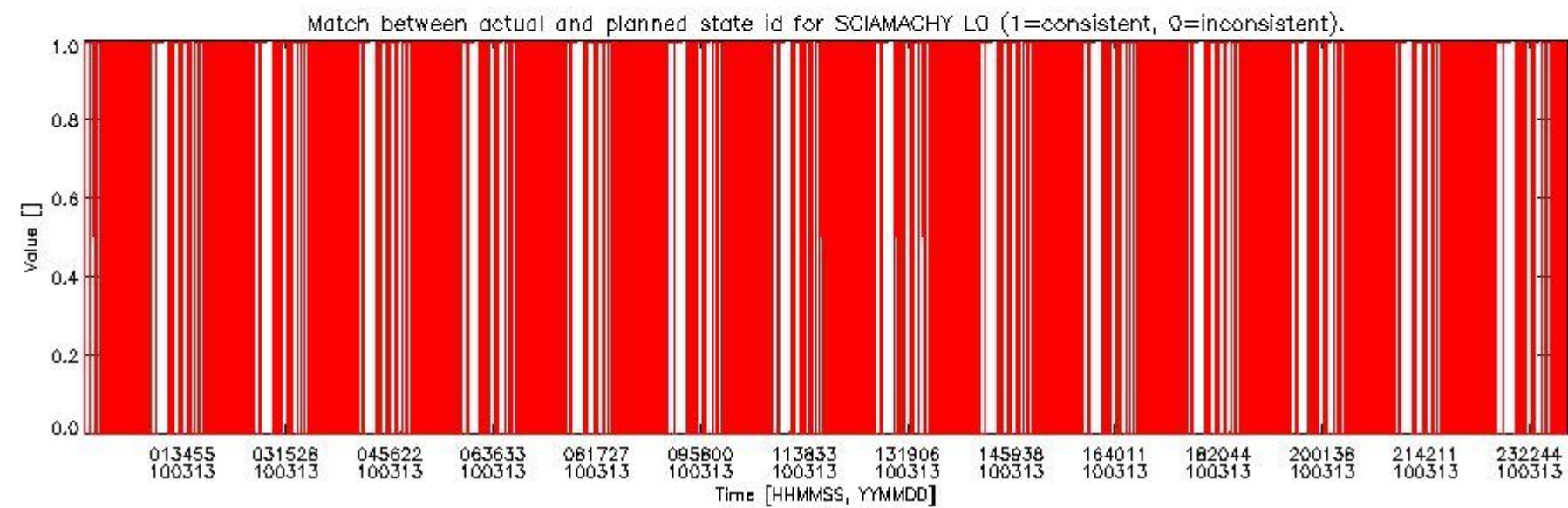
sciamachy_daily_report_level0_KSPT_L0_4303_N_20100313_5.PNG
