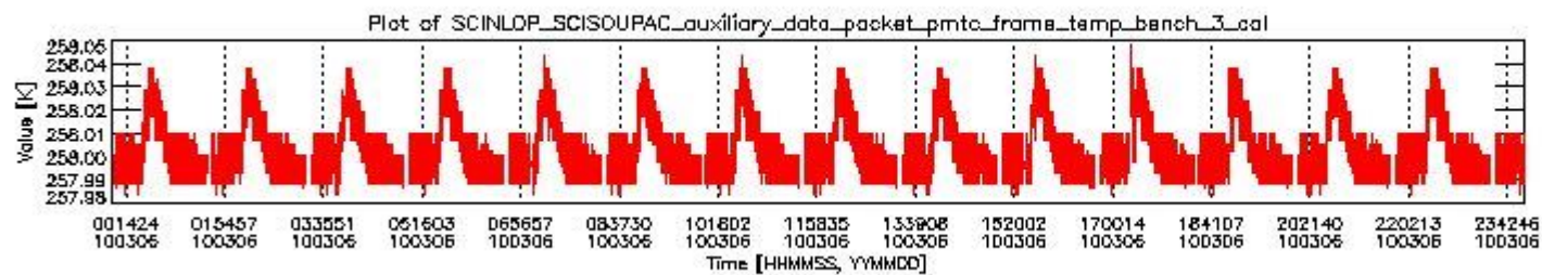
sciamachy_daily_report_level0_Any_version_20100306_2.PNG
