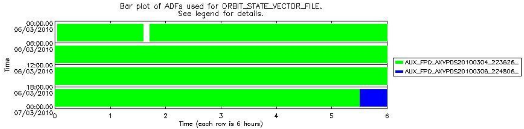
sciamachy_daily_report_level0_Any_version_20100306_8.PNG
