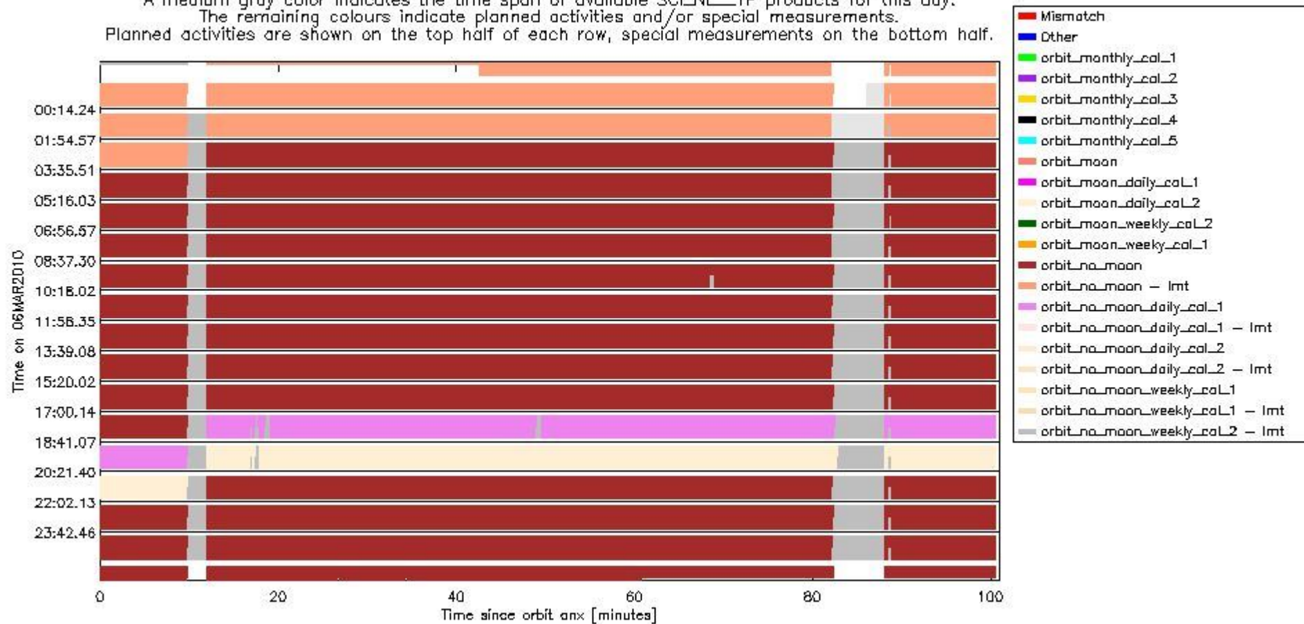
sciamachy_daily_report_level0_Any_version_20100306_6.PNG
