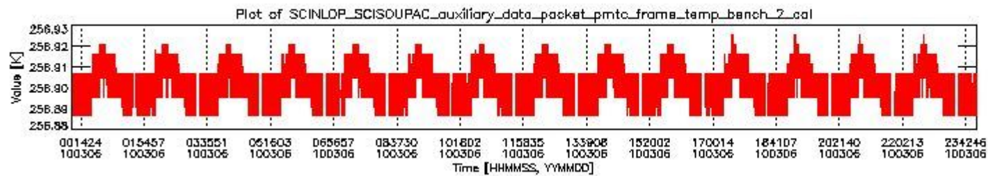
sciamachy_daily_report_level0_Any_version_20100306_1.PNG
