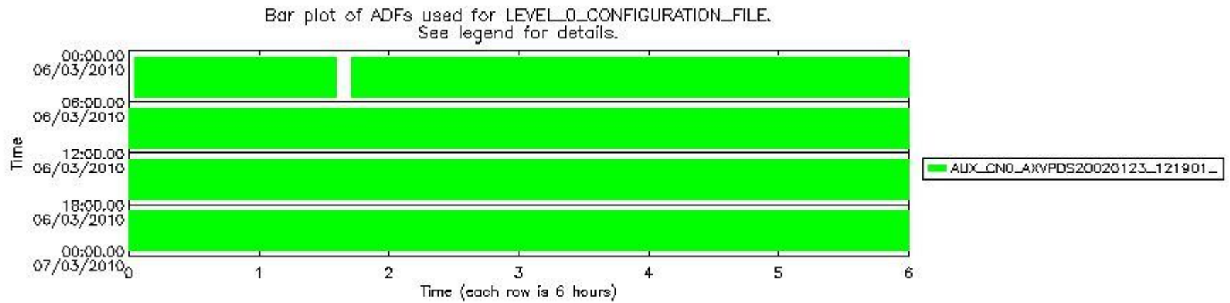
sciamachy_daily_report_level0_Any_version_20100306_7.PNG
