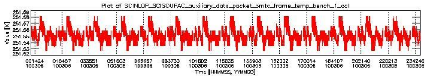
sciamachy_daily_report_level0_Any_version_20100306_0.PNG
