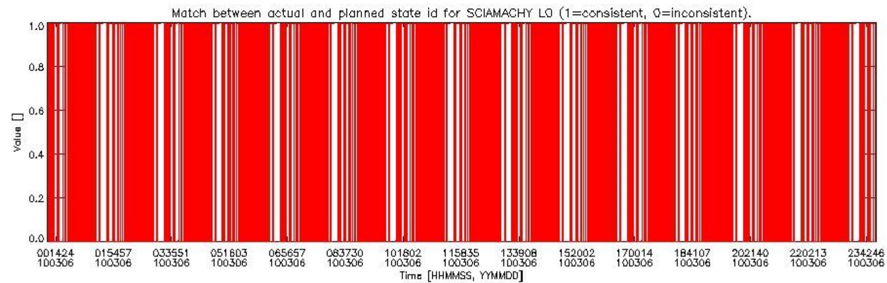
sciamachy_daily_report_level0_Any_version_20100306_5.PNG
