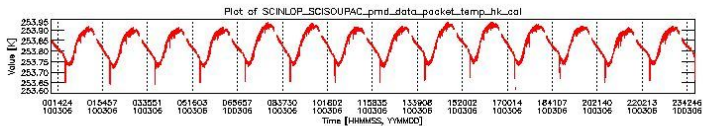
sciamachy_daily_report_level0_Any_version_20100306_3.PNG
