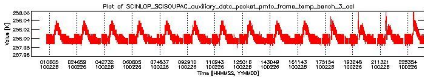
sciamachy_daily_report_level0_KSPT_L0_4303_N_20100226_2.PNG
