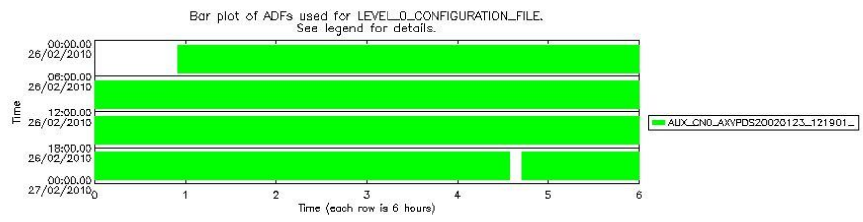
sciamachy_daily_report_level0_KSPT_L0_4303_N_20100226_6.PNG
