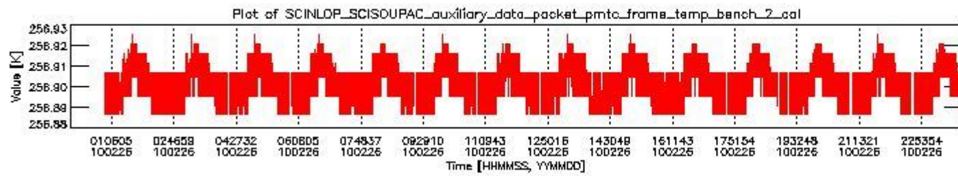
sciamachy_daily_report_level0_KSPT_L0_4303_N_20100226_1.PNG
