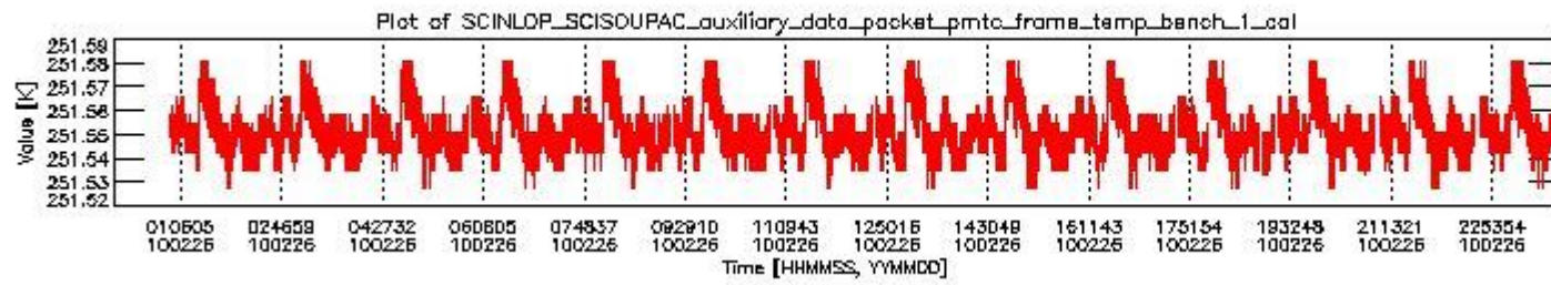
sciamachy_daily_report_level0_KSPT_L0_4303_N_20100226_0.PNG
