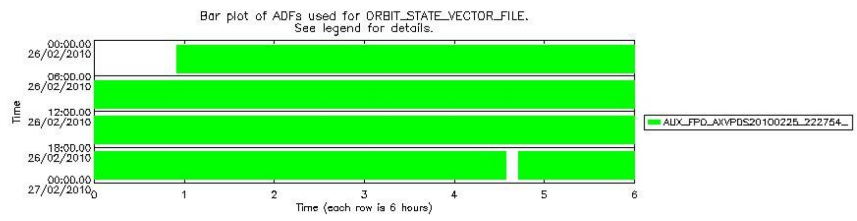
sciamachy_daily_report_level0_KSPT_L0_4303_N_20100226_7.PNG
