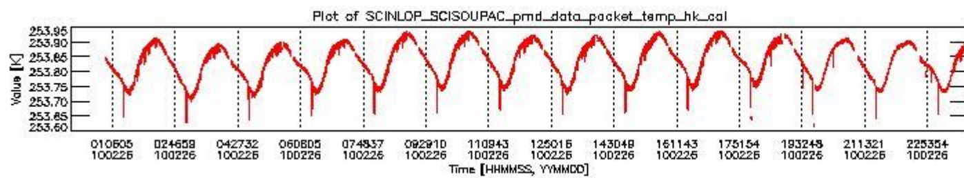
sciamachy_daily_report_level0_KSPT_L0_4303_N_20100226_3.PNG
