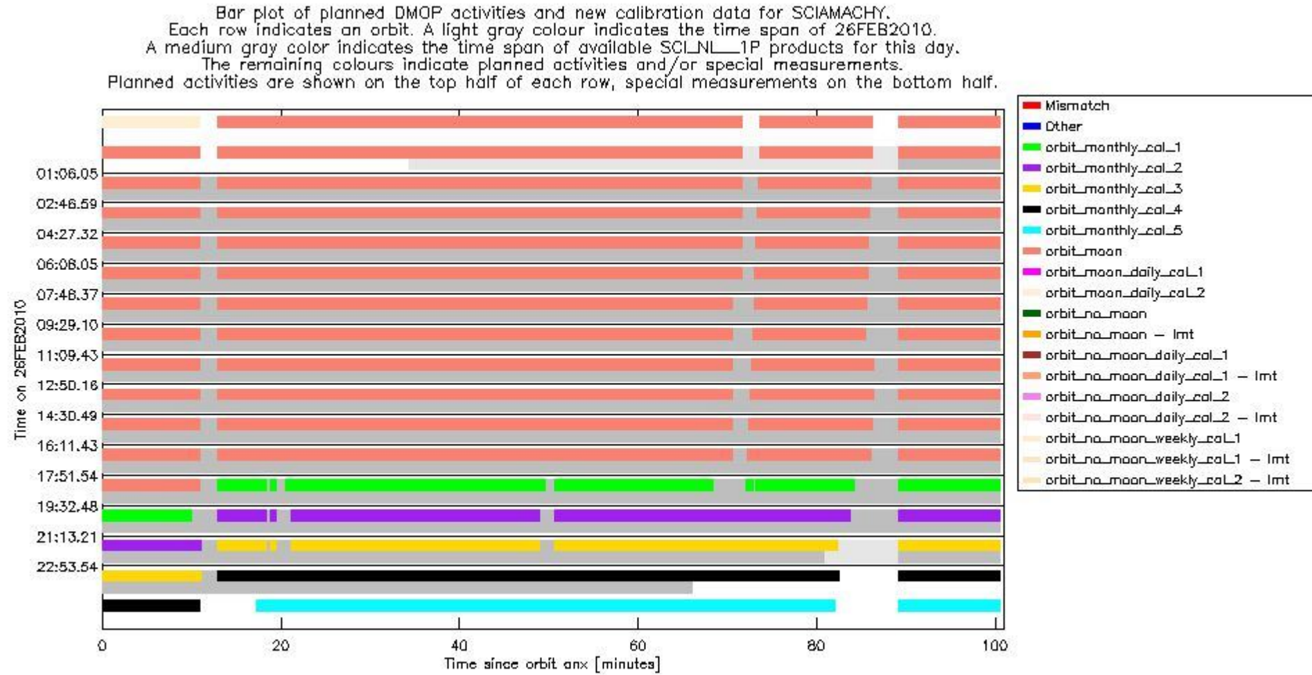
sciamachy_daily_report_level0_KSPT_L0_4303_N_20100226_5.PNG
