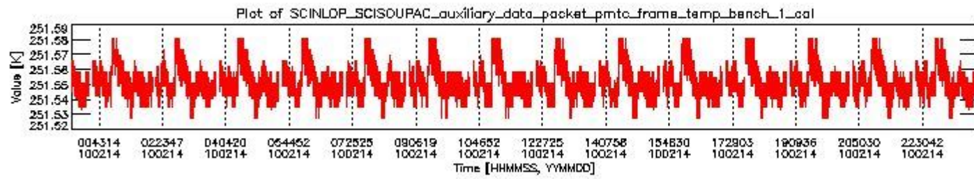
sciamachy_daily_report_level0_KSPT_L0_4303_N_20100214_0.PNG
