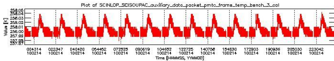
sciamachy_daily_report_level0_KSPT_L0_4303_N_20100214_2.PNG
