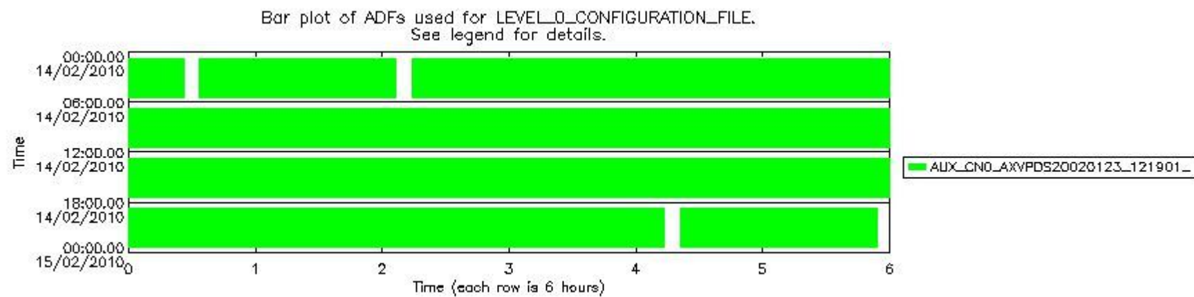
sciamachy_daily_report_level0_KSPT_L0_4303_N_20100214_6.PNG
