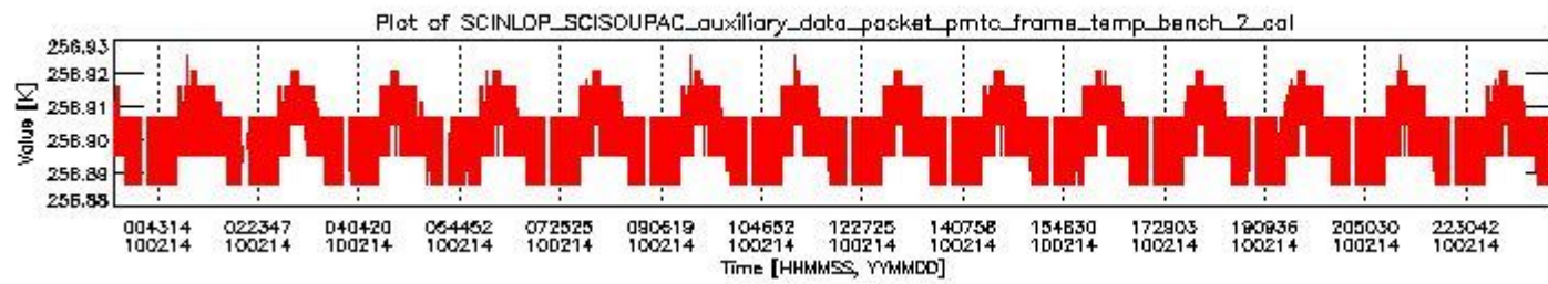
sciamachy_daily_report_level0_KSPT_L0_4303_N_20100214_1.PNG
