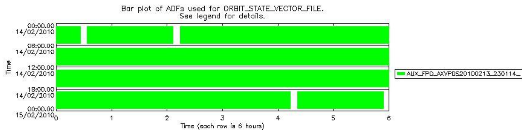
sciamachy_daily_report_level0_KSPT_L0_4303_N_20100214_7.PNG
