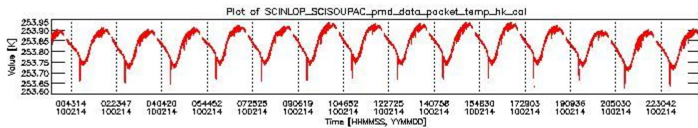
sciamachy_daily_report_level0_KSPT_L0_4303_N_20100214_3.PNG
