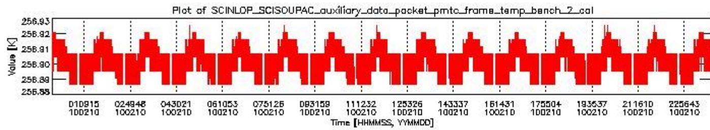
sciamachy_daily_report_level0_KSPT_L0_4303_N_20100210_1.PNG
