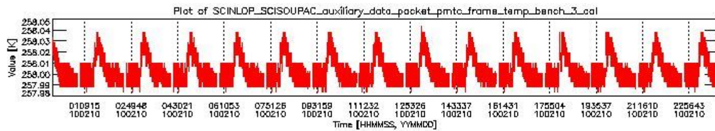
sciamachy_daily_report_level0_KSPT_L0_4303_N_20100210_2.PNG
