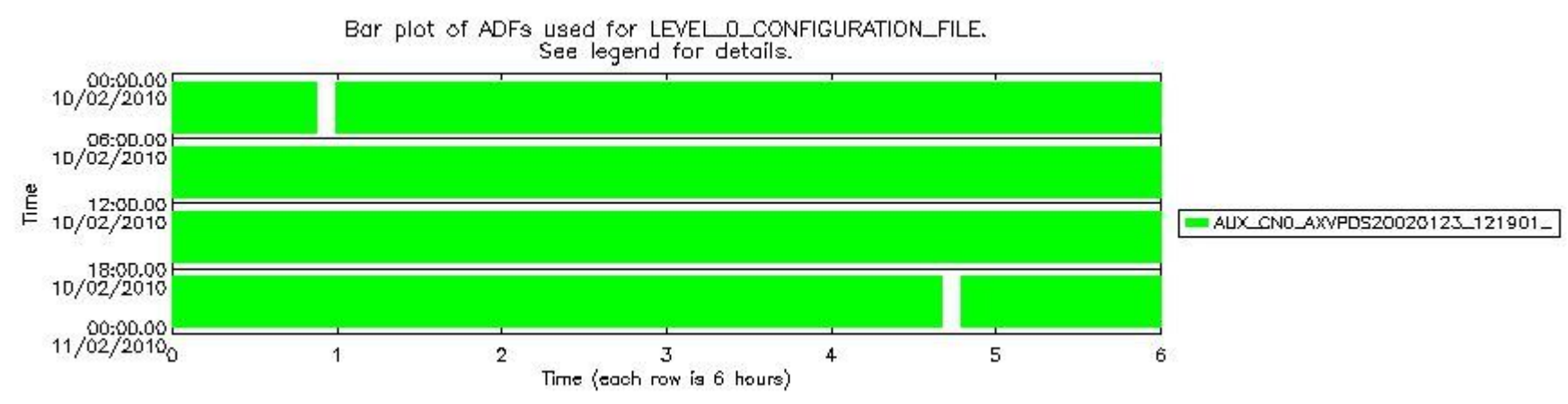
sciamachy_daily_report_level0_KSPT_L0_4303_N_20100210_6.PNG
