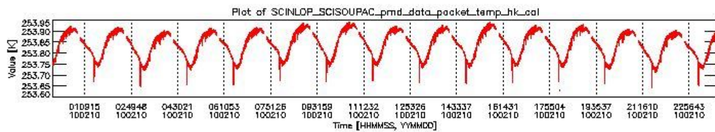
sciamachy_daily_report_level0_KSPT_L0_4303_N_20100210_3.PNG
