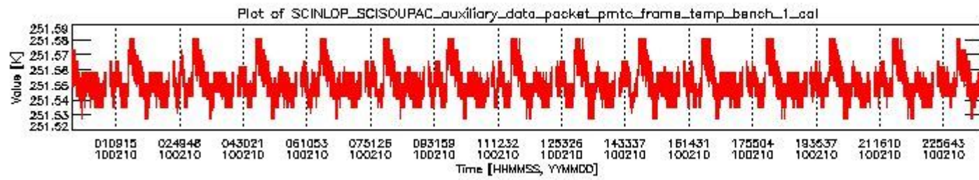
sciamachy_daily_report_level0_KSPT_L0_4303_N_20100210_0.PNG
