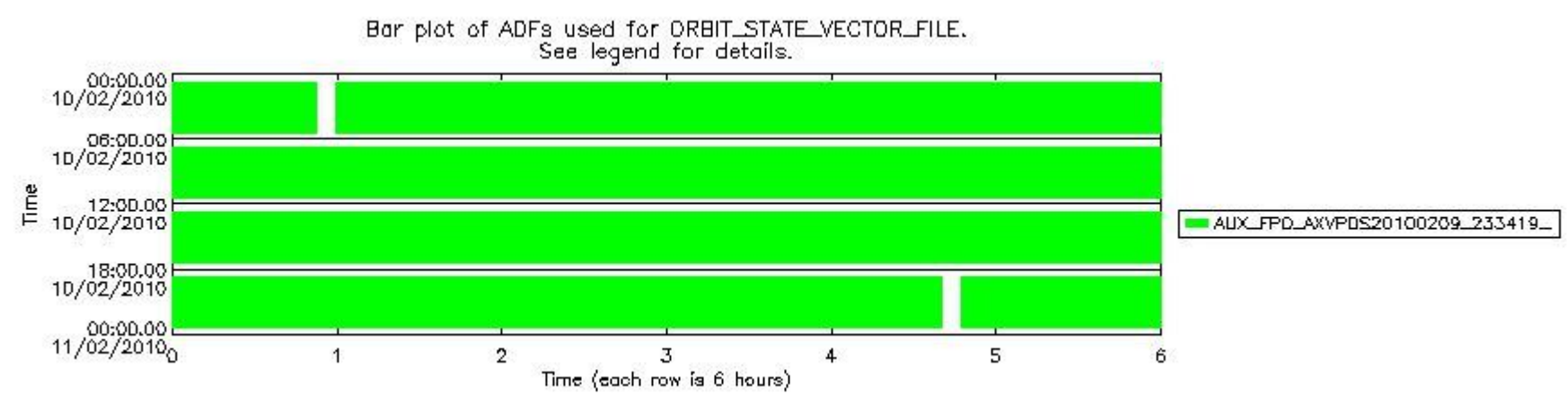
sciamachy_daily_report_level0_KSPT_L0_4303_N_20100210_7.PNG
