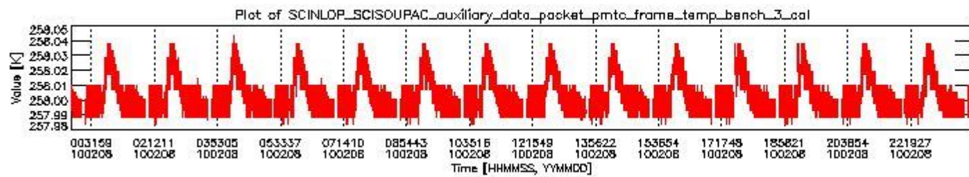
sciamachy_daily_report_level0_KSPT_L0_4303_N_20100208_2.PNG
