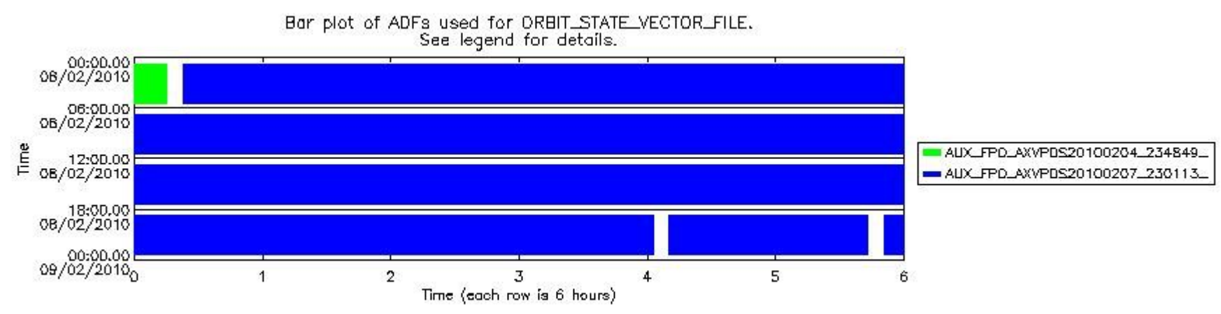
sciamachy_daily_report_level0_KSPT_L0_4303_N_20100208_7.PNG
