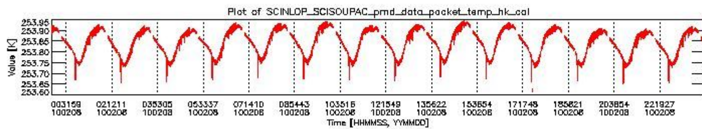
sciamachy_daily_report_level0_KSPT_L0_4303_N_20100208_3.PNG
