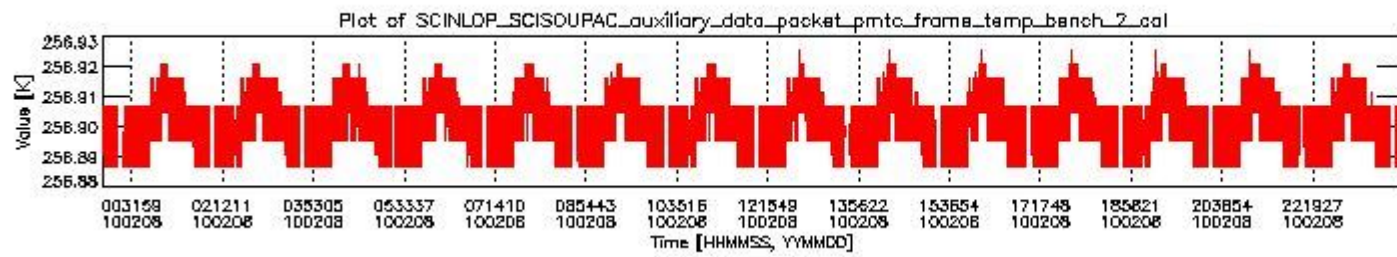
sciamachy_daily_report_level0_KSPT_L0_4303_N_20100208_1.PNG
