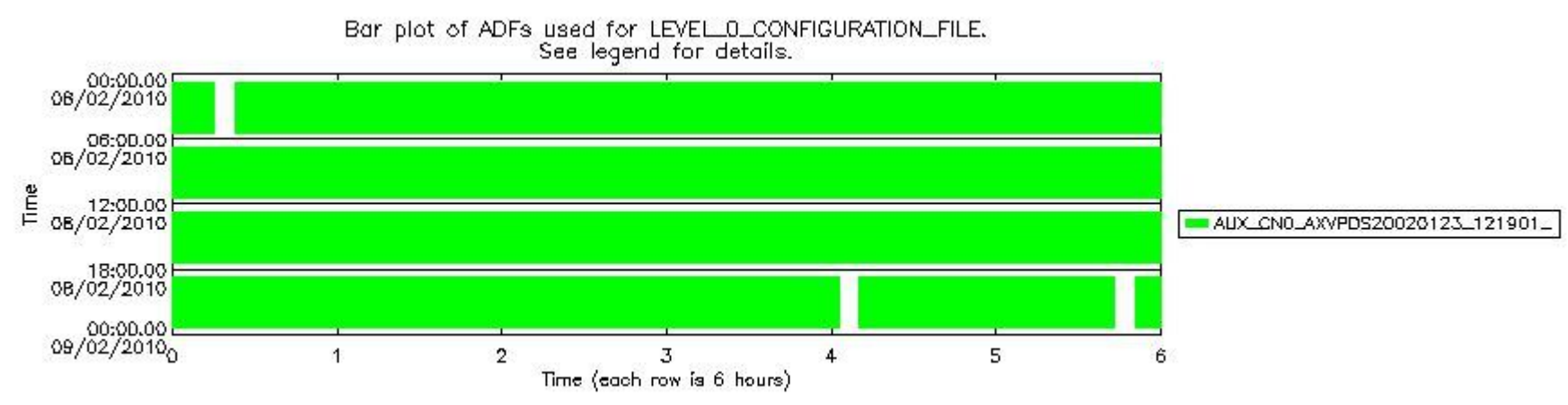
sciamachy_daily_report_level0_KSPT_L0_4303_N_20100208_6.PNG
