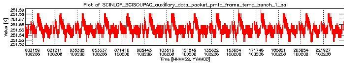
sciamachy_daily_report_level0_KSPT_L0_4303_N_20100208_0.PNG
