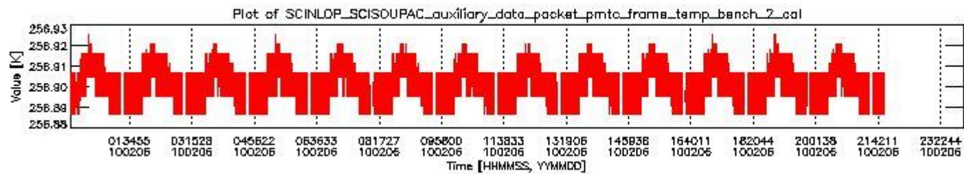
sciamachy_daily_report_level0_KSPT_L0_4303_N_20100206_1.PNG
