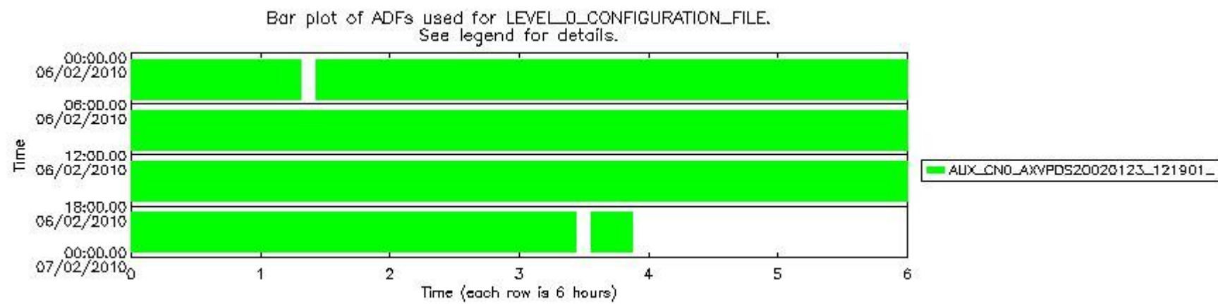
sciamachy_daily_report_level0_KSPT_L0_4303_N_20100206_6.PNG
