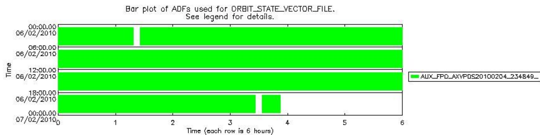
sciamachy_daily_report_level0_KSPT_L0_4303_N_20100206_7.PNG
