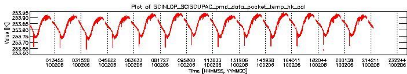
sciamachy_daily_report_level0_KSPT_L0_4303_N_20100206_3.PNG
