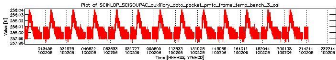
sciamachy_daily_report_level0_KSPT_L0_4303_N_20100206_2.PNG
