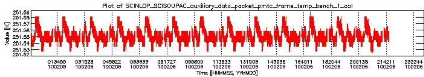
sciamachy_daily_report_level0_KSPT_L0_4303_N_20100206_0.PNG
