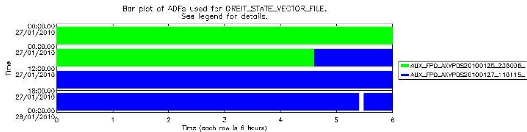
sciamachy_daily_report_level0_KSPT_L0_4303_N_20100127_7.PNG
