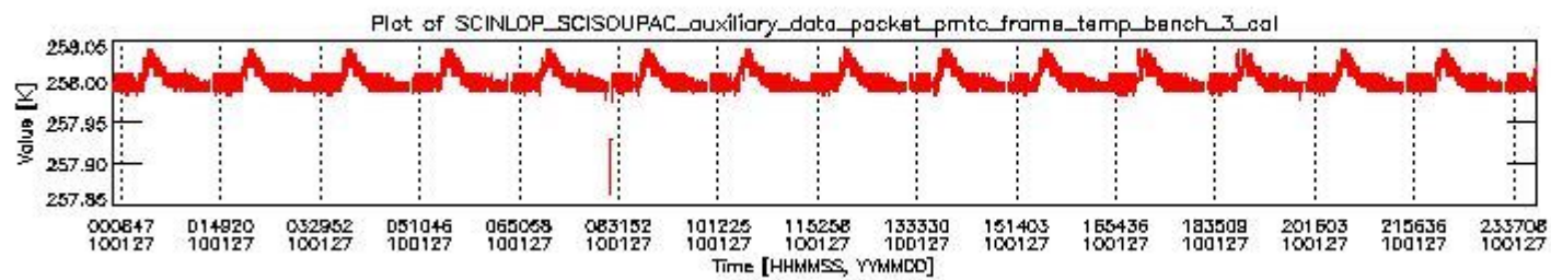
sciamachy_daily_report_level0_KSPT_L0_4303_N_20100127_2.PNG
