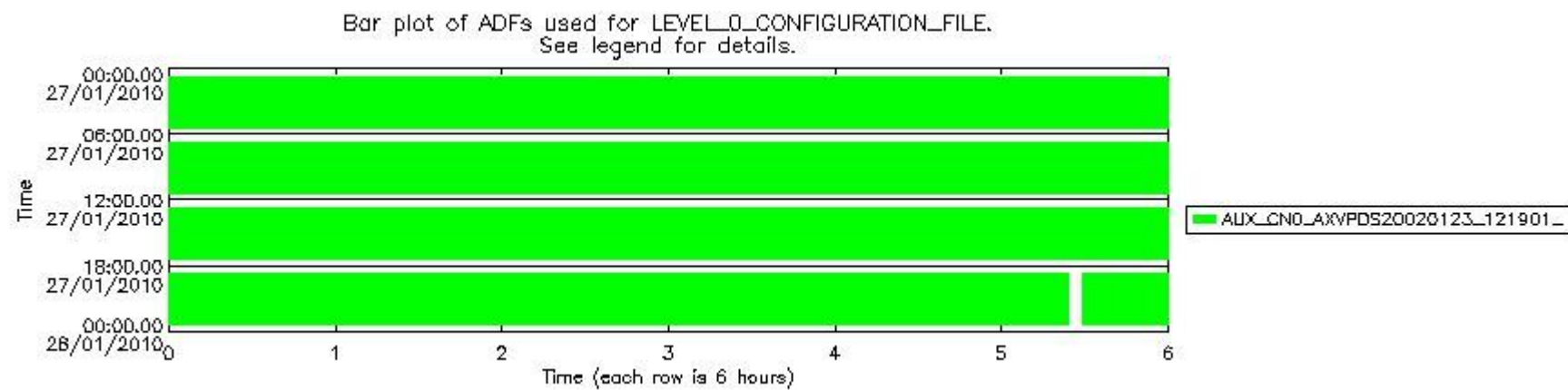
sciamachy_daily_report_level0_KSPT_L0_4303_N_20100127_6.PNG
