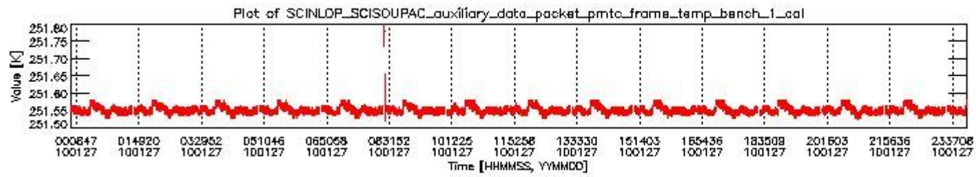
sciamachy_daily_report_level0_KSPT_L0_4303_N_20100127_0.PNG
