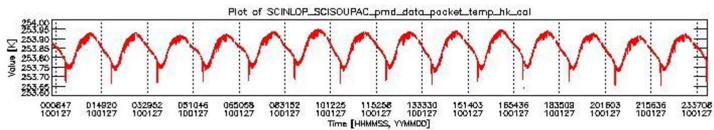
sciamachy_daily_report_level0_KSPT_L0_4303_N_20100127_3.PNG
