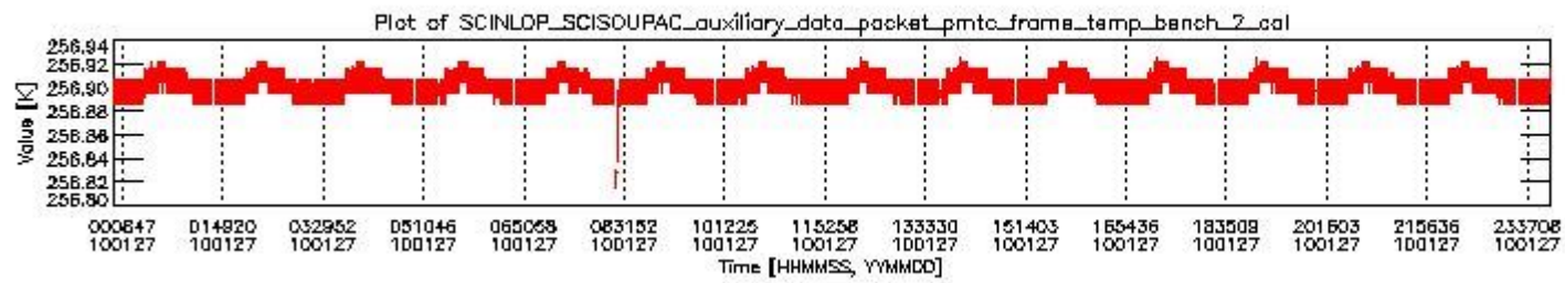
sciamachy_daily_report_level0_KSPT_L0_4303_N_20100127_1.PNG
