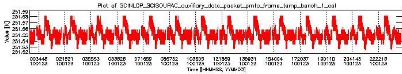
sciamachy_daily_report_level0_KSPT_L0_4303_N_20100123_0.PNG
