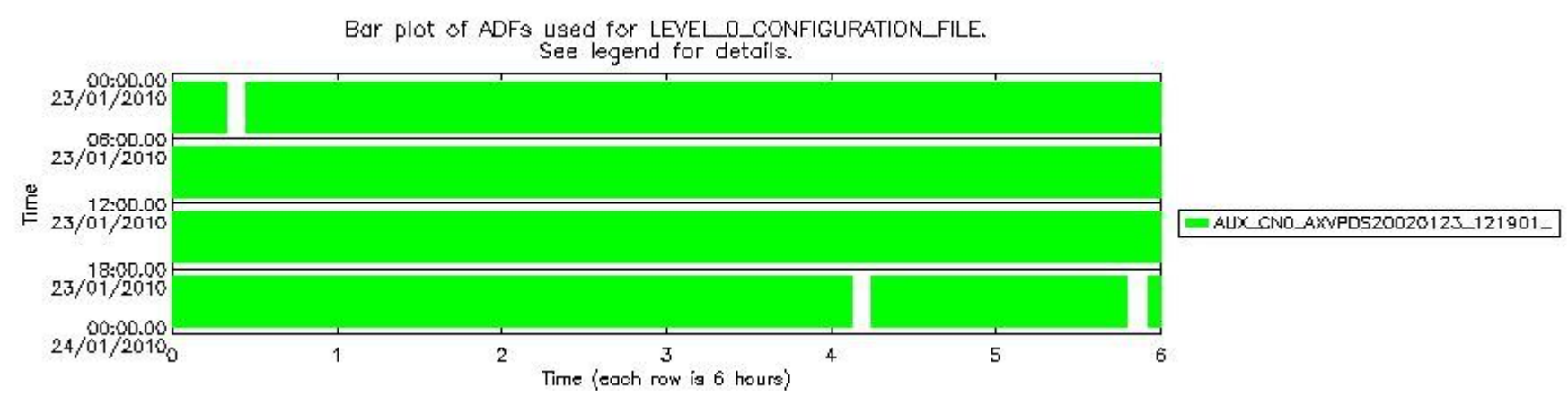
sciamachy_daily_report_level0_KSPT_L0_4303_N_20100123_6.PNG
