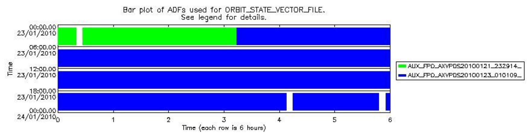
sciamachy_daily_report_level0_KSPT_L0_4303_N_20100123_7.PNG
