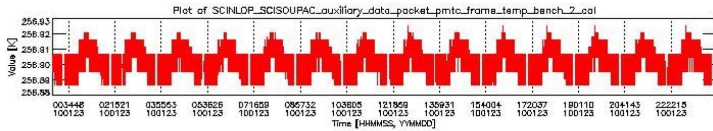
sciamachy_daily_report_level0_KSPT_L0_4303_N_20100123_1.PNG
