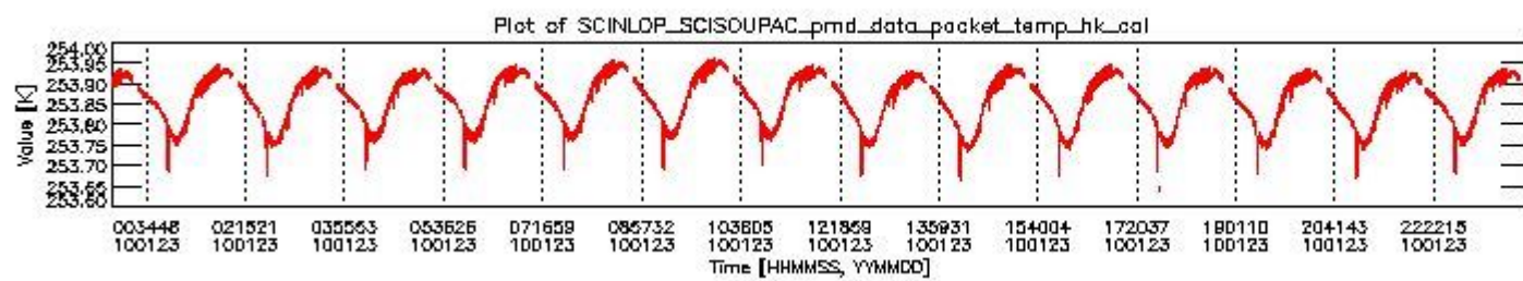
sciamachy_daily_report_level0_KSPT_L0_4303_N_20100123_3.PNG
