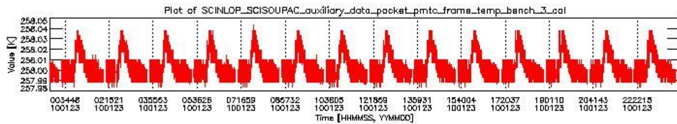
sciamachy_daily_report_level0_KSPT_L0_4303_N_20100123_2.PNG
