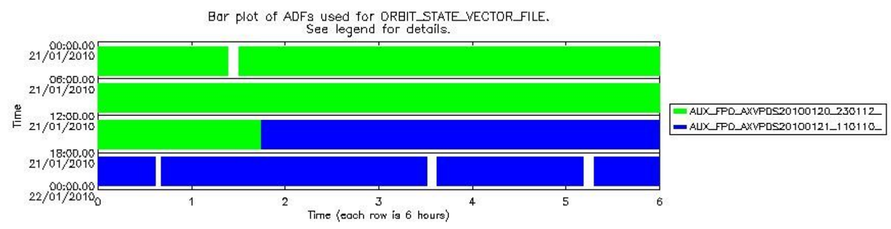
sciamachy_daily_report_level0_KSPT_L0_4303_N_20100121_7.PNG
