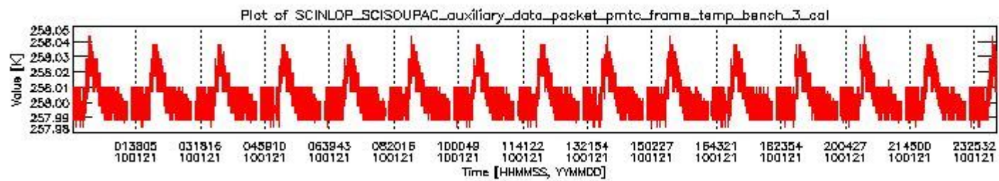
sciamachy_daily_report_level0_KSPT_L0_4303_N_20100121_2.PNG
