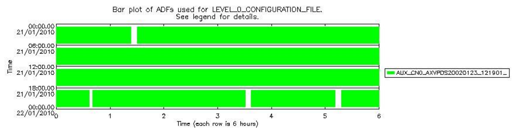
sciamachy_daily_report_level0_KSPT_L0_4303_N_20100121_6.PNG
