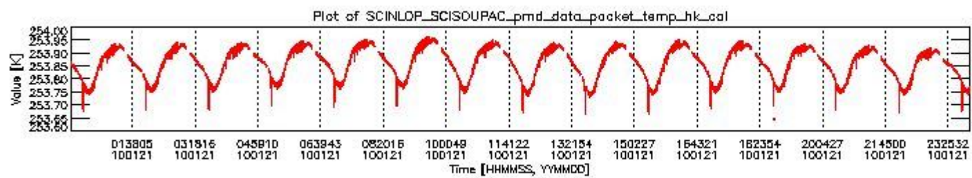
sciamachy_daily_report_level0_KSPT_L0_4303_N_20100121_3.PNG
