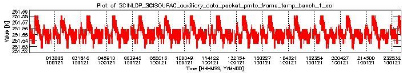
sciamachy_daily_report_level0_KSPT_L0_4303_N_20100121_0.PNG
