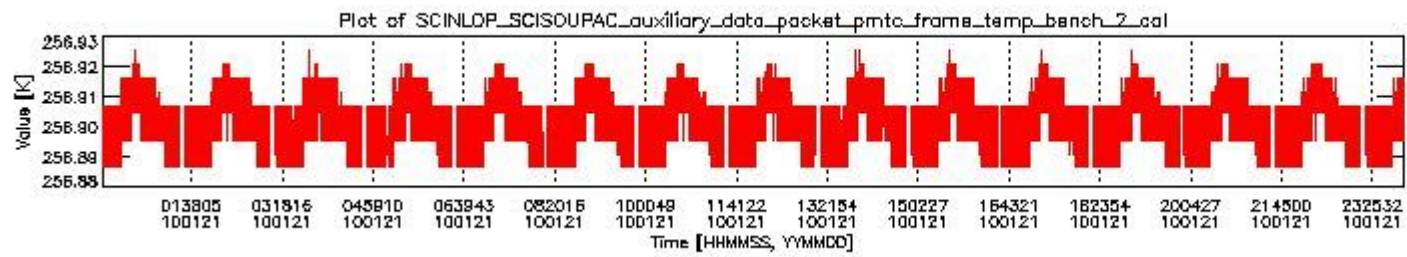
sciamachy_daily_report_level0_KSPT_L0_4303_N_20100121_1.PNG
