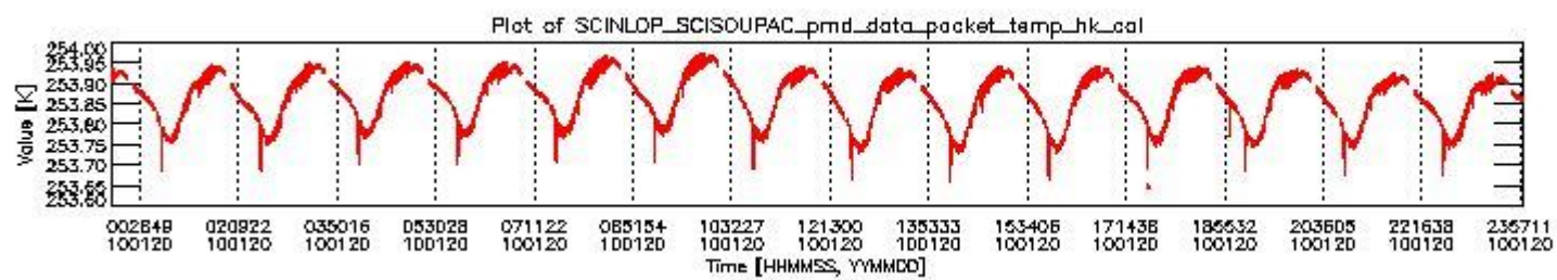
sciamachy_daily_report_level0_KSPT_L0_4303_N_20100120_3.PNG
