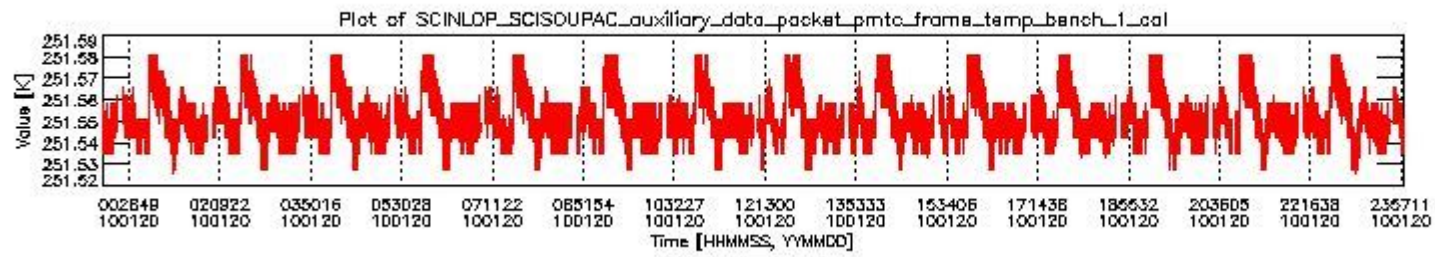
sciamachy_daily_report_level0_KSPT_L0_4303_N_20100120_0.PNG
