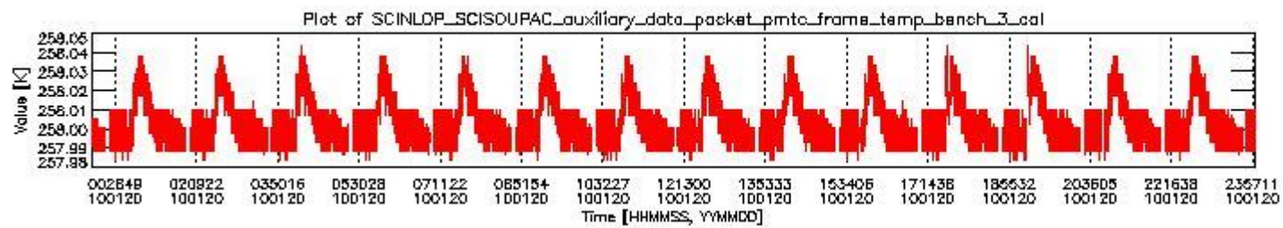
sciamachy_daily_report_level0_KSPT_L0_4303_N_20100120_2.PNG
