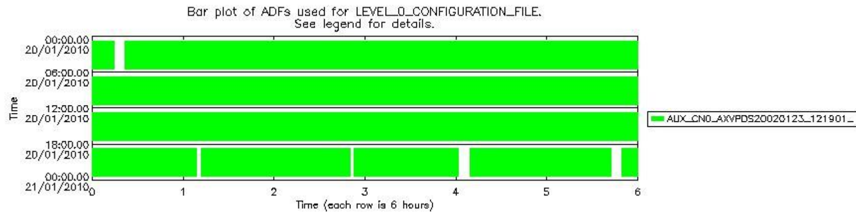
sciamachy_daily_report_level0_KSPT_L0_4303_N_20100120_6.PNG
