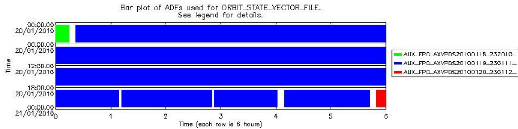
sciamachy_daily_report_level0_KSPT_L0_4303_N_20100120_7.PNG
