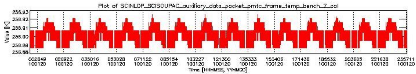
sciamachy_daily_report_level0_KSPT_L0_4303_N_20100120_1.PNG
