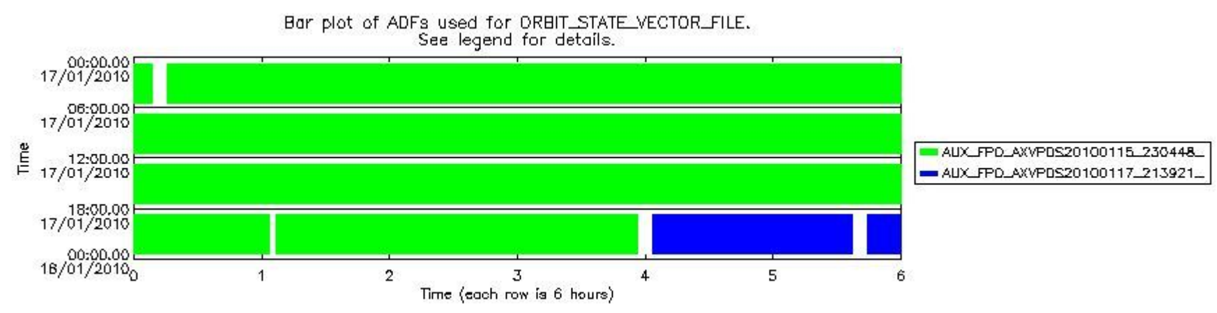
sciamachy_daily_report_level0_KSPT_L0_4303_N_20100117_7.PNG
