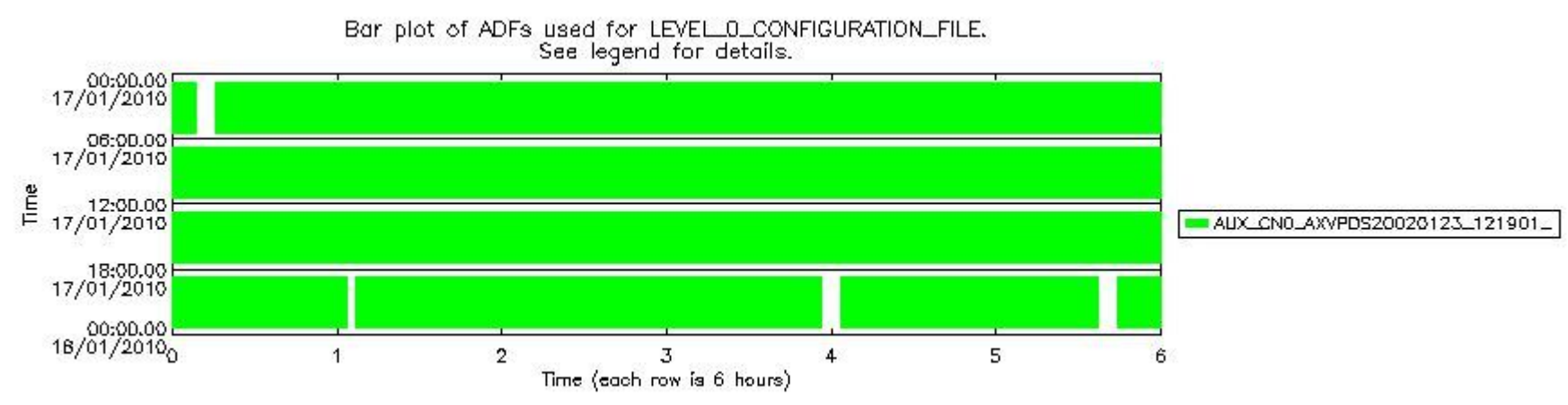
sciamachy_daily_report_level0_KSPT_L0_4303_N_20100117_6.PNG
