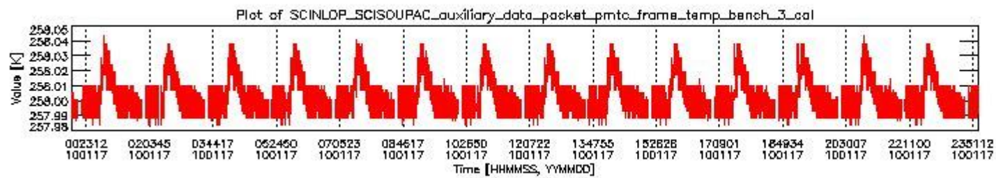
sciamachy_daily_report_level0_KSPT_L0_4303_N_20100117_2.PNG
