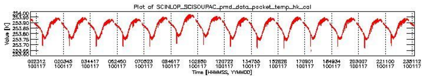
sciamachy_daily_report_level0_KSPT_L0_4303_N_20100117_3.PNG
