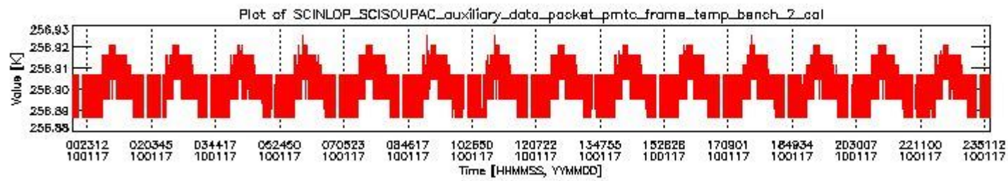
sciamachy_daily_report_level0_KSPT_L0_4303_N_20100117_1.PNG
