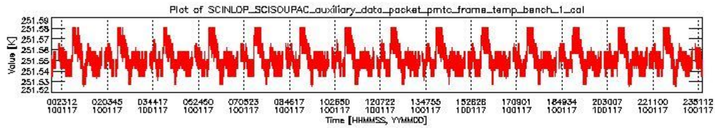
sciamachy_daily_report_level0_KSPT_L0_4303_N_20100117_0.PNG
