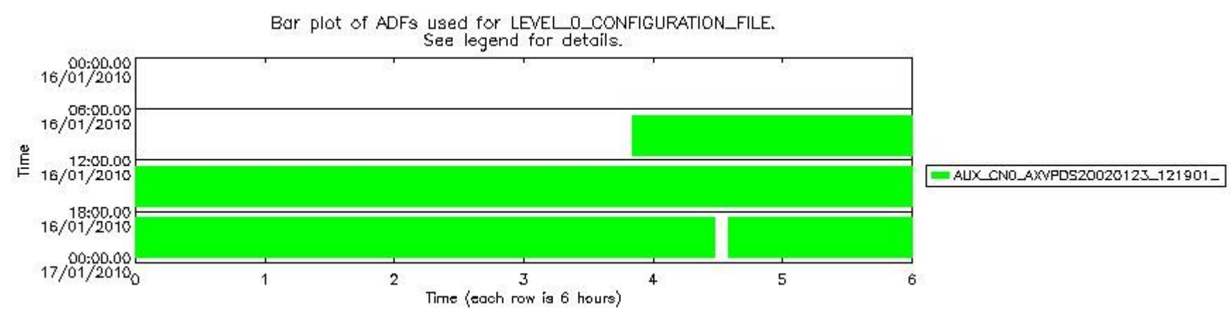
sciamachy_daily_report_level0_KSPT_L0_4303_N_20100116_6.PNG
