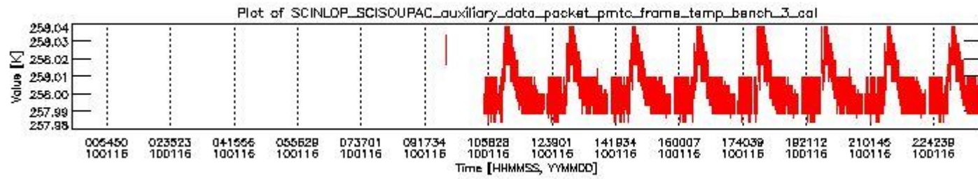
sciamachy_daily_report_level0_KSPT_L0_4303_N_20100116_2.PNG
