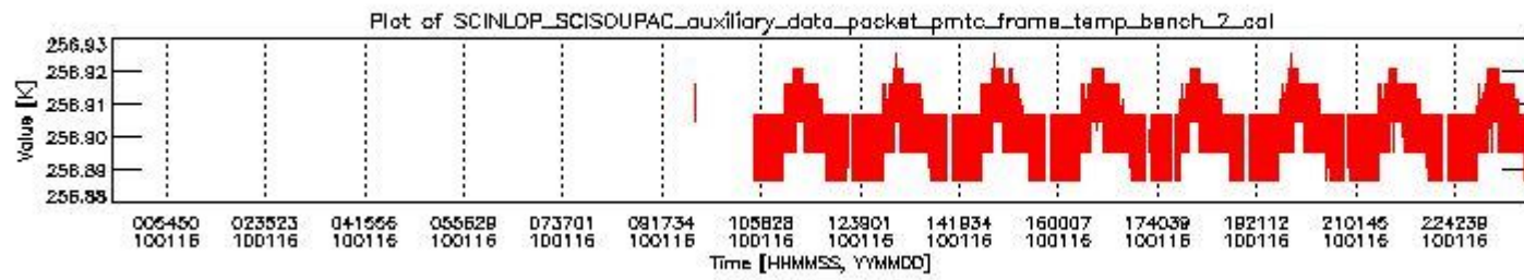
sciamachy_daily_report_level0_KSPT_L0_4303_N_20100116_1.PNG
