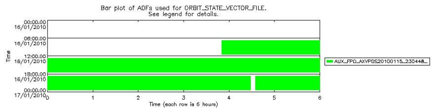
sciamachy_daily_report_level0_KSPT_L0_4303_N_20100116_7.PNG
