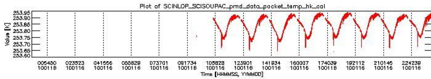
sciamachy_daily_report_level0_KSPT_L0_4303_N_20100116_3.PNG
