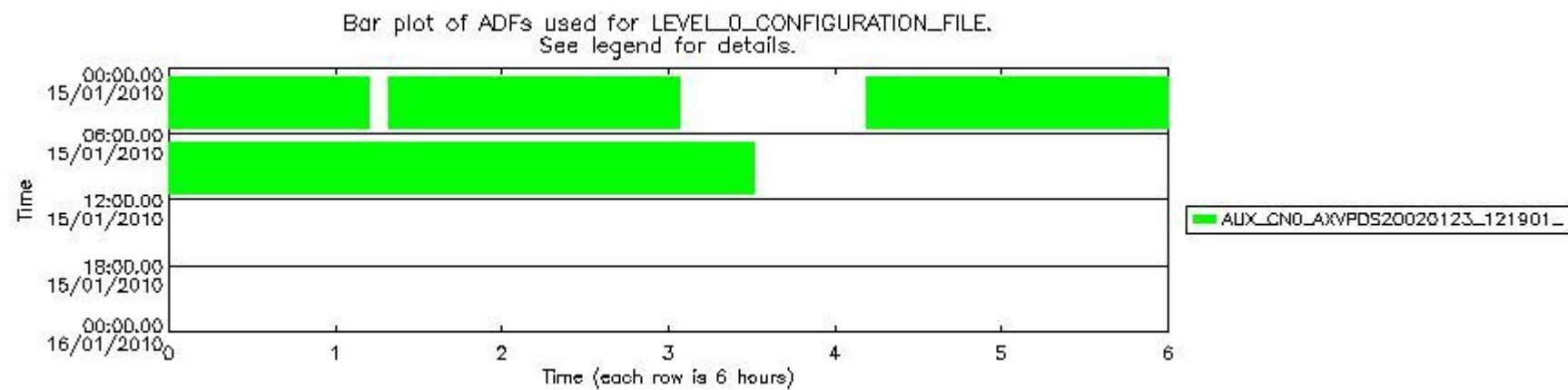
sciamachy_daily_report_level0_KSPT_L0_4303_N_20100115_6.PNG
