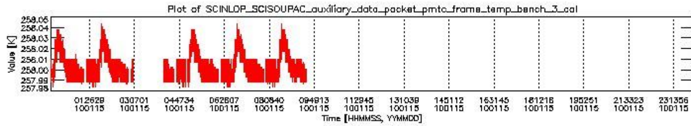
sciamachy_daily_report_level0_KSPT_L0_4303_N_20100115_2.PNG
