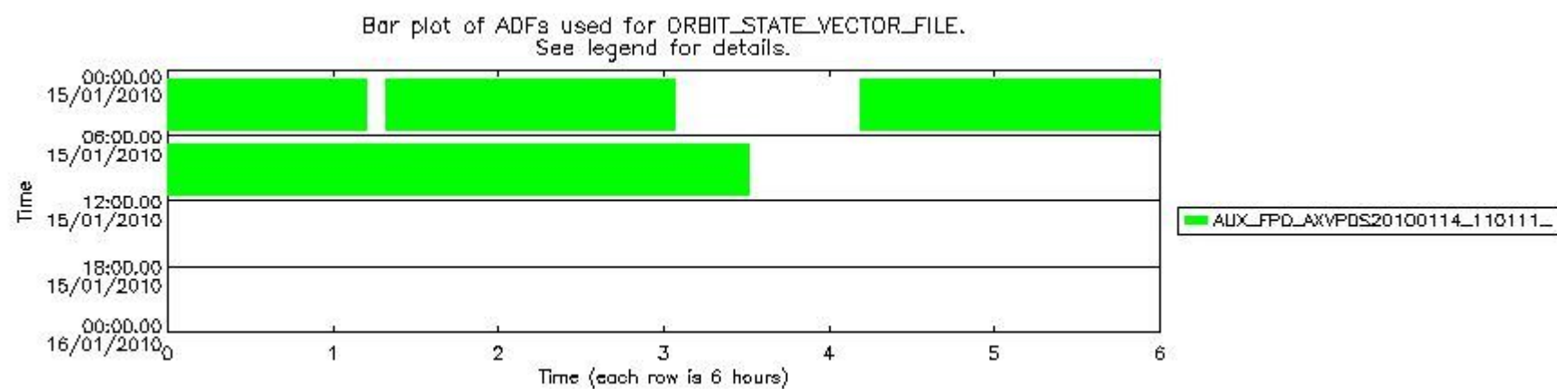
sciamachy_daily_report_level0_KSPT_L0_4303_N_20100115_7.PNG
