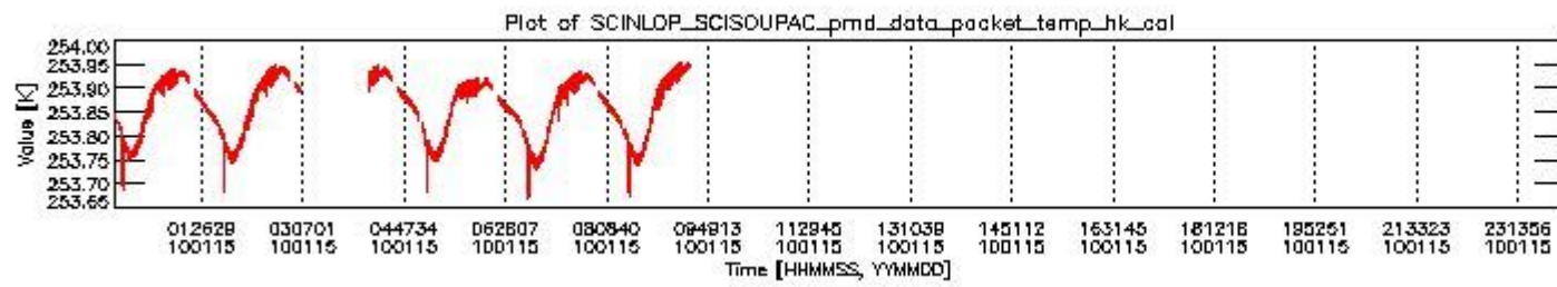
sciamachy_daily_report_level0_KSPT_L0_4303_N_20100115_3.PNG
