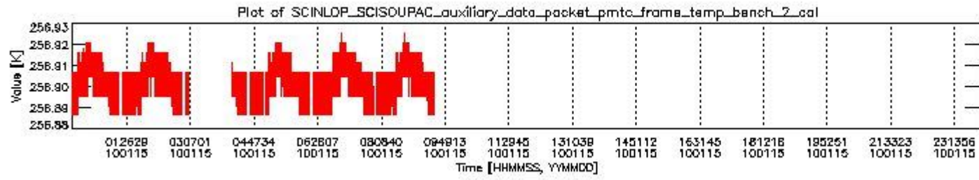
sciamachy_daily_report_level0_KSPT_L0_4303_N_20100115_1.PNG
