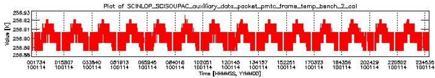
sciamachy_daily_report_level0_KSPT_L0_4303_N_20100114_1.PNG
