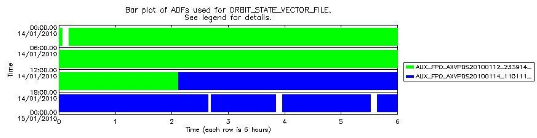
sciamachy_daily_report_level0_KSPT_L0_4303_N_20100114_7.PNG
