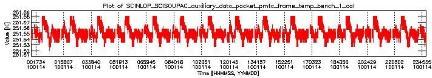
sciamachy_daily_report_level0_KSPT_L0_4303_N_20100114_0.PNG
