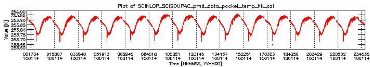
sciamachy_daily_report_level0_KSPT_L0_4303_N_20100114_3.PNG
