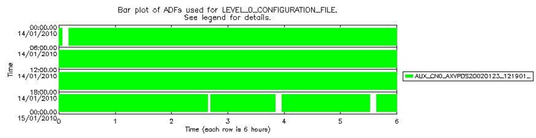
sciamachy_daily_report_level0_KSPT_L0_4303_N_20100114_6.PNG
