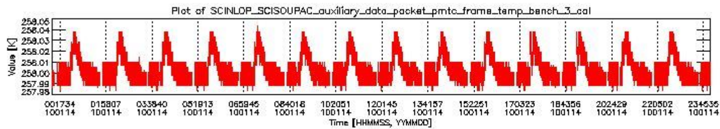
sciamachy_daily_report_level0_KSPT_L0_4303_N_20100114_2.PNG
