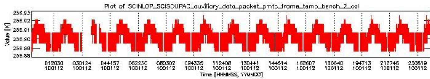
sciamachy_daily_report_level0_KSPT_L0_4303_N_20100112_1.PNG
