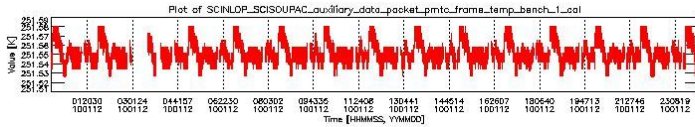
sciamachy_daily_report_level0_KSPT_L0_4303_N_20100112_0.PNG
