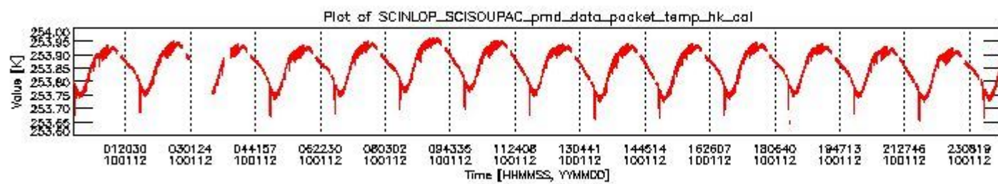
sciamachy_daily_report_level0_KSPT_L0_4303_N_20100112_3.PNG
