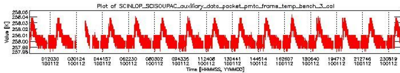
sciamachy_daily_report_level0_KSPT_L0_4303_N_20100112_2.PNG
