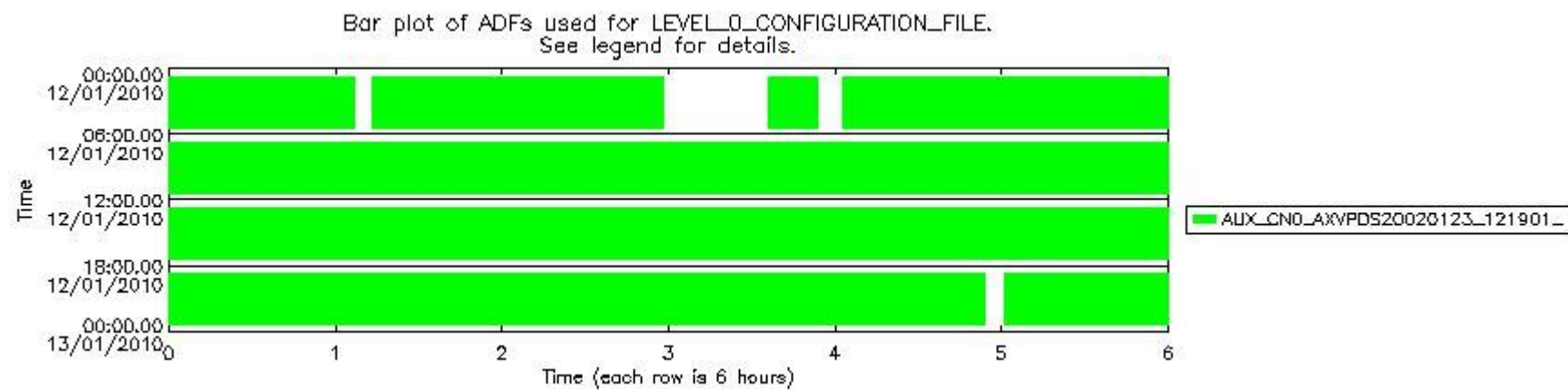
sciamachy_daily_report_level0_KSPT_L0_4303_N_20100112_6.PNG
