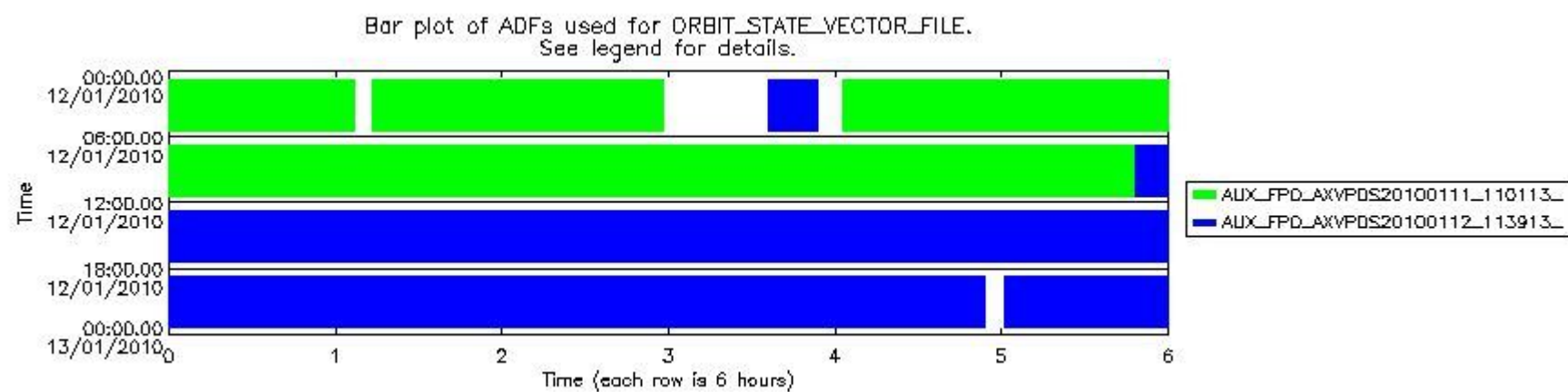
sciamachy_daily_report_level0_KSPT_L0_4303_N_20100112_7.PNG
