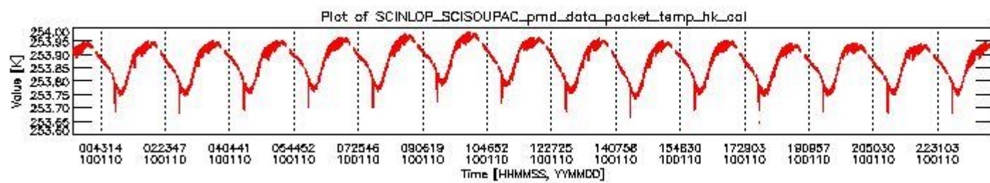
sciamachy_daily_report_level0_KSPT_L0_4303_N_20100110_3.PNG
