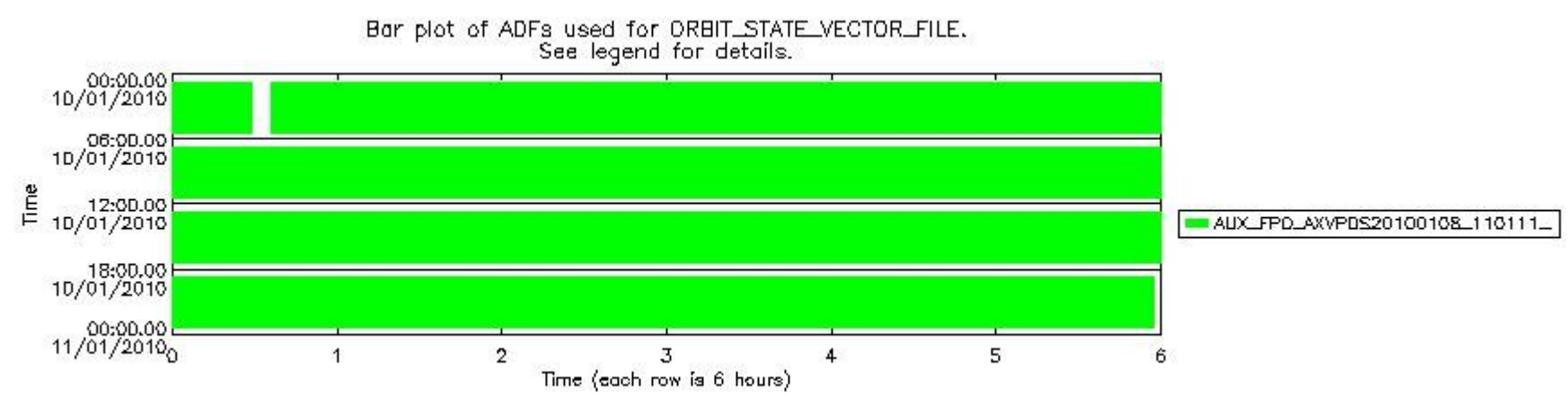
sciamachy_daily_report_level0_KSPT_L0_4303_N_20100110_7.PNG
