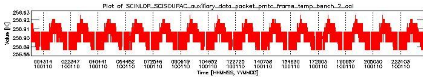
sciamachy_daily_report_level0_KSPT_L0_4303_N_20100110_1.PNG
