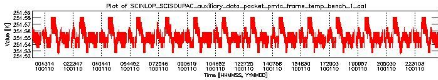
sciamachy_daily_report_level0_KSPT_L0_4303_N_20100110_0.PNG
