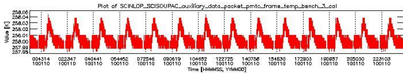
sciamachy_daily_report_level0_KSPT_L0_4303_N_20100110_2.PNG
