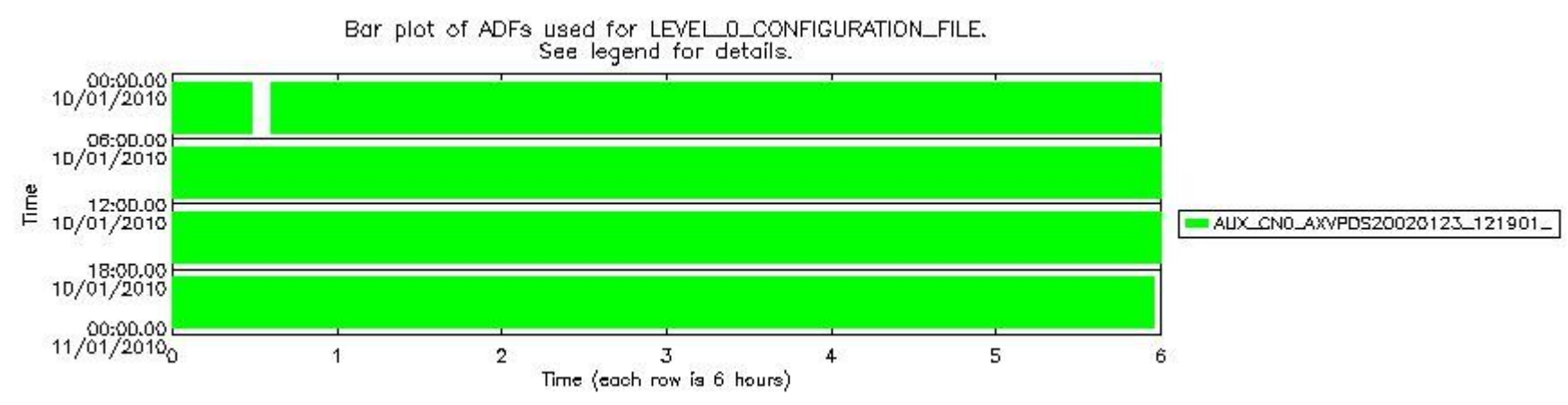
sciamachy_daily_report_level0_KSPT_L0_4303_N_20100110_6.PNG
