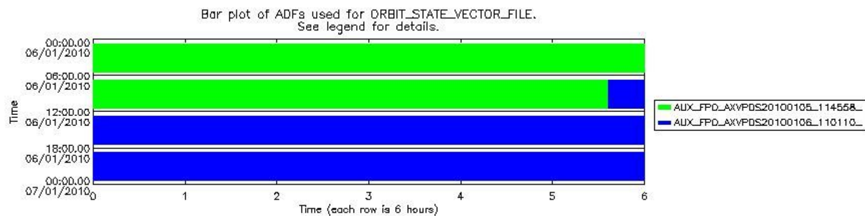
sciamachy_daily_report_level0_KSPT_L0_4303_N_20100106_7.PNG
