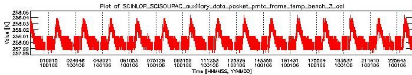
sciamachy_daily_report_level0_KSPT_L0_4303_N_20100106_2.PNG
