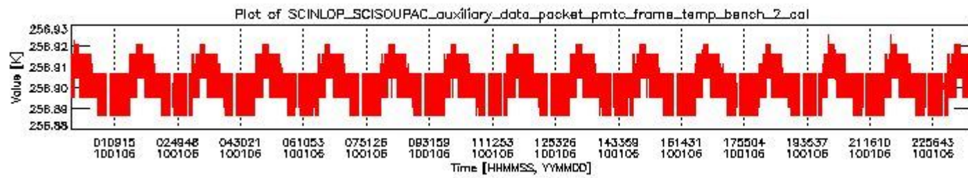
sciamachy_daily_report_level0_KSPT_L0_4303_N_20100106_1.PNG
