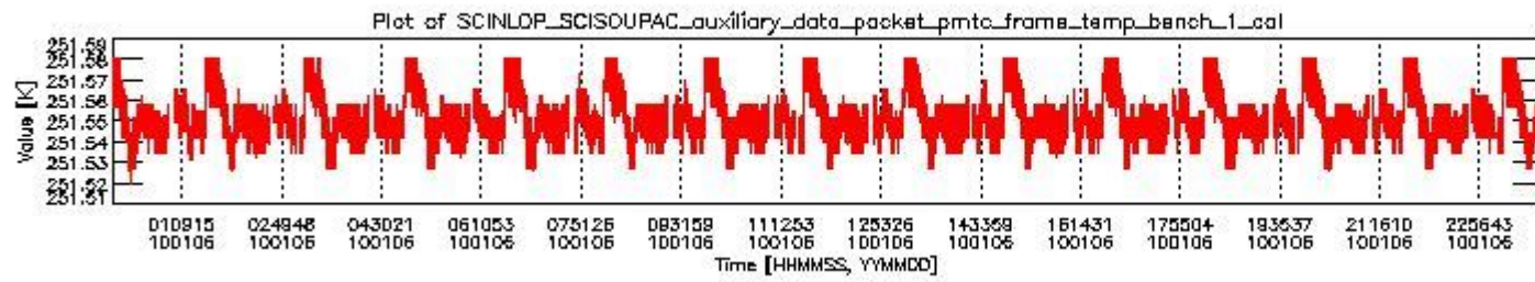
sciamachy_daily_report_level0_KSPT_L0_4303_N_20100106_0.PNG
