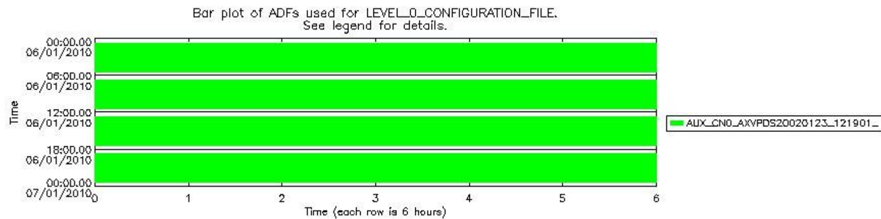
sciamachy_daily_report_level0_KSPT_L0_4303_N_20100106_6.PNG
