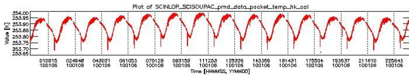
sciamachy_daily_report_level0_KSPT_L0_4303_N_20100106_3.PNG
