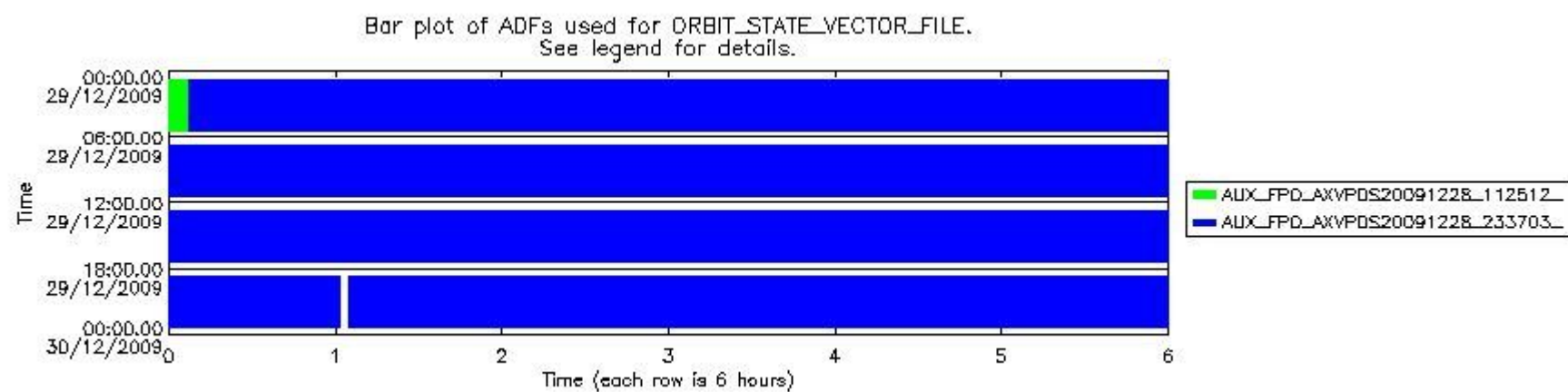
sciamachy_daily_report_level0_KSPT_L0_4303_N_20091229_7.PNG
