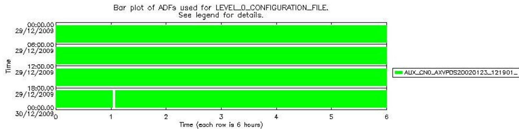
sciamachy_daily_report_level0_KSPT_L0_4303_N_20091229_6.PNG
