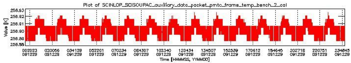
sciamachy_daily_report_level0_KSPT_L0_4303_N_20091229_1.PNG
