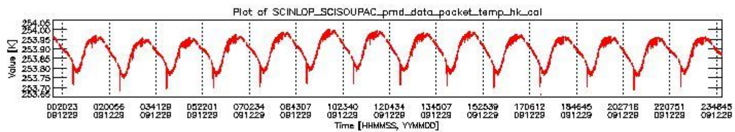
sciamachy_daily_report_level0_KSPT_L0_4303_N_20091229_3.PNG
