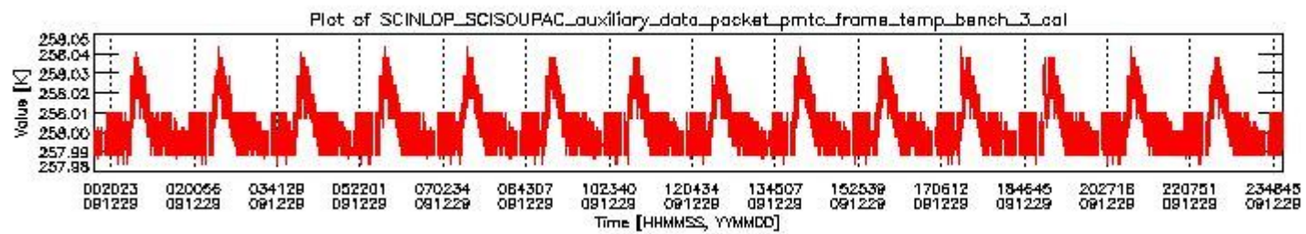
sciamachy_daily_report_level0_KSPT_L0_4303_N_20091229_2.PNG
