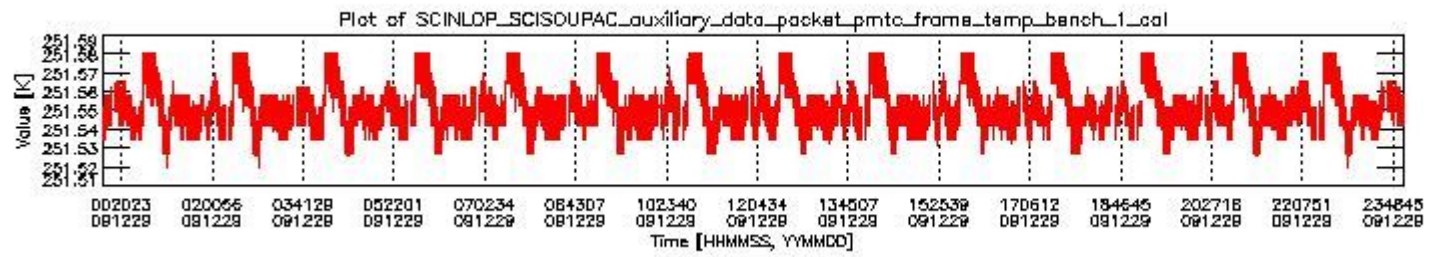
sciamachy_daily_report_level0_KSPT_L0_4303_N_20091229_0.PNG
