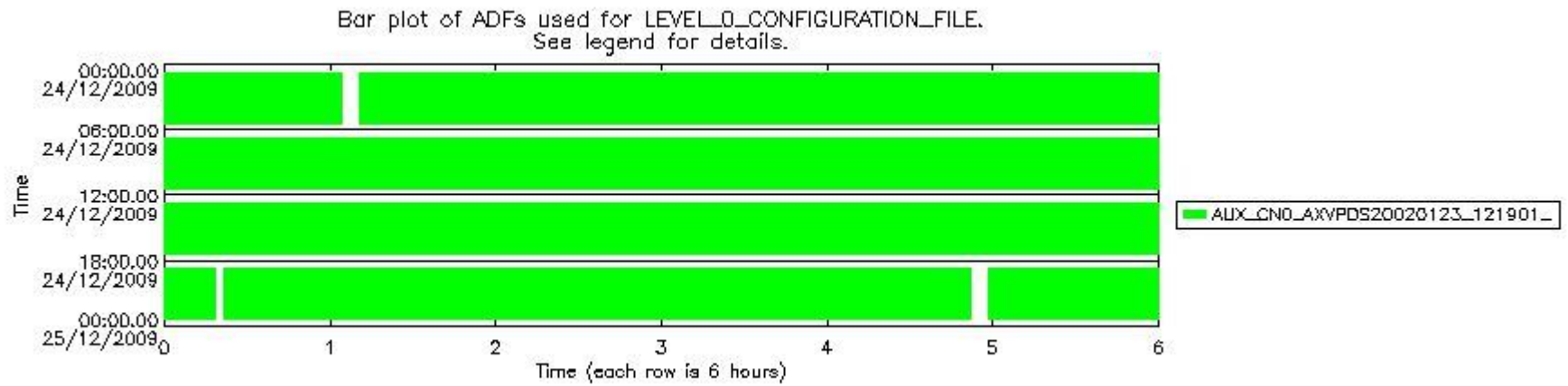
sciamachy_daily_report_level0_KSPT_L0_4303_N_20091224_6.PNG
