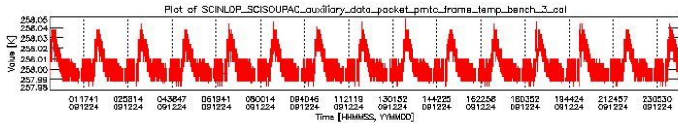
sciamachy_daily_report_level0_KSPT_L0_4303_N_20091224_2.PNG
