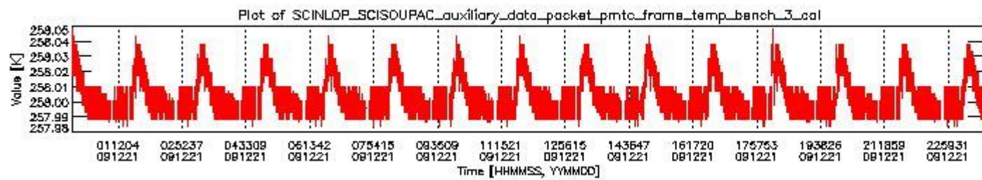
sciamachy_daily_report_level0_KSPT_L0_4303_N_20091221_2.PNG
