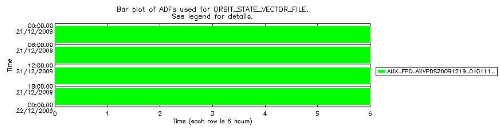
sciamachy_daily_report_level0_KSPT_L0_4303_N_20091221_7.PNG
