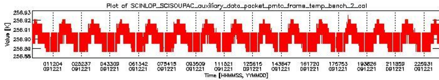
sciamachy_daily_report_level0_KSPT_L0_4303_N_20091221_1.PNG
