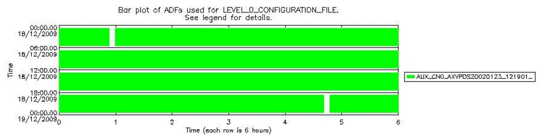
sciamachy_daily_report_level0_KSPT_L0_4303_N_20091218_6.PNG
