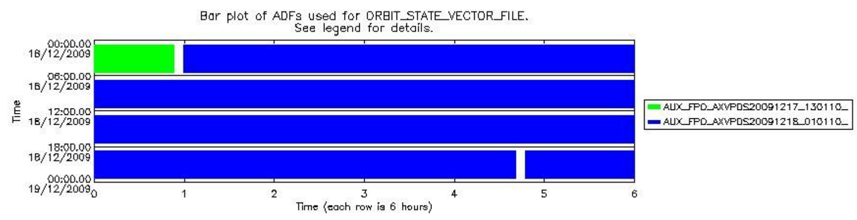
sciamachy_daily_report_level0_KSPT_L0_4303_N_20091218_7.PNG
