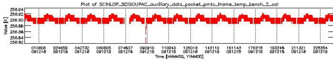
sciamachy_daily_report_level0_KSPT_L0_4303_N_20091218_1.PNG
