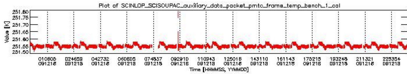
sciamachy_daily_report_level0_KSPT_L0_4303_N_20091218_0.PNG
