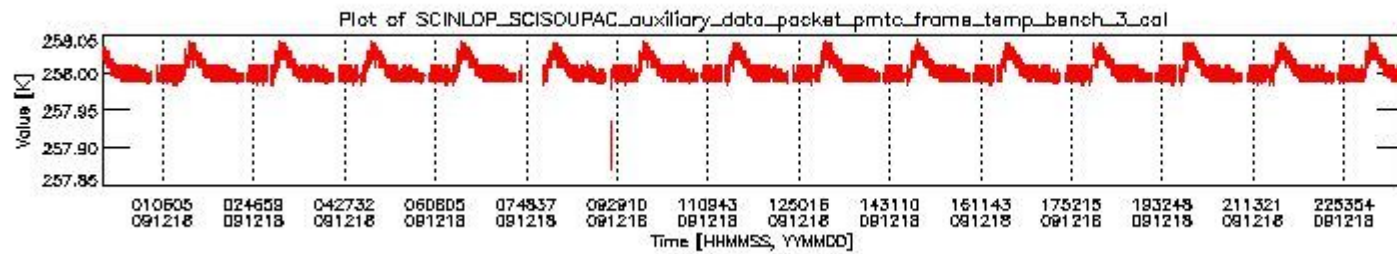
sciamachy_daily_report_level0_KSPT_L0_4303_N_20091218_2.PNG
