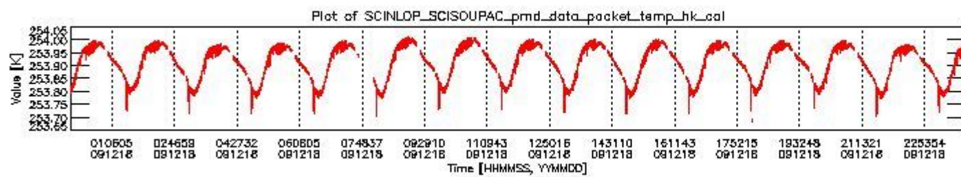
sciamachy_daily_report_level0_KSPT_L0_4303_N_20091218_3.PNG
