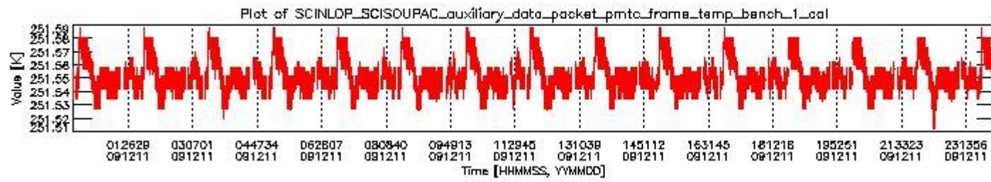
sciamachy_daily_report_level0_KSPT_L0_4303_N_20091211_0.PNG
