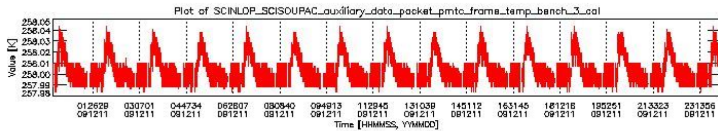
sciamachy_daily_report_level0_KSPT_L0_4303_N_20091211_2.PNG
