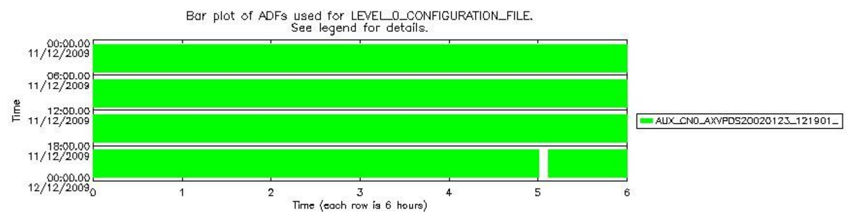
sciamachy_daily_report_level0_KSPT_L0_4303_N_20091211_6.PNG
