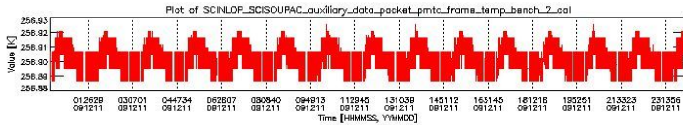
sciamachy_daily_report_level0_KSPT_L0_4303_N_20091211_1.PNG
