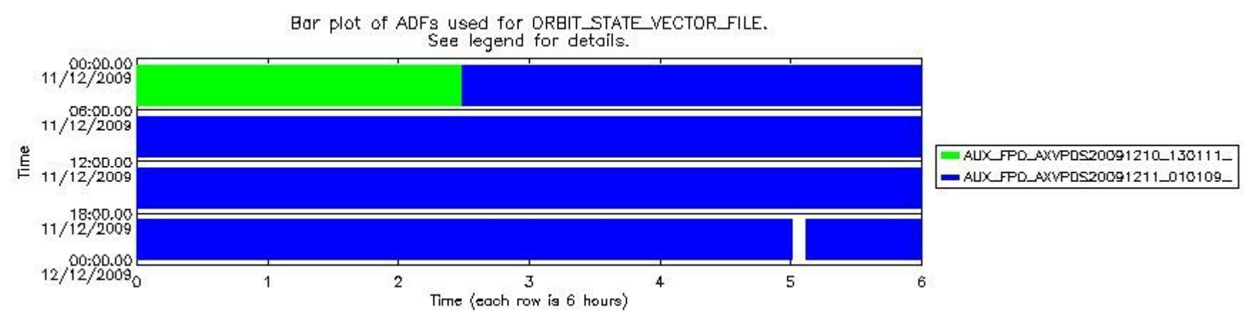
sciamachy_daily_report_level0_KSPT_L0_4303_N_20091211_7.PNG
