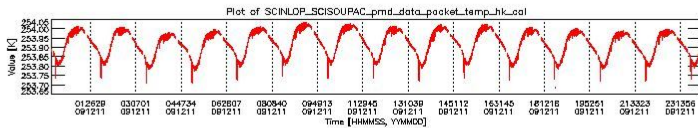
sciamachy_daily_report_level0_KSPT_L0_4303_N_20091211_3.PNG
