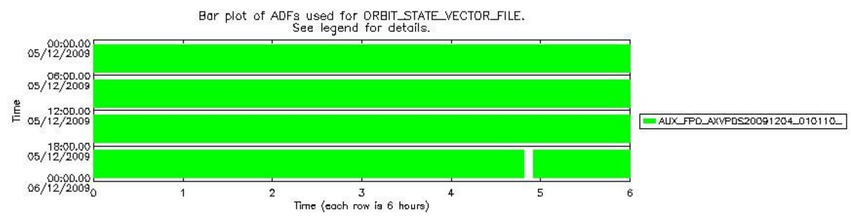
sciamachy_daily_report_level0_KSPT_L0_4303_N_20091205_7.PNG
