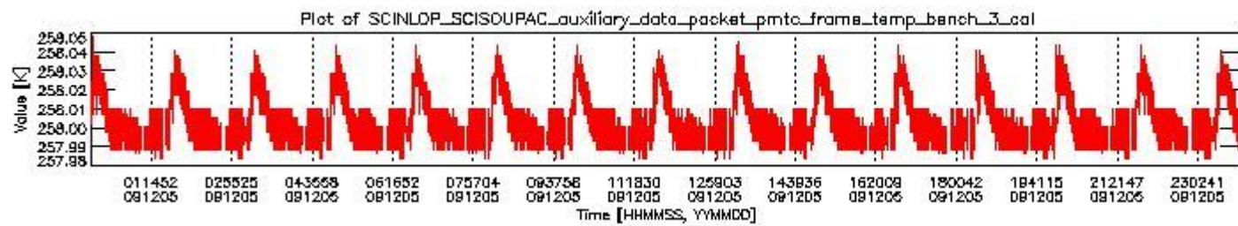
sciamachy_daily_report_level0_KSPT_L0_4303_N_20091205_2.PNG
