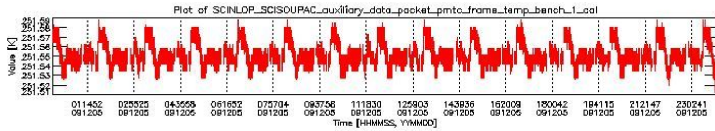
sciamachy_daily_report_level0_KSPT_L0_4303_N_20091205_0.PNG
