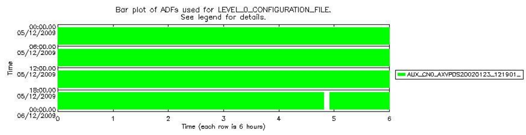
sciamachy_daily_report_level0_KSPT_L0_4303_N_20091205_6.PNG
