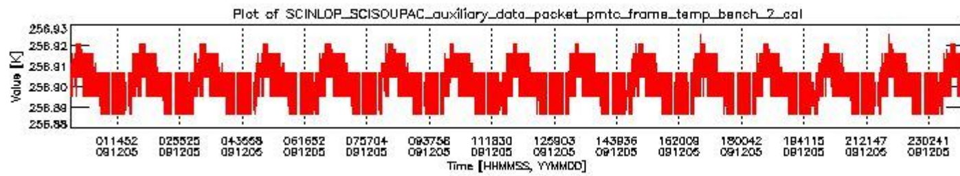
sciamachy_daily_report_level0_KSPT_L0_4303_N_20091205_1.PNG
