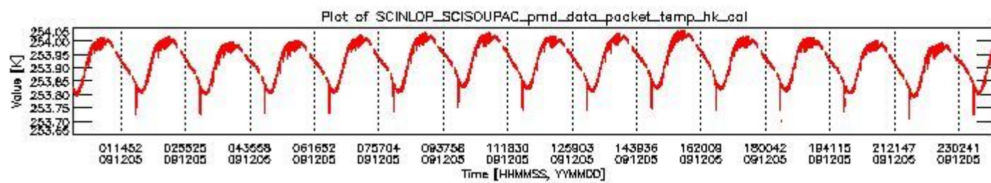
sciamachy_daily_report_level0_KSPT_L0_4303_N_20091205_3.PNG
