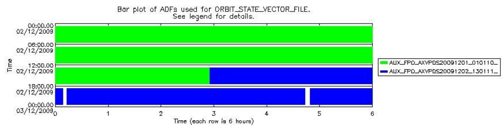
sciamachy_daily_report_level0_KSPT_L0_4303_N_20091202_7.PNG
