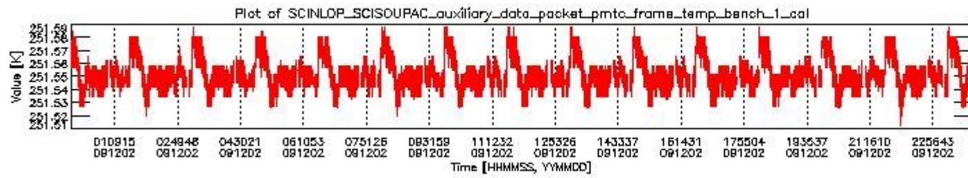
sciamachy_daily_report_level0_KSPT_L0_4303_N_20091202_0.PNG
