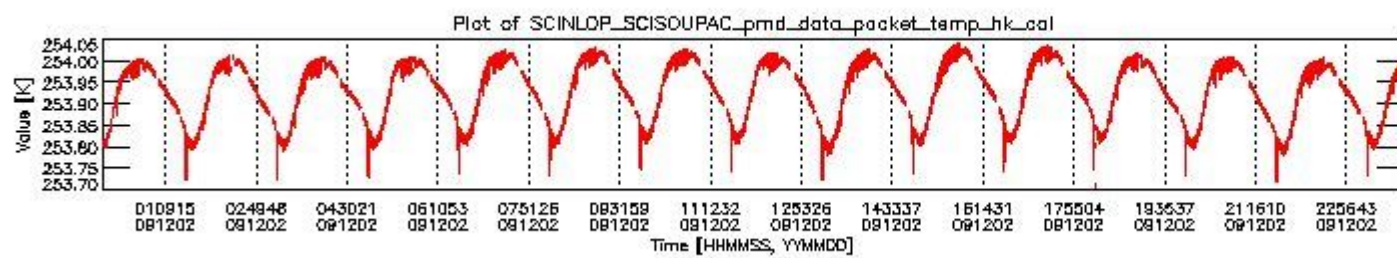
sciamachy_daily_report_level0_KSPT_L0_4303_N_20091202_3.PNG
