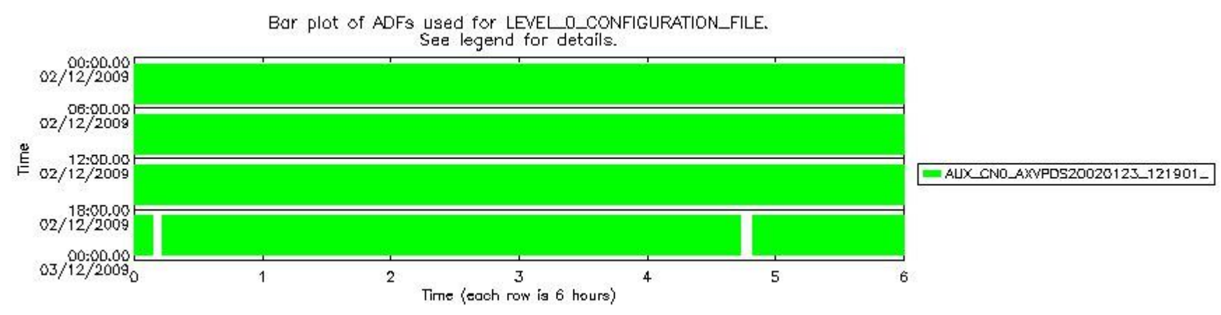
sciamachy_daily_report_level0_KSPT_L0_4303_N_20091202_6.PNG
