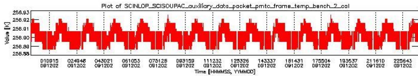
sciamachy_daily_report_level0_KSPT_L0_4303_N_20091202_1.PNG
