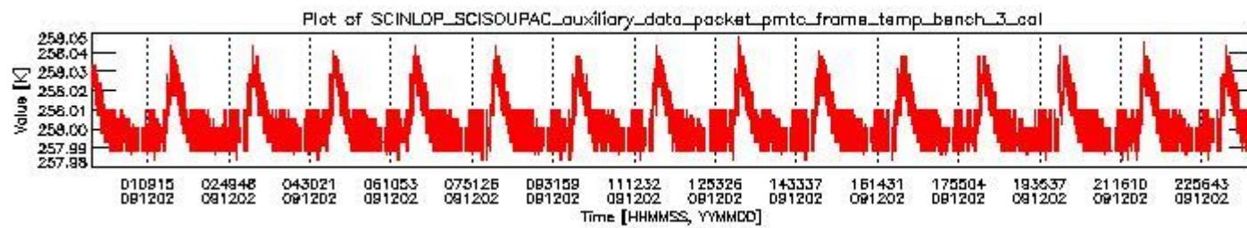
sciamachy_daily_report_level0_KSPT_L0_4303_N_20091202_2.PNG
