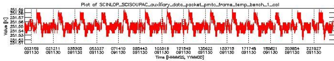
sciamachy_daily_report_level0_KSPT_L0_4303_N_20091130_0.PNG
