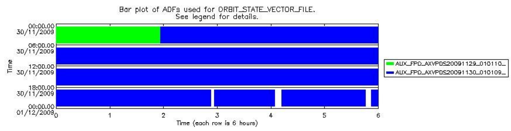
sciamachy_daily_report_level0_KSPT_L0_4303_N_20091130_7.PNG
