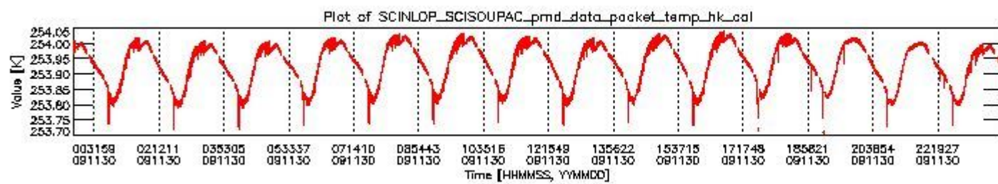
sciamachy_daily_report_level0_KSPT_L0_4303_N_20091130_3.PNG
