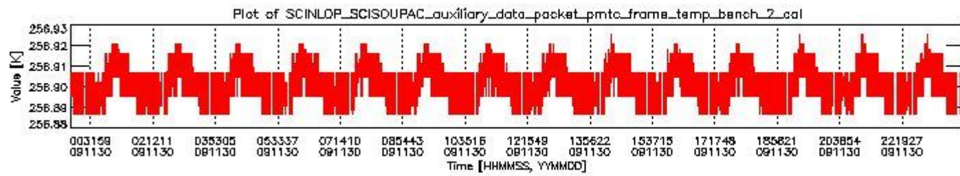
sciamachy_daily_report_level0_KSPT_L0_4303_N_20091130_1.PNG
