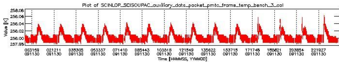
sciamachy_daily_report_level0_KSPT_L0_4303_N_20091130_2.PNG
