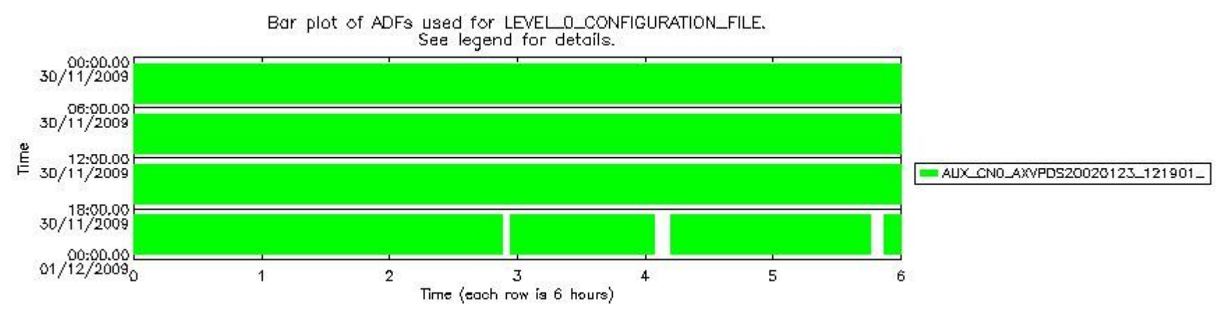
sciamachy_daily_report_level0_KSPT_L0_4303_N_20091130_6.PNG
