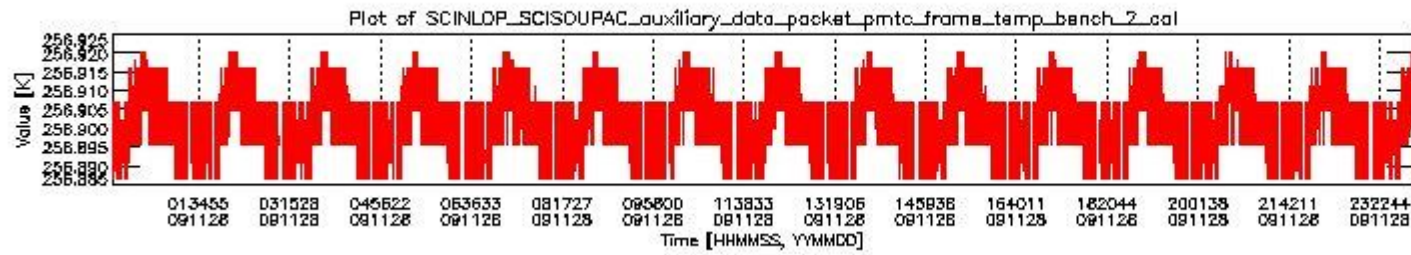
sciamachy_daily_report_level0_KSPT_L0_4303_N_20091128_1.PNG
