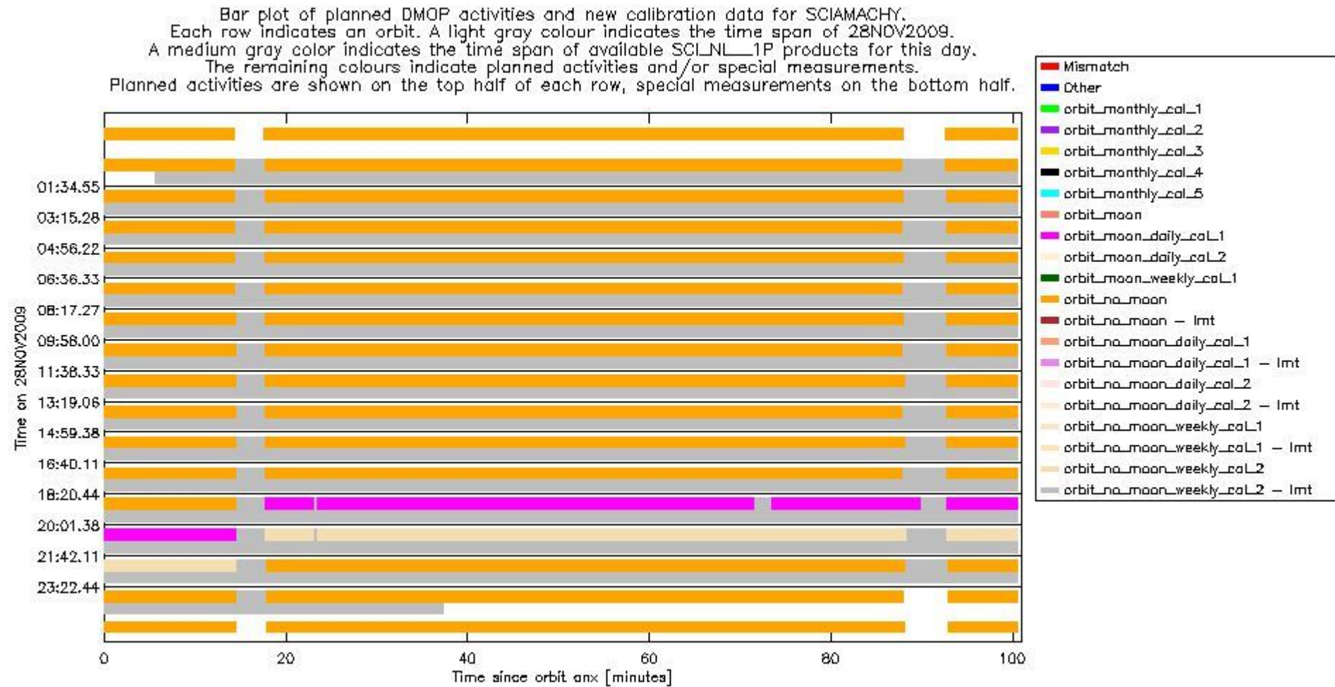
sciamachy_daily_report_level0_KSPT_L0_4303_N_20091128_5.PNG
