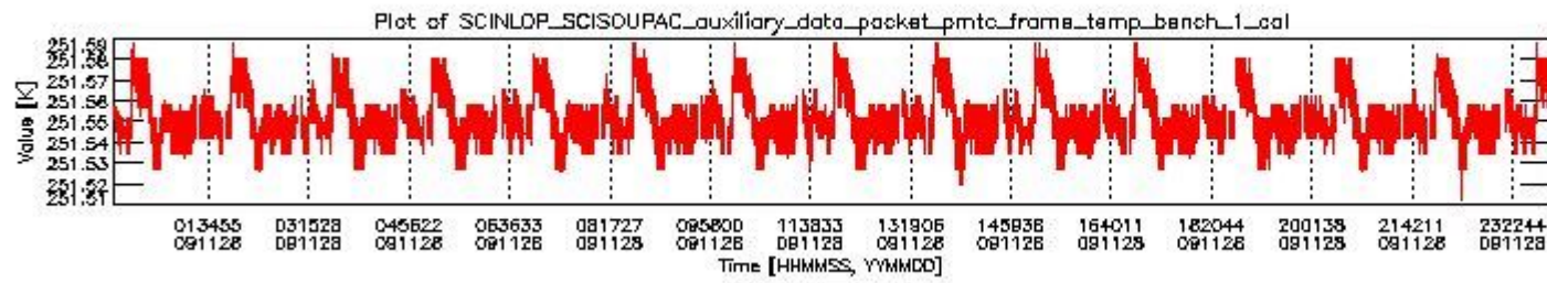
sciamachy_daily_report_level0_KSPT_L0_4303_N_20091128_0.PNG
