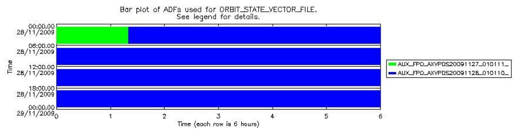
sciamachy_daily_report_level0_KSPT_L0_4303_N_20091128_7.PNG
