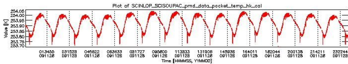
sciamachy_daily_report_level0_KSPT_L0_4303_N_20091128_3.PNG
