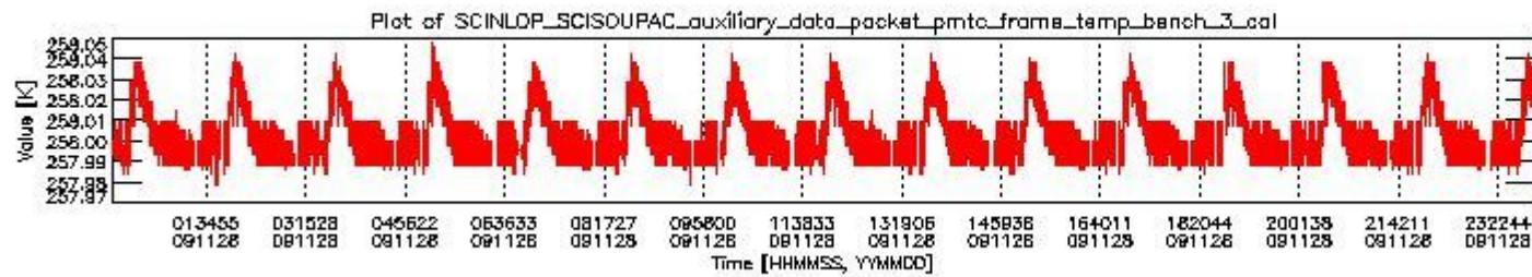
sciamachy_daily_report_level0_KSPT_L0_4303_N_20091128_2.PNG
