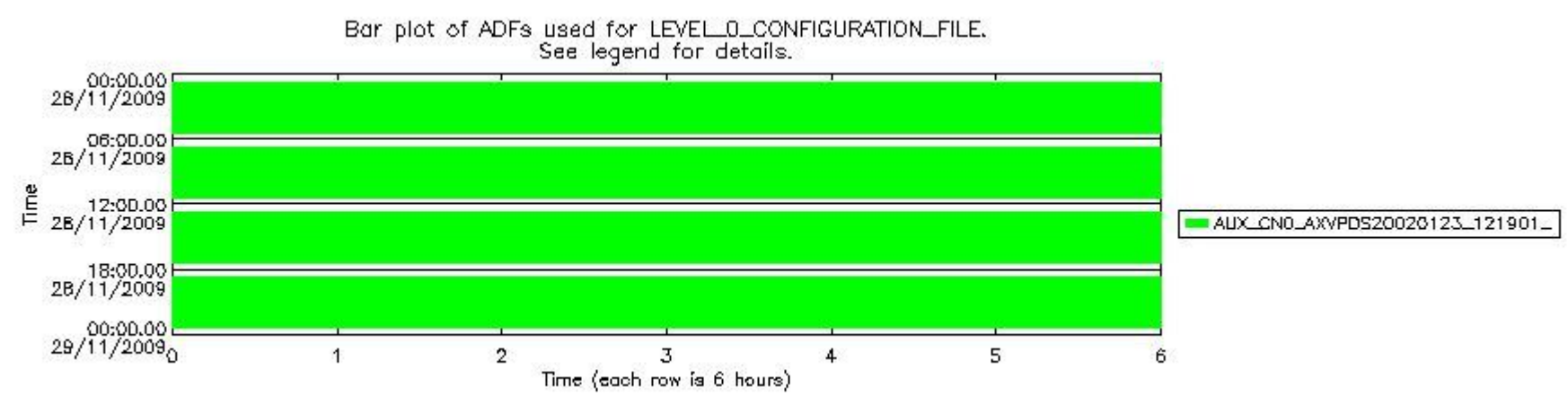
sciamachy_daily_report_level0_KSPT_L0_4303_N_20091128_6.PNG
