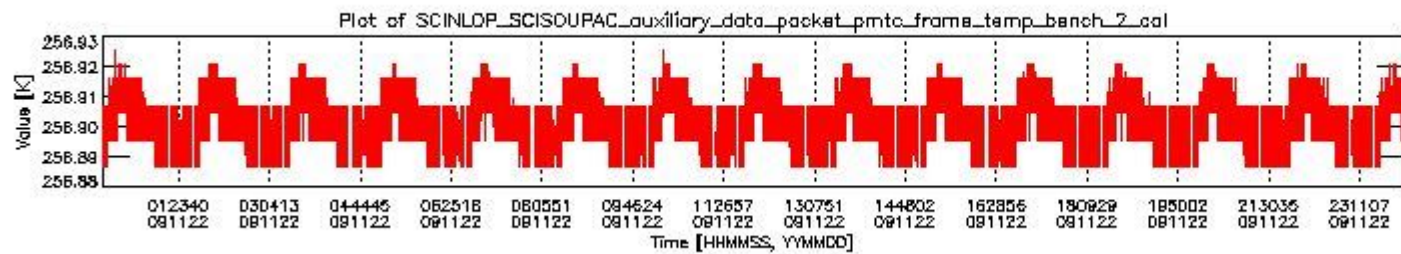
sciamachy_daily_report_level0_KSPT_L0_4303_N_20091122_1.PNG
