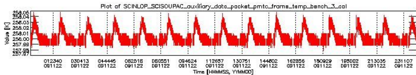
sciamachy_daily_report_level0_KSPT_L0_4303_N_20091122_2.PNG
