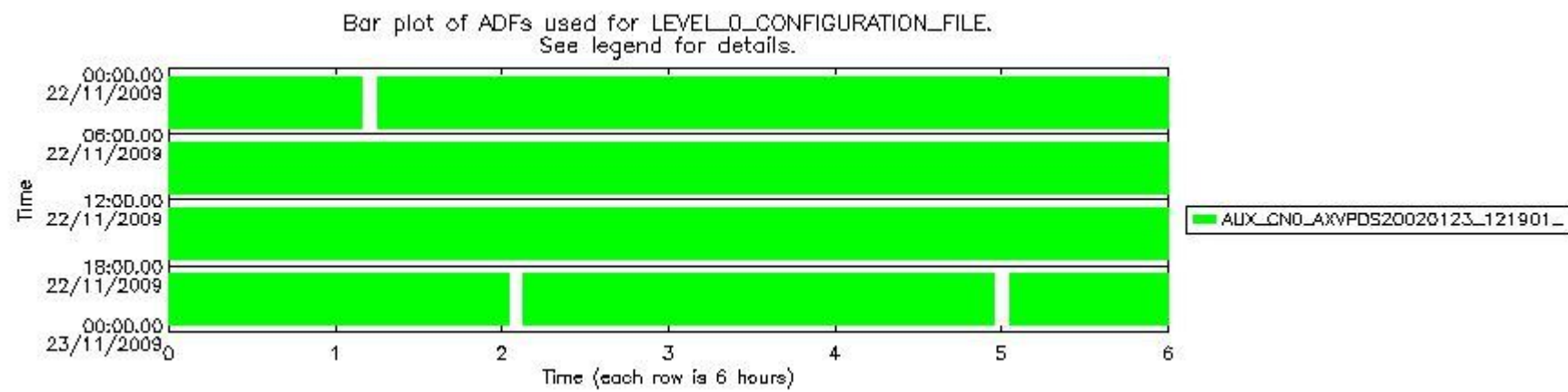
sciamachy_daily_report_level0_KSPT_L0_4303_N_20091122_6.PNG
