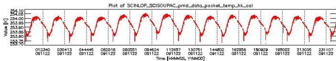
sciamachy_daily_report_level0_KSPT_L0_4303_N_20091122_3.PNG
