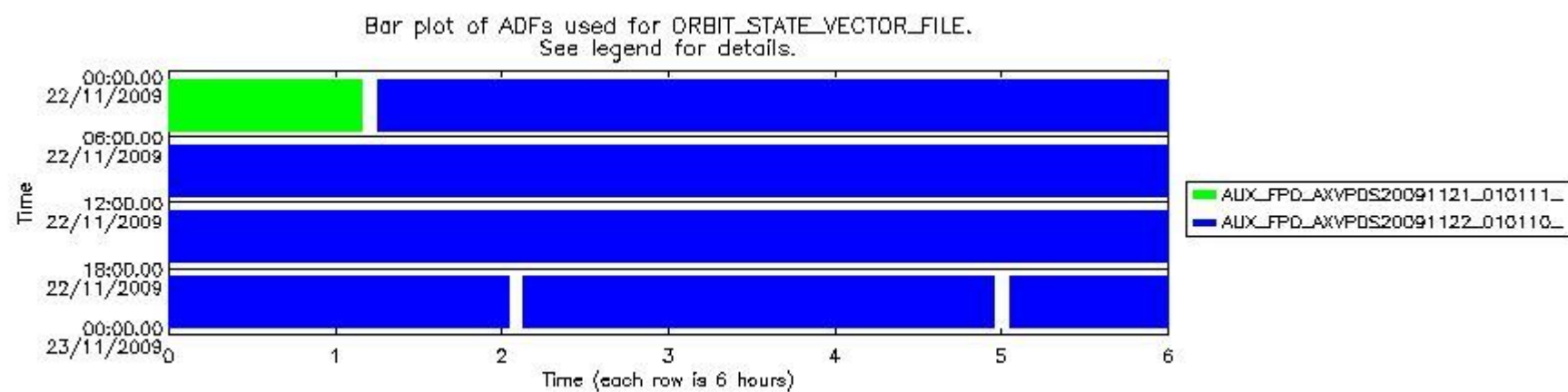
sciamachy_daily_report_level0_KSPT_L0_4303_N_20091122_7.PNG
