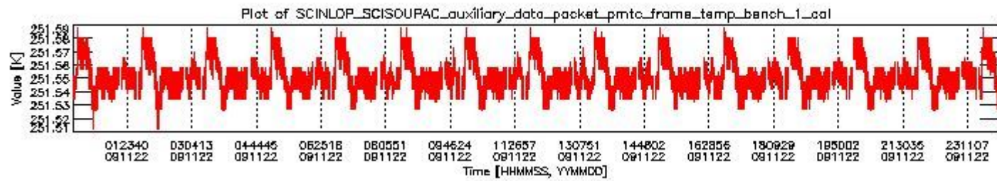
sciamachy_daily_report_level0_KSPT_L0_4303_N_20091122_0.PNG
