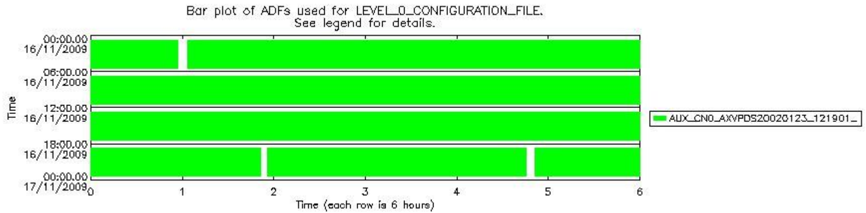
sciamachy_daily_report_level0_KSPT_L0_4303_N_20091116_6.PNG
