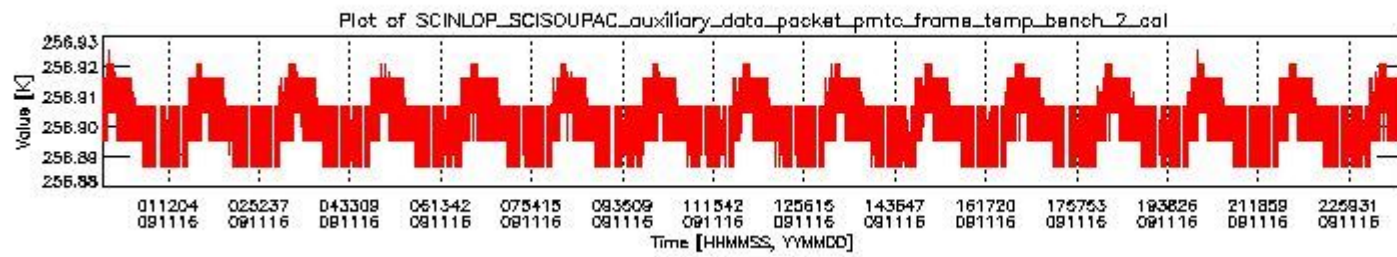
sciamachy_daily_report_level0_KSPT_L0_4303_N_20091116_1.PNG
