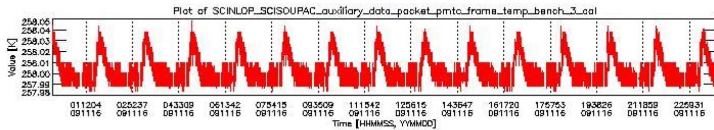
sciamachy_daily_report_level0_KSPT_L0_4303_N_20091116_2.PNG
