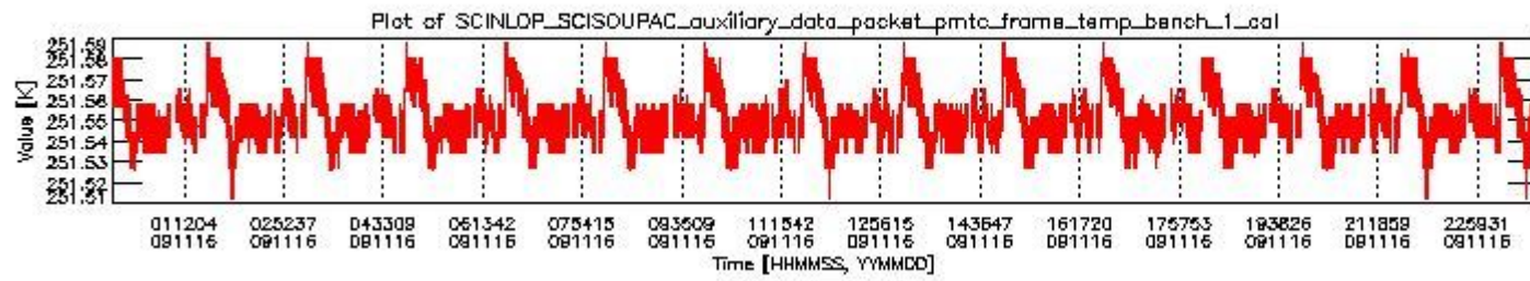
sciamachy_daily_report_level0_KSPT_L0_4303_N_20091116_0.PNG
