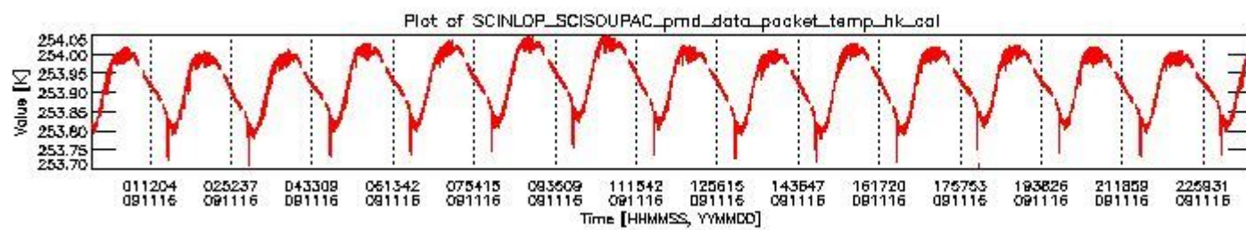
sciamachy_daily_report_level0_KSPT_L0_4303_N_20091116_3.PNG
