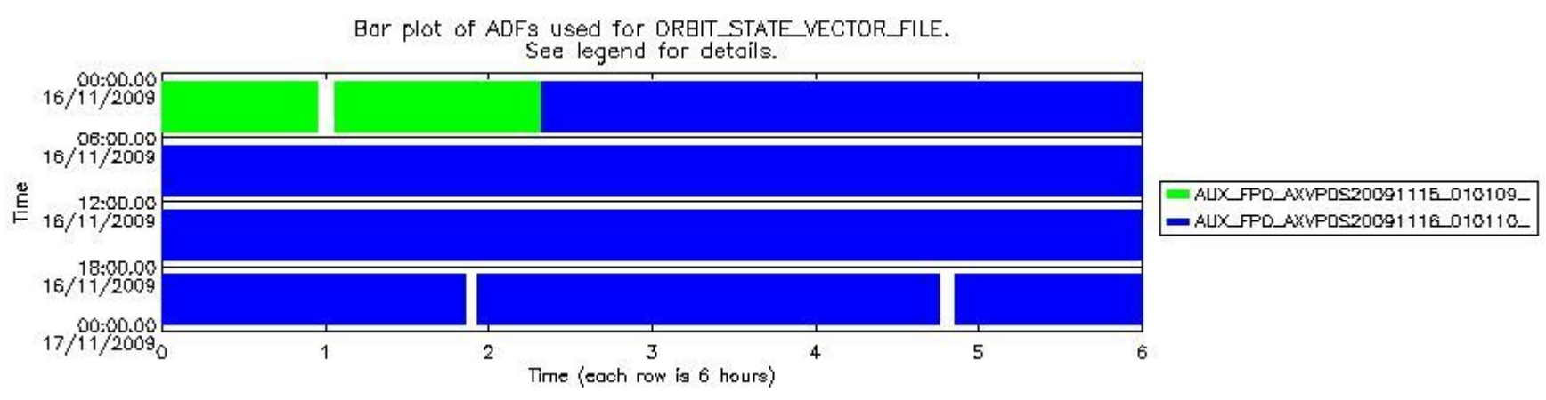
sciamachy_daily_report_level0_KSPT_L0_4303_N_20091116_7.PNG
