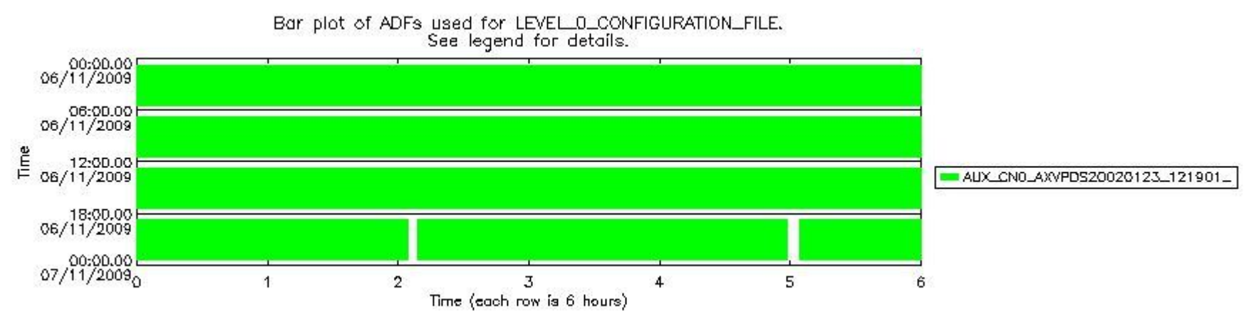
sciamachy_daily_report_level0_KSPT_L0_4303_N_20091106_6.PNG
