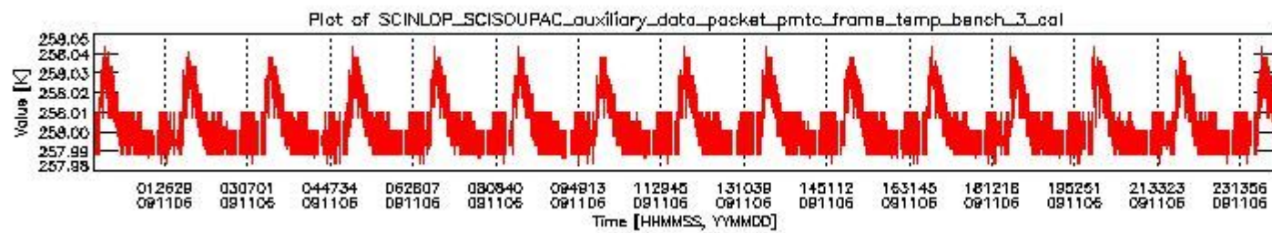
sciamachy_daily_report_level0_KSPT_L0_4303_N_20091106_2.PNG
