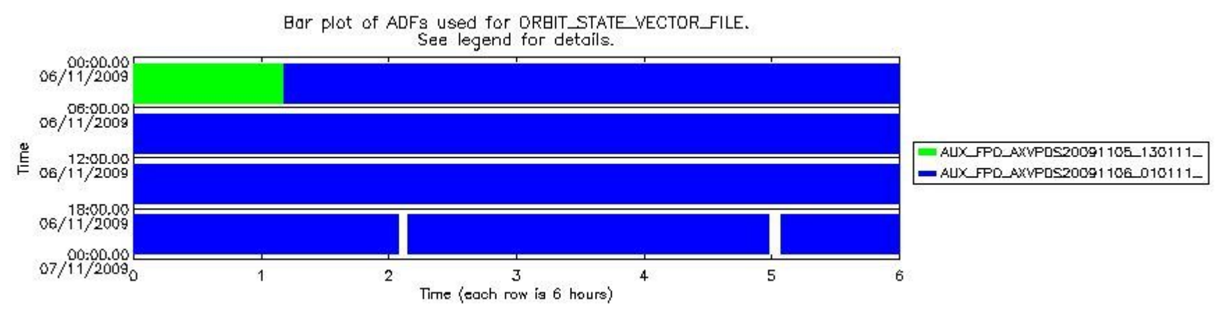
sciamachy_daily_report_level0_KSPT_L0_4303_N_20091106_7.PNG
