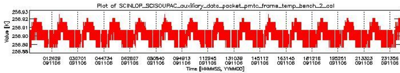
sciamachy_daily_report_level0_KSPT_L0_4303_N_20091106_1.PNG
