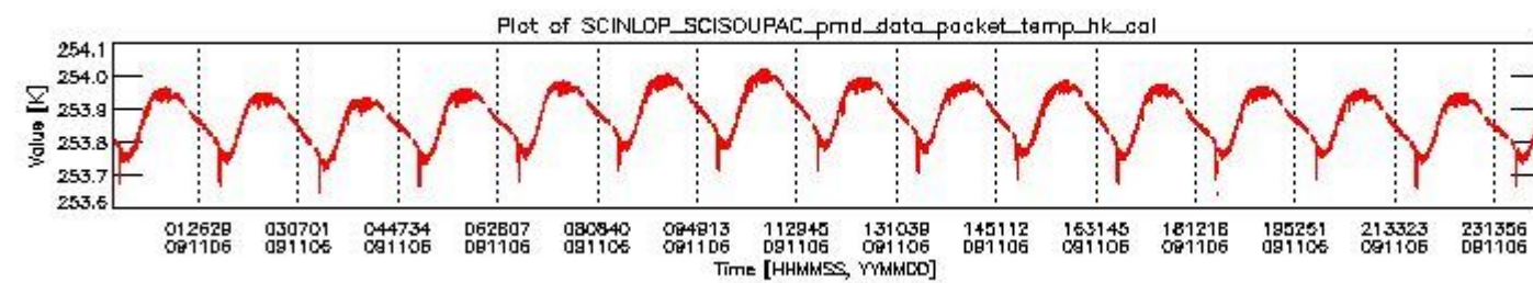
sciamachy_daily_report_level0_KSPT_L0_4303_N_20091106_3.PNG
