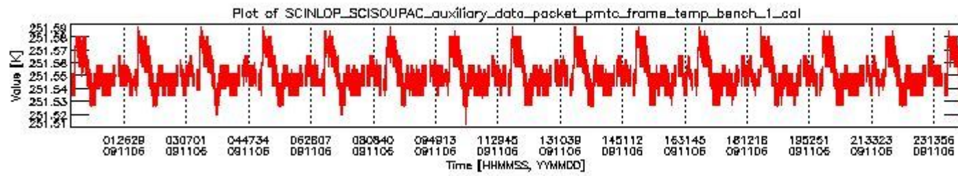
sciamachy_daily_report_level0_KSPT_L0_4303_N_20091106_0.PNG
