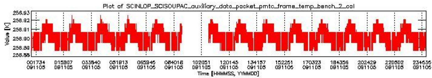
sciamachy_daily_report_level0_KSPT_L0_4303_N_20091105_1.PNG
