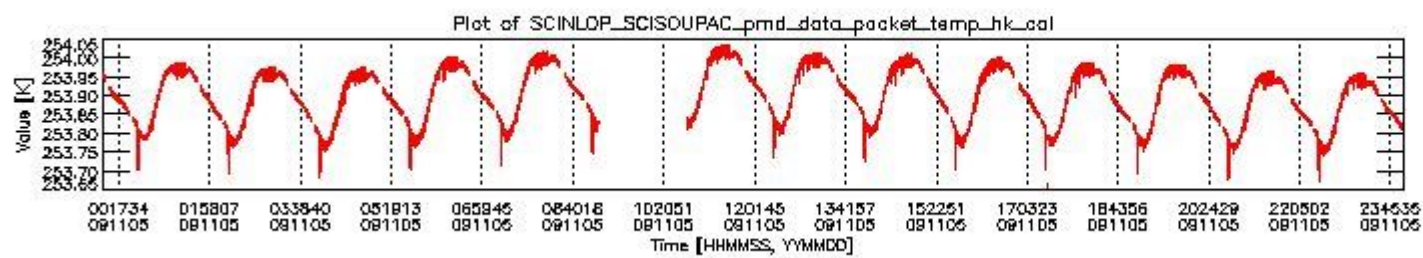
sciamachy_daily_report_level0_KSPT_L0_4303_N_20091105_3.PNG
