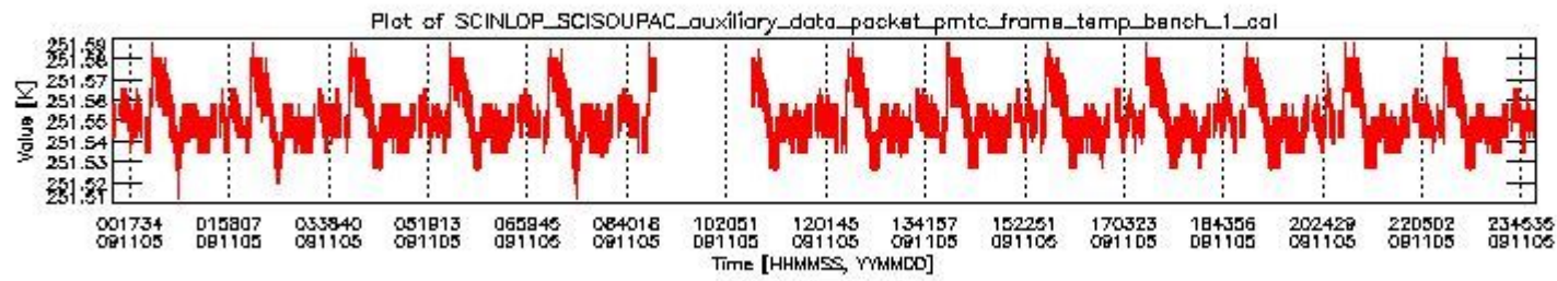
sciamachy_daily_report_level0_KSPT_L0_4303_N_20091105_0.PNG
