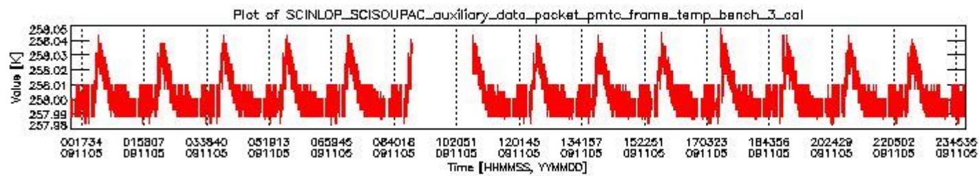
sciamachy_daily_report_level0_KSPT_L0_4303_N_20091105_2.PNG
