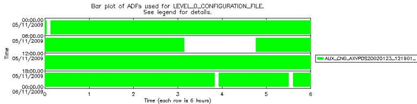
sciamachy_daily_report_level0_KSPT_L0_4303_N_20091105_6.PNG
