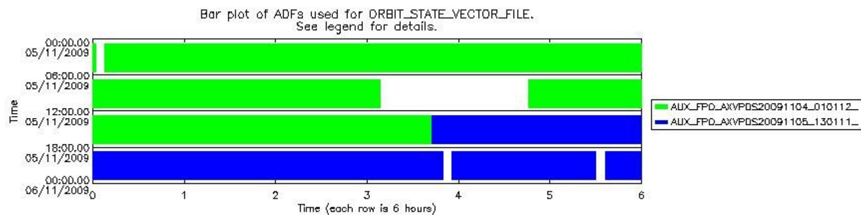
sciamachy_daily_report_level0_KSPT_L0_4303_N_20091105_7.PNG
