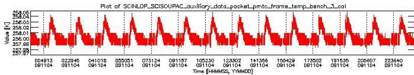
sciamachy_daily_report_level0_KSPT_L0_4303_N_20091104_2.PNG
