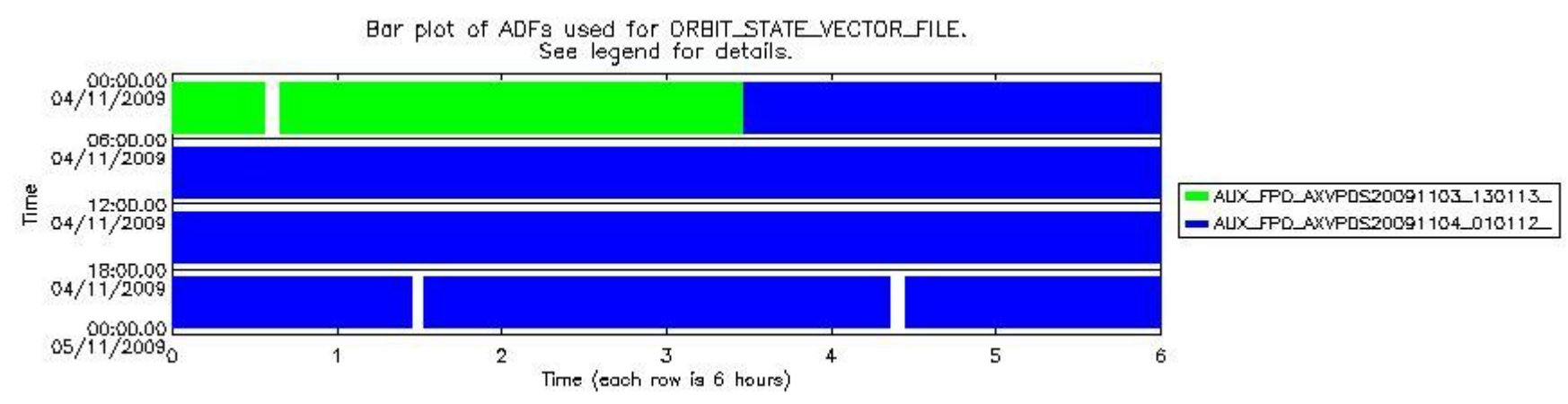
sciamachy_daily_report_level0_KSPT_L0_4303_N_20091104_7.PNG
