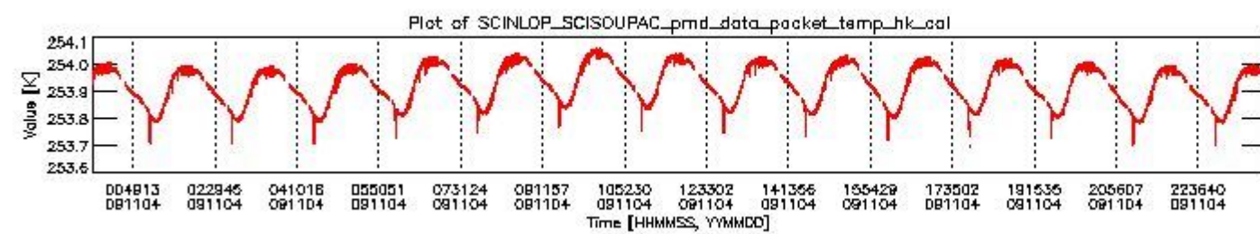
sciamachy_daily_report_level0_KSPT_L0_4303_N_20091104_3.PNG
