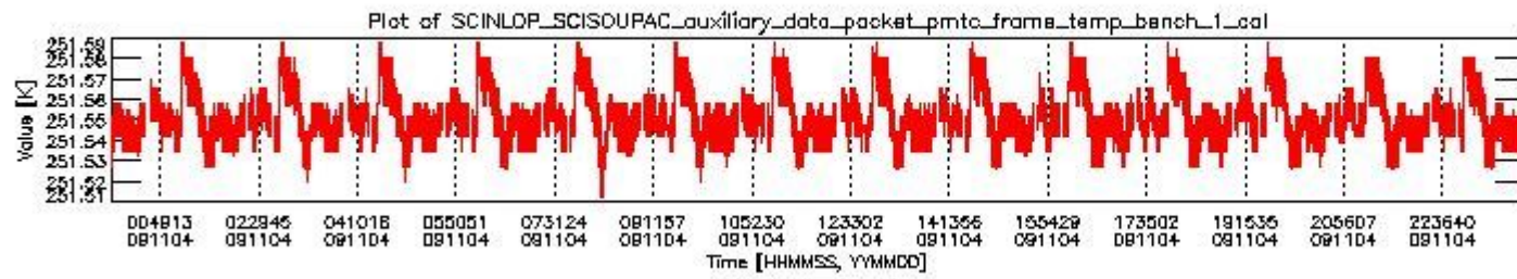
sciamachy_daily_report_level0_KSPT_L0_4303_N_20091104_0.PNG
