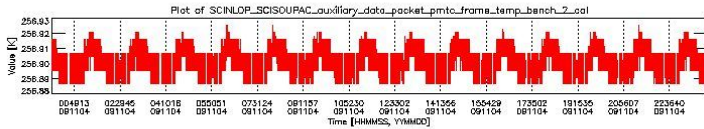
sciamachy_daily_report_level0_KSPT_L0_4303_N_20091104_1.PNG
