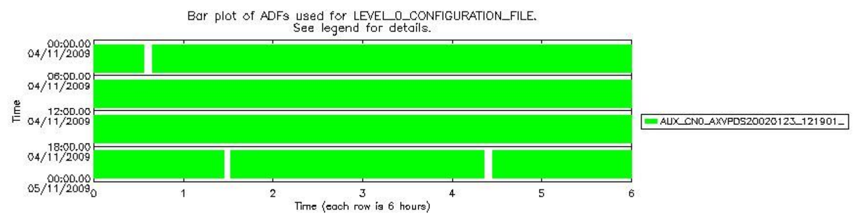
sciamachy_daily_report_level0_KSPT_L0_4303_N_20091104_6.PNG
