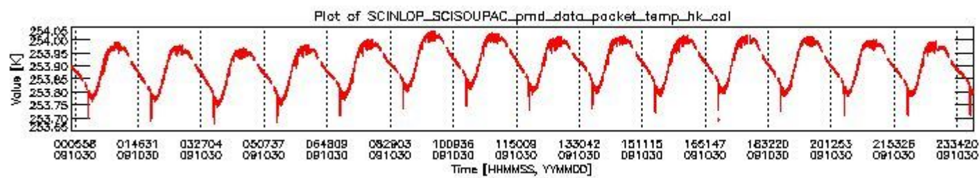
sciamachy_daily_report_level0_KSPT_L0_4303_N_20091030_3.PNG
