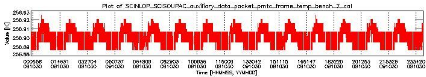
sciamachy_daily_report_level0_KSPT_L0_4303_N_20091030_1.PNG
