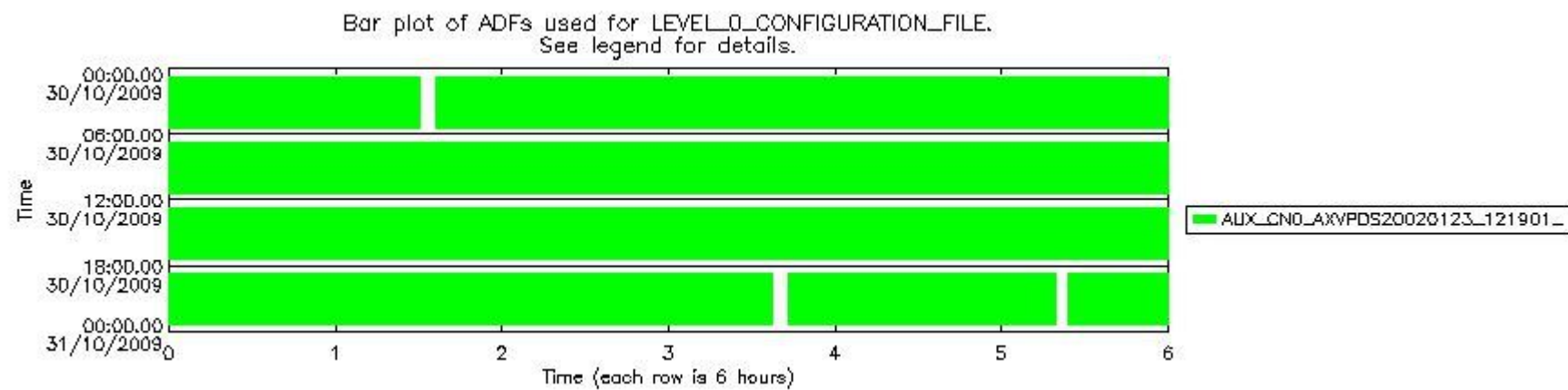
sciamachy_daily_report_level0_KSPT_L0_4303_N_20091030_6.PNG
