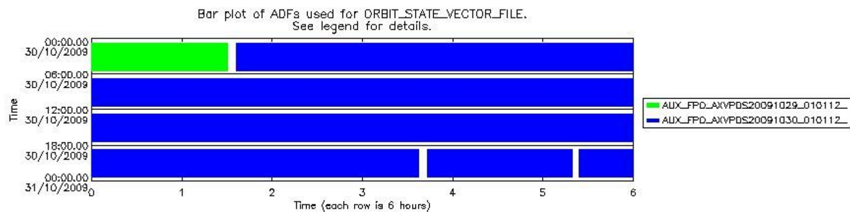
sciamachy_daily_report_level0_KSPT_L0_4303_N_20091030_7.PNG
