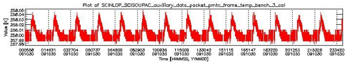
sciamachy_daily_report_level0_KSPT_L0_4303_N_20091030_2.PNG
