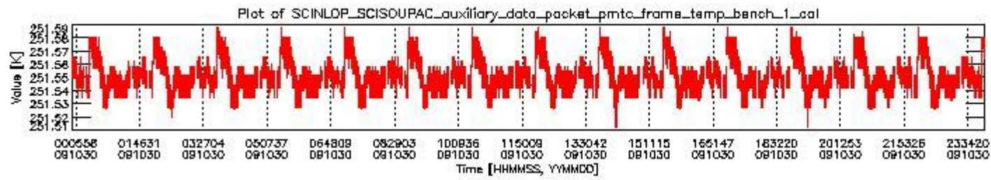
sciamachy_daily_report_level0_KSPT_L0_4303_N_20091030_0.PNG
