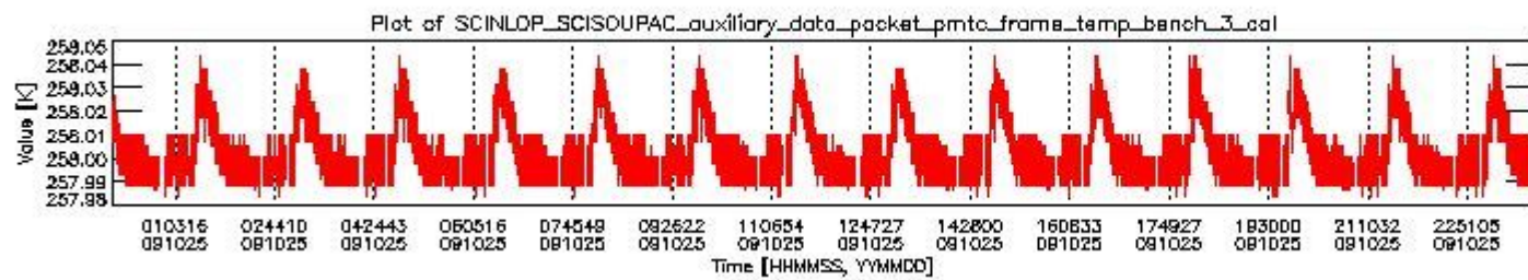
sciamachy_daily_report_level0_KSPT_L0_4303_N_20091025_2.PNG
