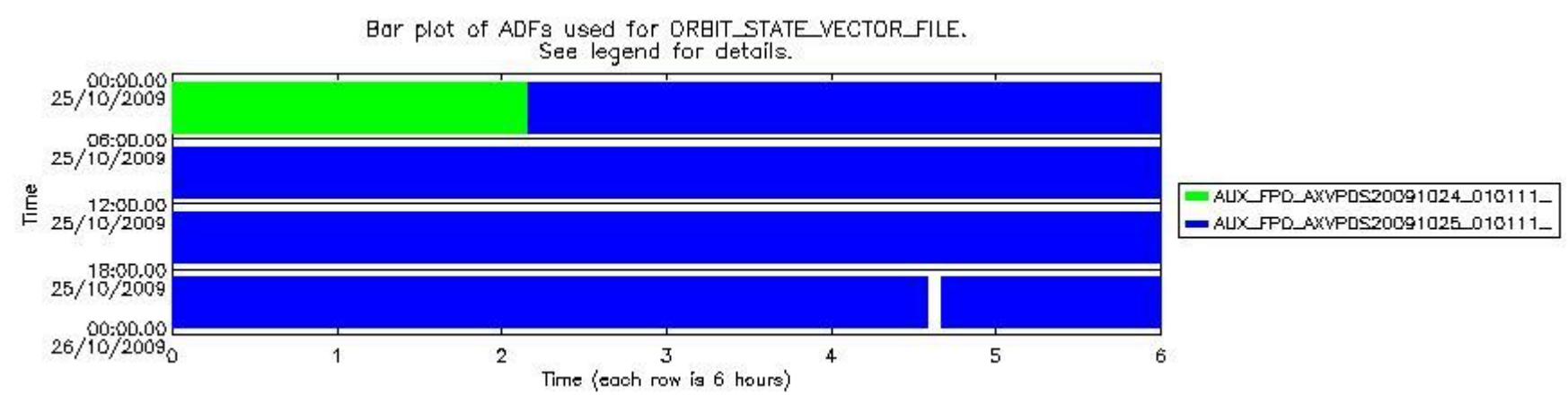
sciamachy_daily_report_level0_KSPT_L0_4303_N_20091025_7.PNG
