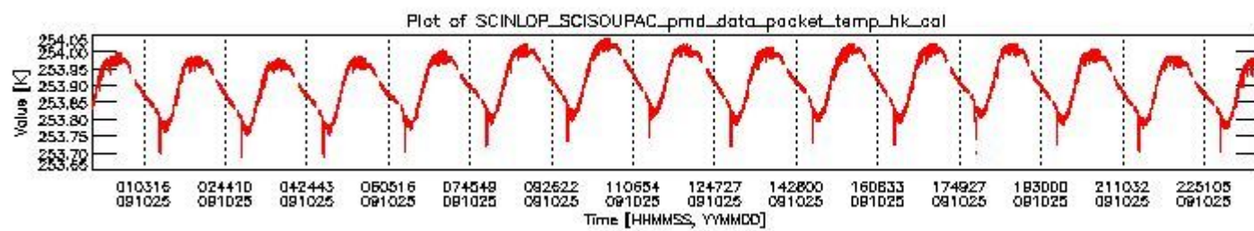
sciamachy_daily_report_level0_KSPT_L0_4303_N_20091025_3.PNG
