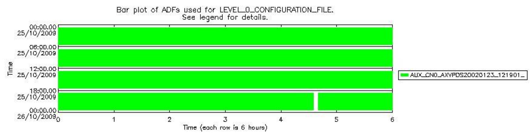
sciamachy_daily_report_level0_KSPT_L0_4303_N_20091025_6.PNG
