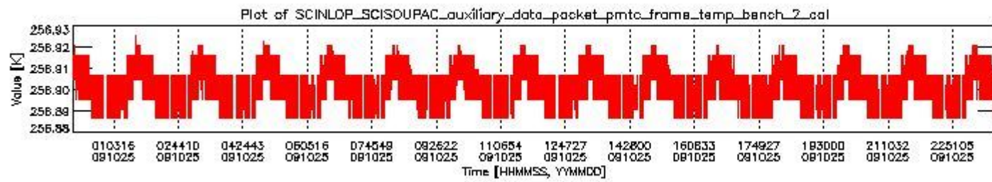
sciamachy_daily_report_level0_KSPT_L0_4303_N_20091025_1.PNG
