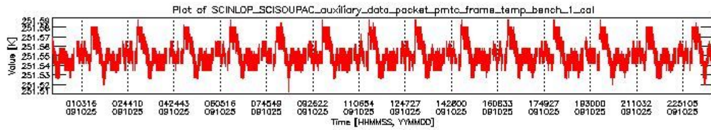
sciamachy_daily_report_level0_KSPT_L0_4303_N_20091025_0.PNG
