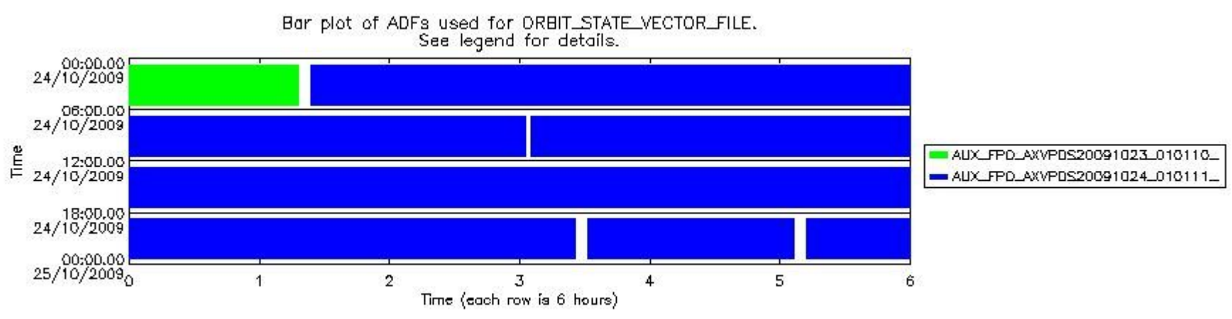
sciamachy_daily_report_level0_KSPT_L0_4303_N_20091024_7.PNG
