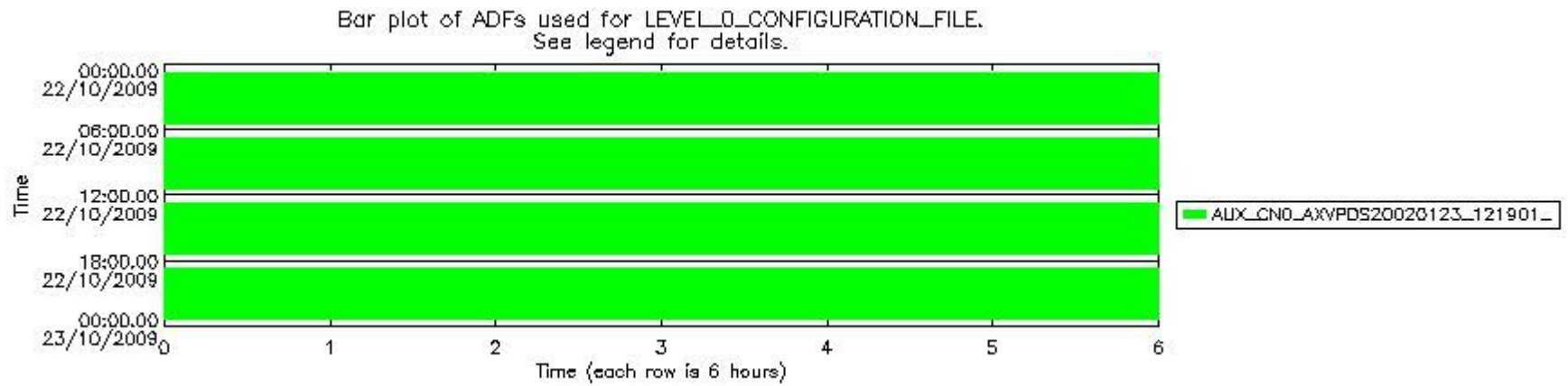
sciamachy_daily_report_level0_KSPT_L0_4303_N_20091022_6.PNG
