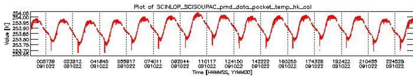
sciamachy_daily_report_level0_KSPT_L0_4303_N_20091022_3.PNG
