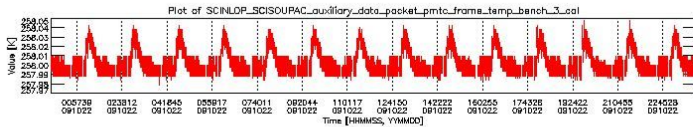
sciamachy_daily_report_level0_KSPT_L0_4303_N_20091022_2.PNG
