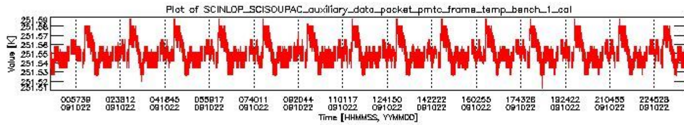
sciamachy_daily_report_level0_KSPT_L0_4303_N_20091022_0.PNG
