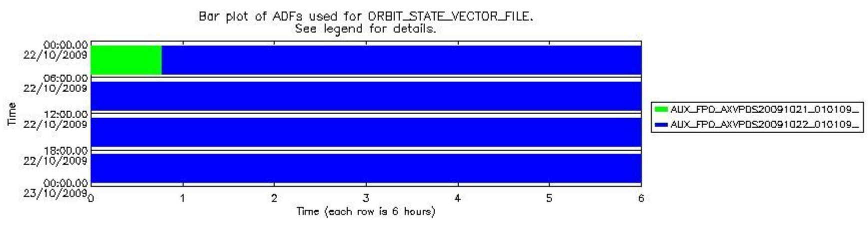
sciamachy_daily_report_level0_KSPT_L0_4303_N_20091022_7.PNG
