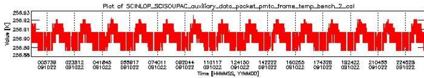
sciamachy_daily_report_level0_KSPT_L0_4303_N_20091022_1.PNG
