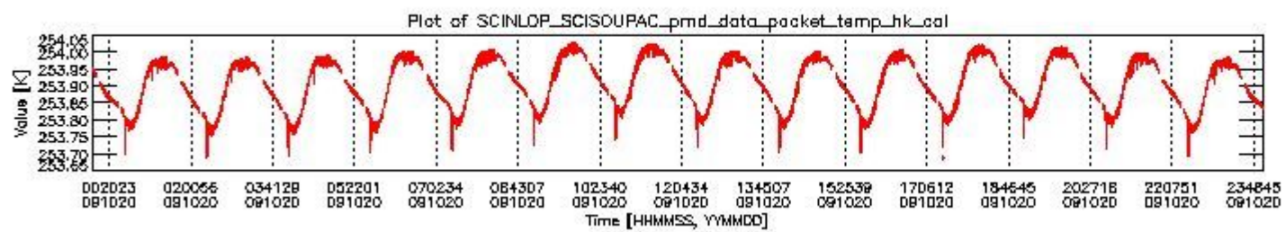
sciamachy_daily_report_level0_KSPT_L0_4303_N_20091020_3.PNG
