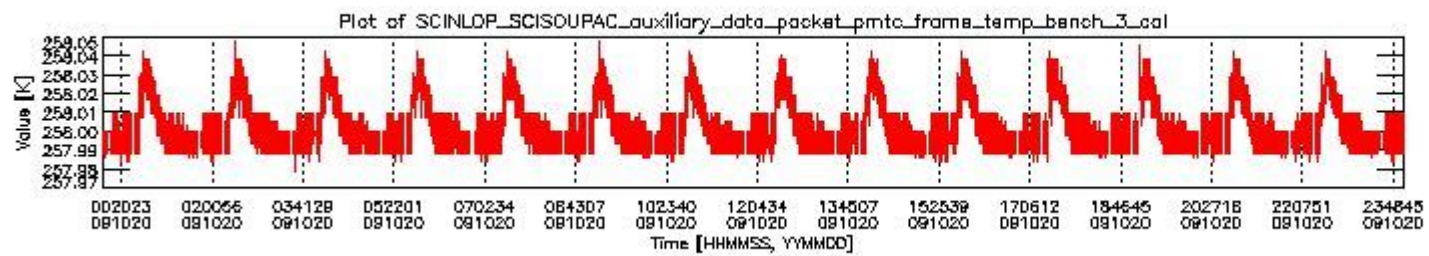
sciamachy_daily_report_level0_KSPT_L0_4303_N_20091020_2.PNG
