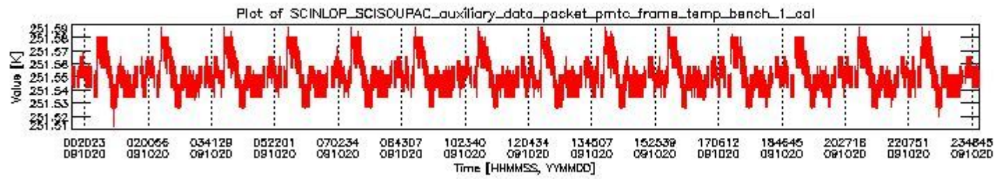
sciamachy_daily_report_level0_KSPT_L0_4303_N_20091020_0.PNG
