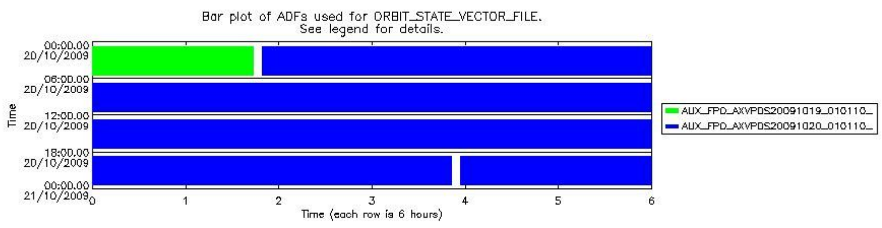
sciamachy_daily_report_level0_KSPT_L0_4303_N_20091020_7.PNG
