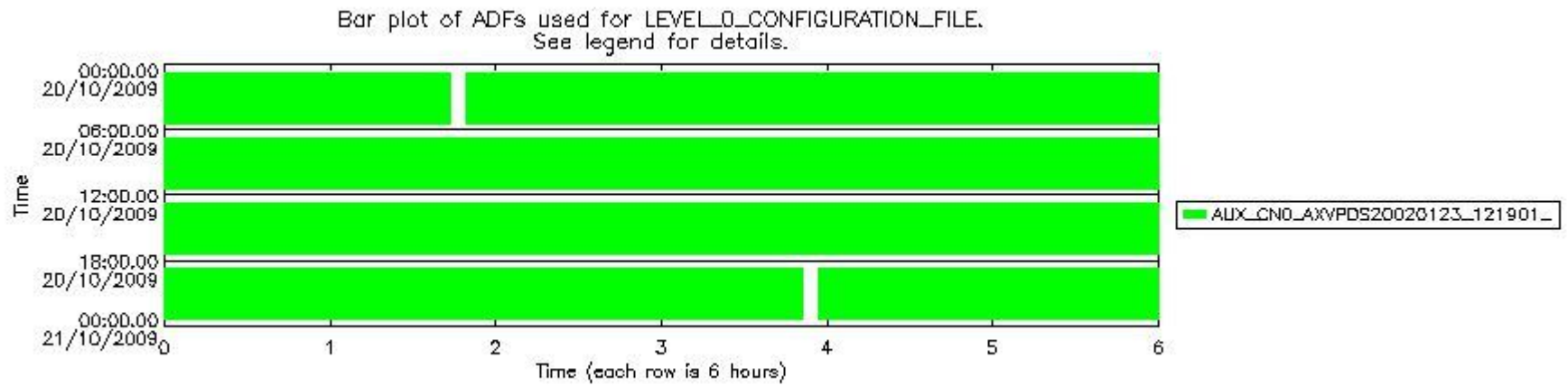
sciamachy_daily_report_level0_KSPT_L0_4303_N_20091020_6.PNG
