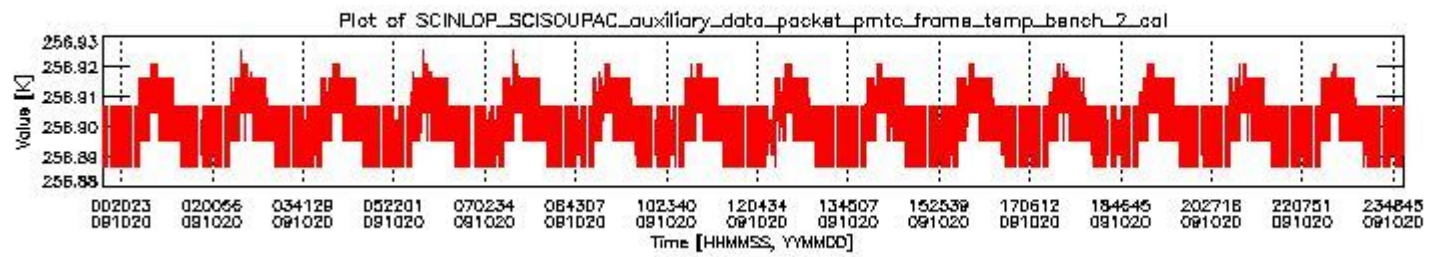
sciamachy_daily_report_level0_KSPT_L0_4303_N_20091020_1.PNG
