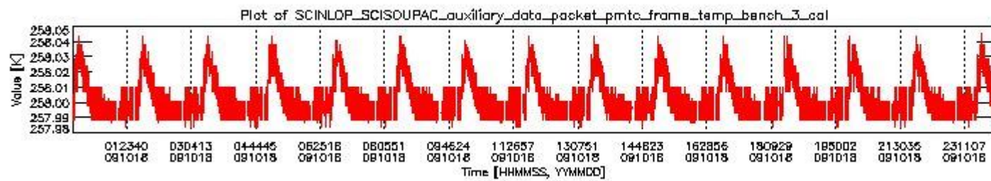
sciamachy_daily_report_level0_KSPT_L0_4303_N_20091018_2.PNG
