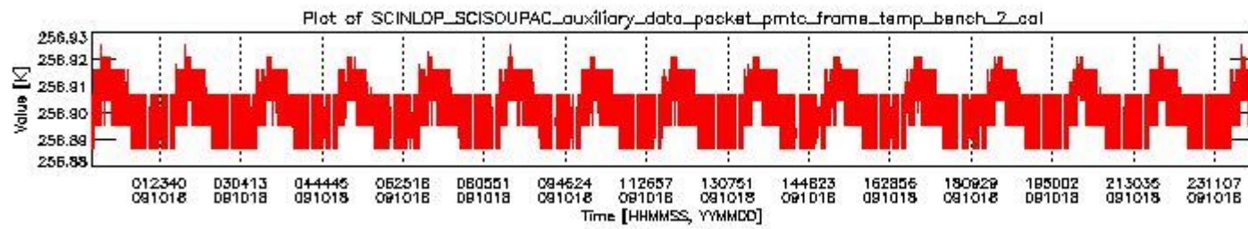
sciamachy_daily_report_level0_KSPT_L0_4303_N_20091018_1.PNG
