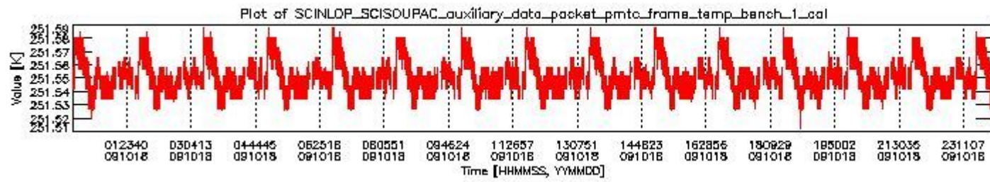
sciamachy_daily_report_level0_KSPT_L0_4303_N_20091018_0.PNG
