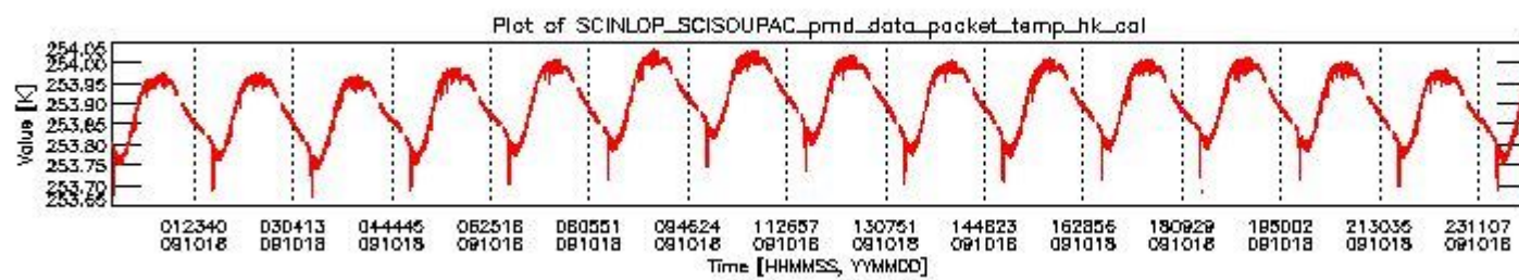
sciamachy_daily_report_level0_KSPT_L0_4303_N_20091018_3.PNG
