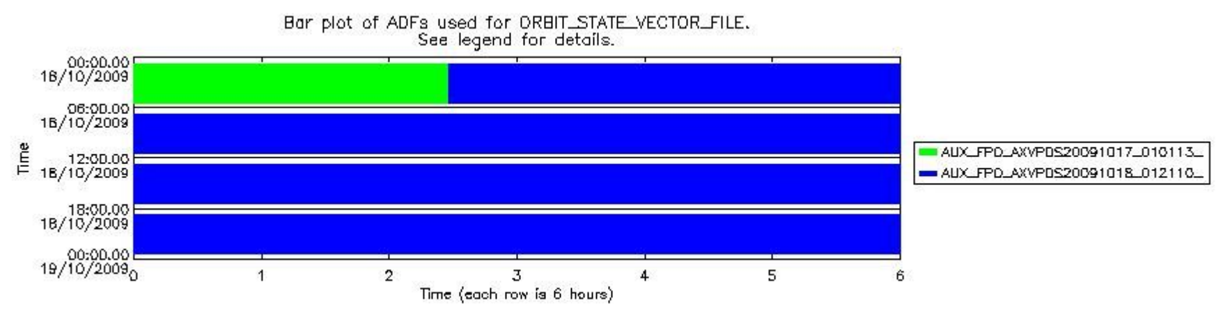
sciamachy_daily_report_level0_KSPT_L0_4303_N_20091018_7.PNG
