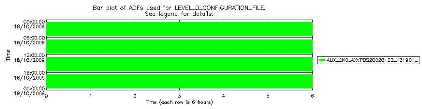
sciamachy_daily_report_level0_KSPT_L0_4303_N_20091018_6.PNG
