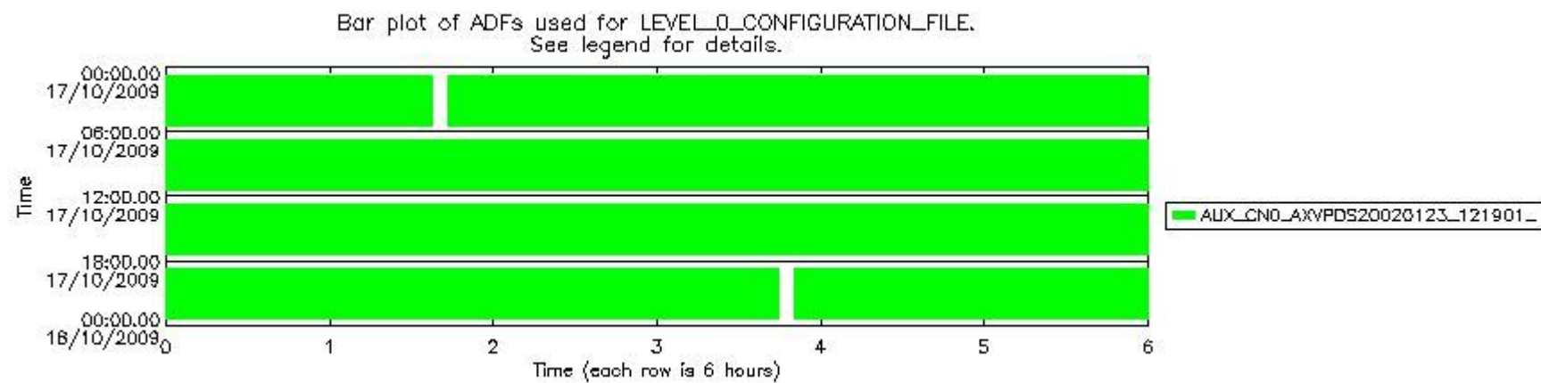
sciamachy_daily_report_level0_KSPT_L0_4303_N_20091017_6.PNG
