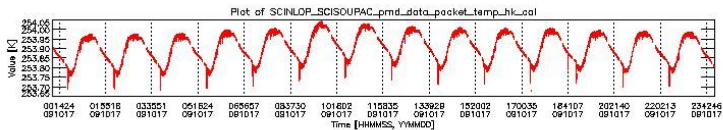
sciamachy_daily_report_level0_KSPT_L0_4303_N_20091017_3.PNG
