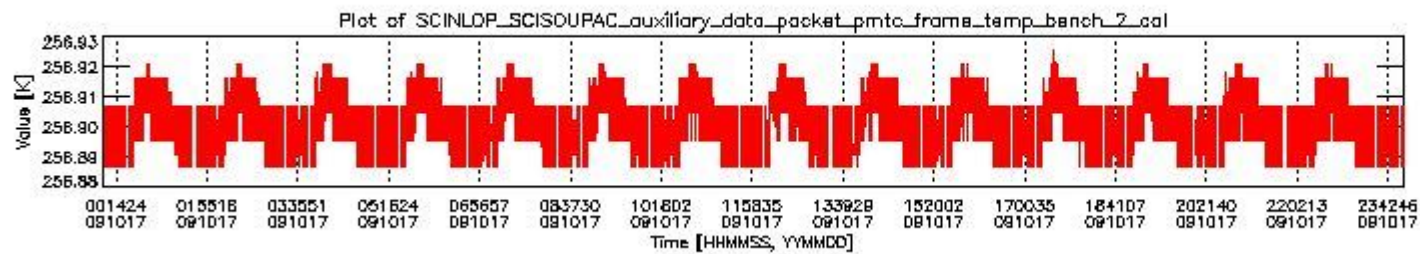
sciamachy_daily_report_level0_KSPT_L0_4303_N_20091017_1.PNG
