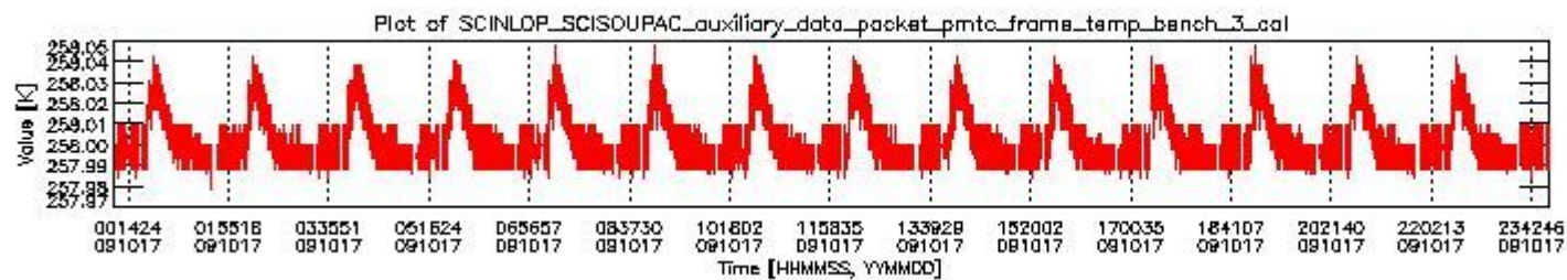
sciamachy_daily_report_level0_KSPT_L0_4303_N_20091017_2.PNG
