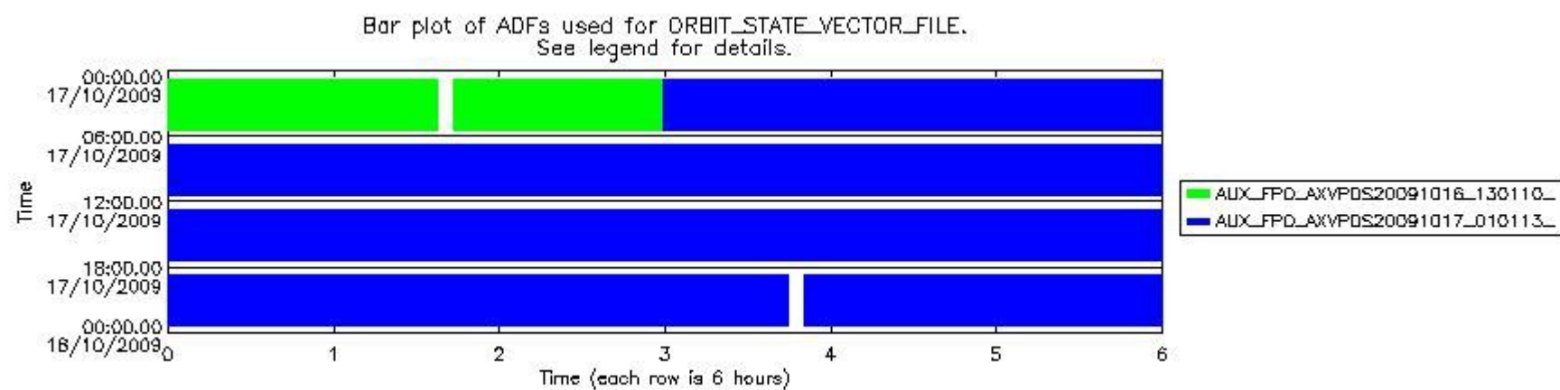
sciamachy_daily_report_level0_KSPT_L0_4303_N_20091017_7.PNG
