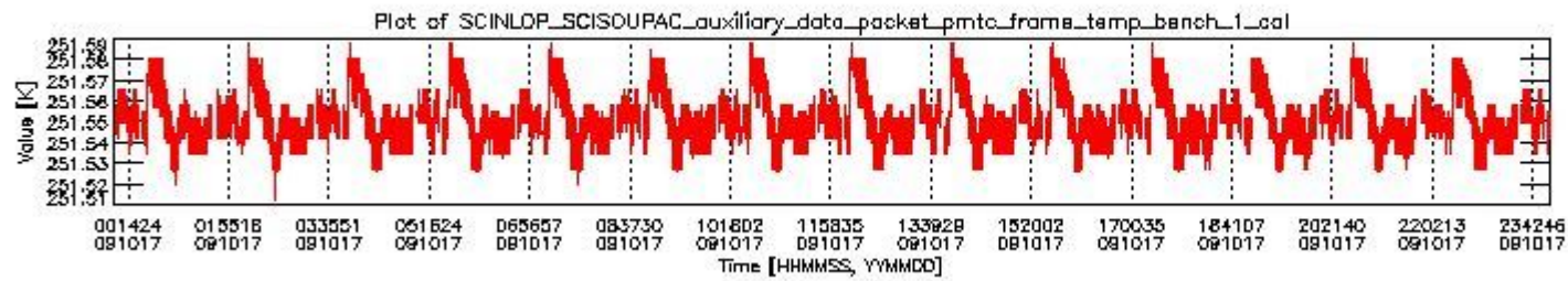
sciamachy_daily_report_level0_KSPT_L0_4303_N_20091017_0.PNG
