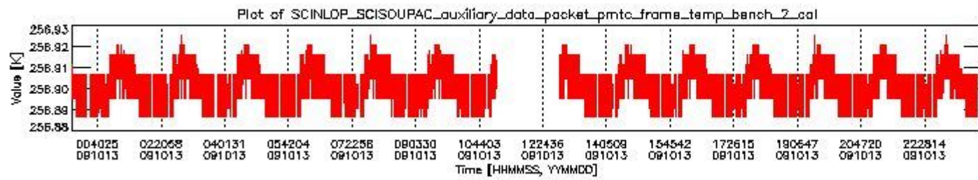
sciamachy_daily_report_level0_KSPT_L0_4303_N_20091013_1.PNG
