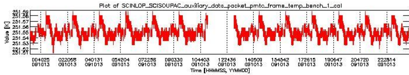
sciamachy_daily_report_level0_KSPT_L0_4303_N_20091013_0.PNG
