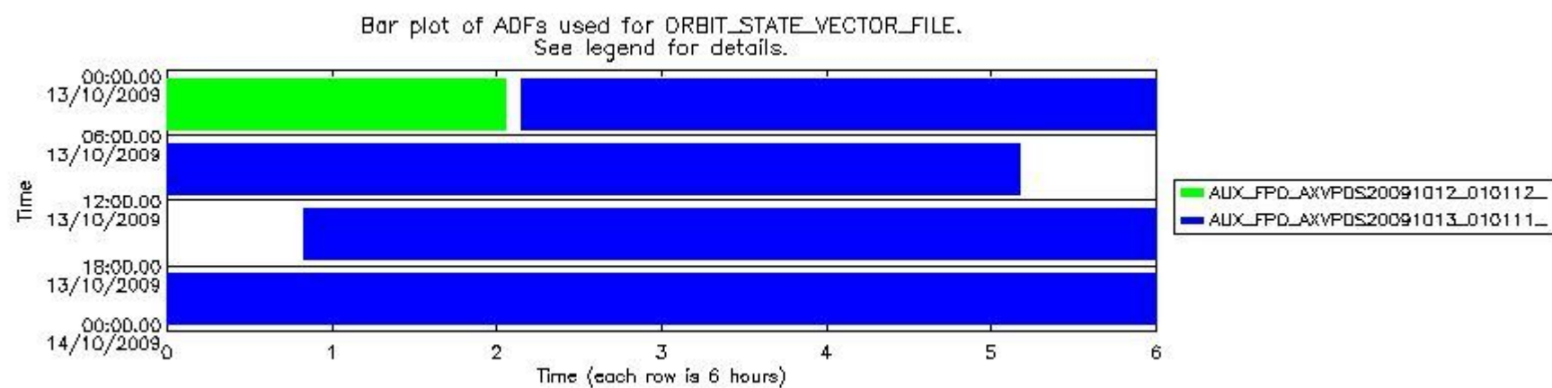
sciamachy_daily_report_level0_KSPT_L0_4303_N_20091013_7.PNG
