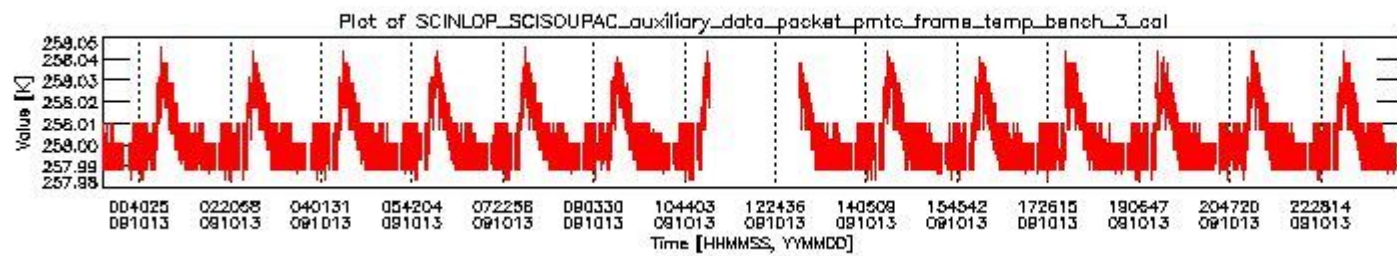
sciamachy_daily_report_level0_KSPT_L0_4303_N_20091013_2.PNG
