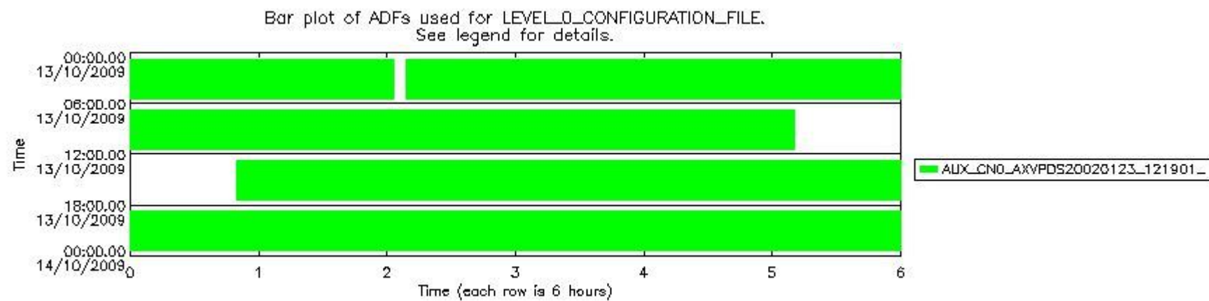
sciamachy_daily_report_level0_KSPT_L0_4303_N_20091013_6.PNG
