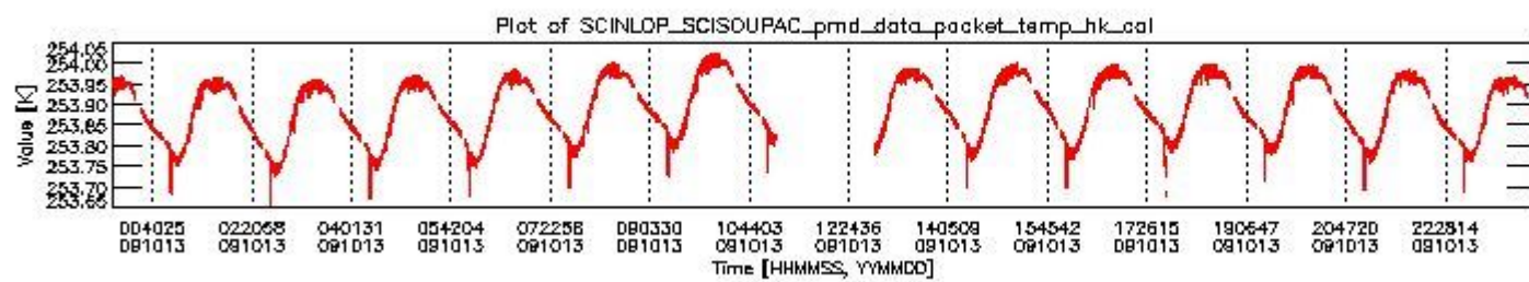
sciamachy_daily_report_level0_KSPT_L0_4303_N_20091013_3.PNG
