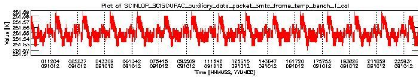
sciamachy_daily_report_level0_KSPT_L0_4303_N_20091012_0.PNG
