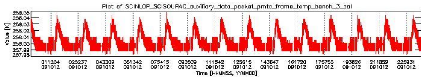
sciamachy_daily_report_level0_KSPT_L0_4303_N_20091012_2.PNG
