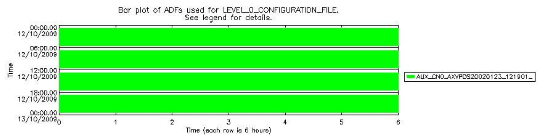
sciamachy_daily_report_level0_KSPT_L0_4303_N_20091012_6.PNG
