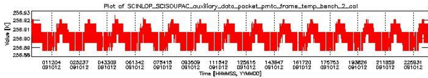
sciamachy_daily_report_level0_KSPT_L0_4303_N_20091012_1.PNG
