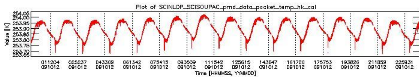
sciamachy_daily_report_level0_KSPT_L0_4303_N_20091012_3.PNG
