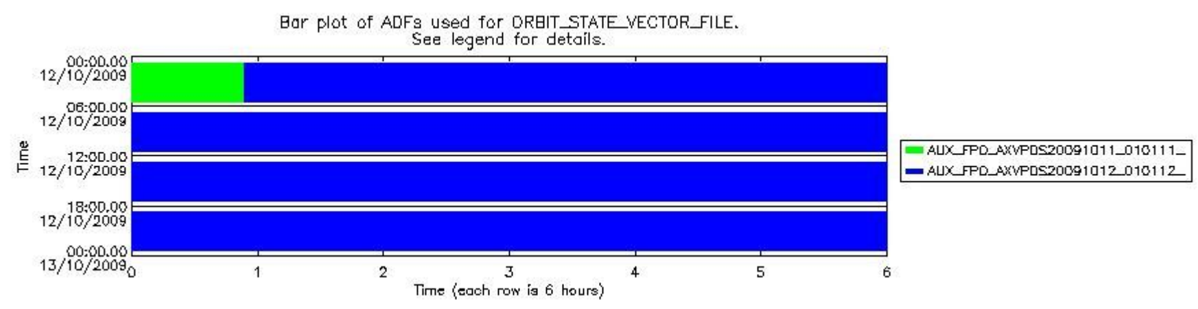
sciamachy_daily_report_level0_KSPT_L0_4303_N_20091012_7.PNG
