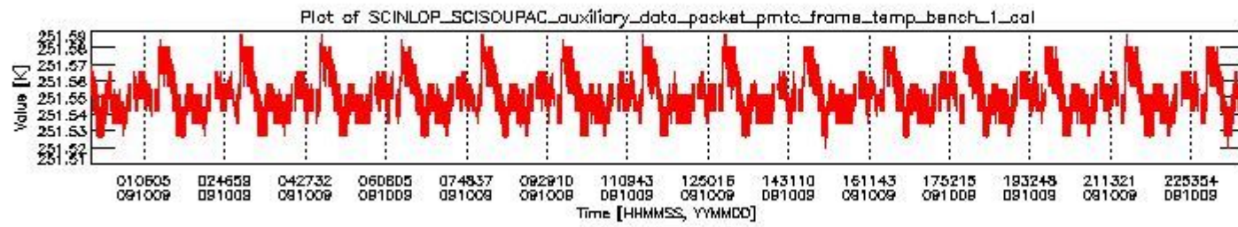
sciamachy_daily_report_level0_KSPT_L0_4303_N_20091009_0.PNG
