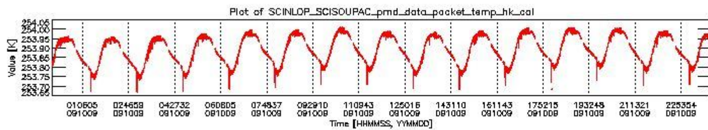
sciamachy_daily_report_level0_KSPT_L0_4303_N_20091009_3.PNG
