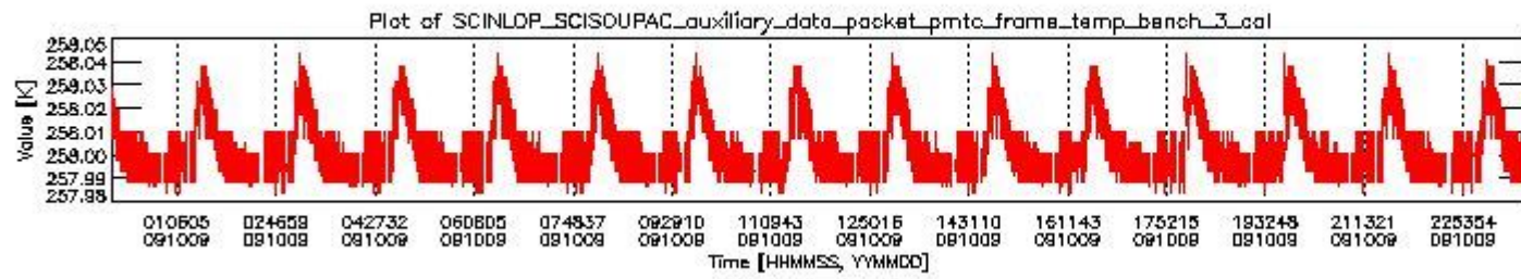
sciamachy_daily_report_level0_KSPT_L0_4303_N_20091009_2.PNG
