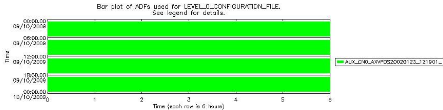
sciamachy_daily_report_level0_KSPT_L0_4303_N_20091009_6.PNG
