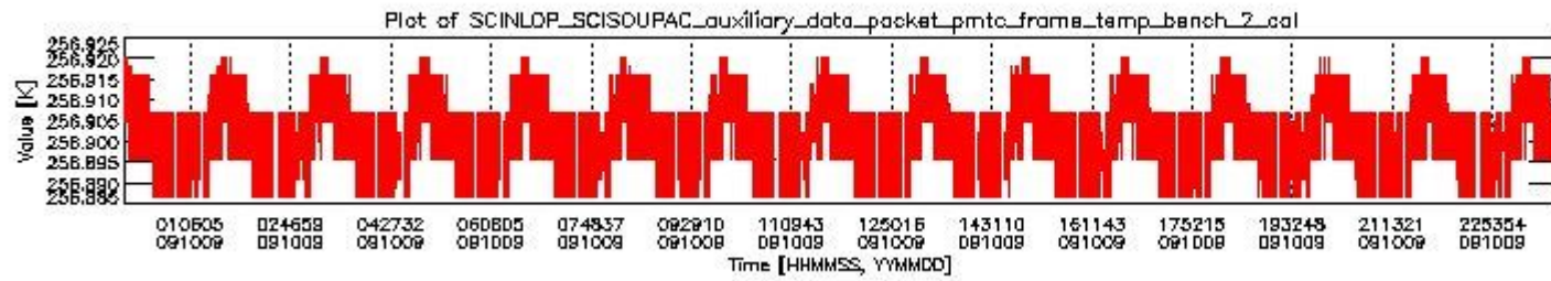
sciamachy_daily_report_level0_KSPT_L0_4303_N_20091009_1.PNG
