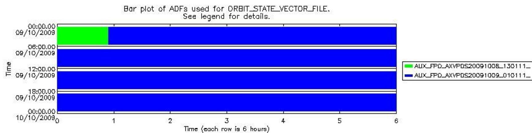
sciamachy_daily_report_level0_KSPT_L0_4303_N_20091009_7.PNG
