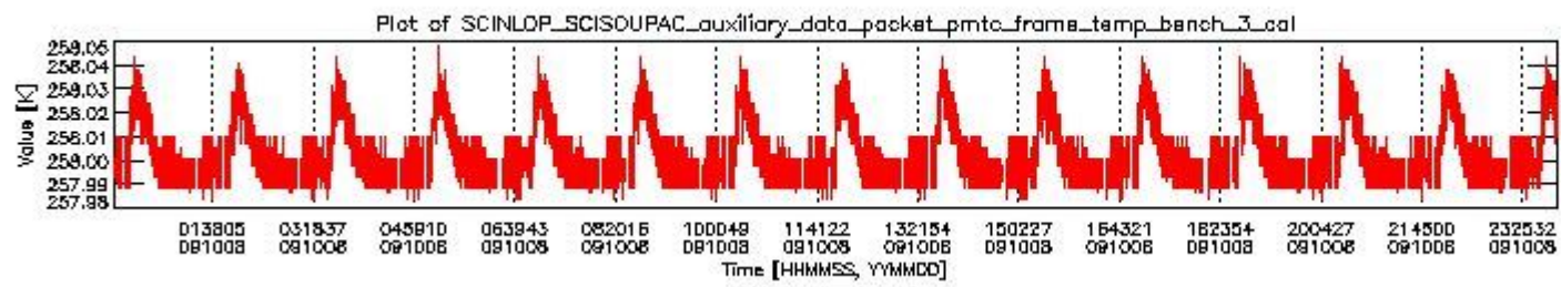
sciamachy_daily_report_level0_KSPT_L0_4303_N_20091008_2.PNG
