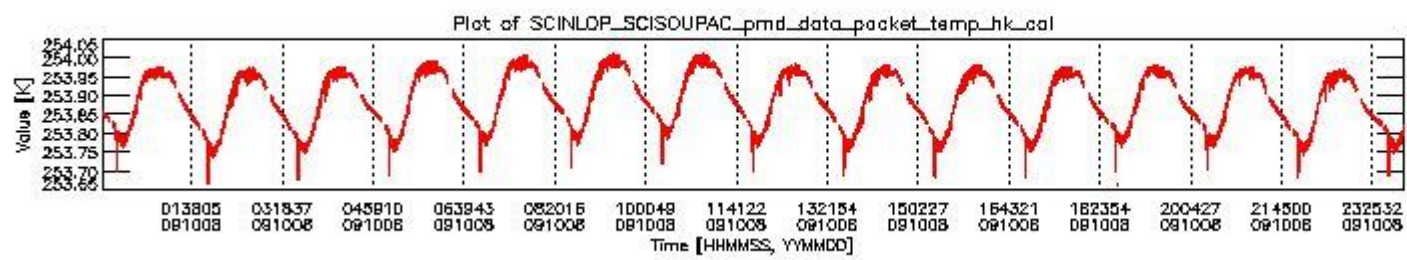
sciamachy_daily_report_level0_KSPT_L0_4303_N_20091008_3.PNG
