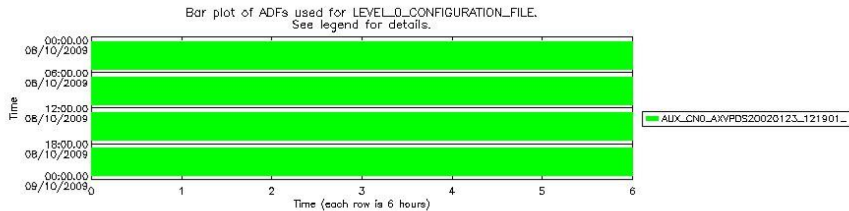
sciamachy_daily_report_level0_KSPT_L0_4303_N_20091008_6.PNG
