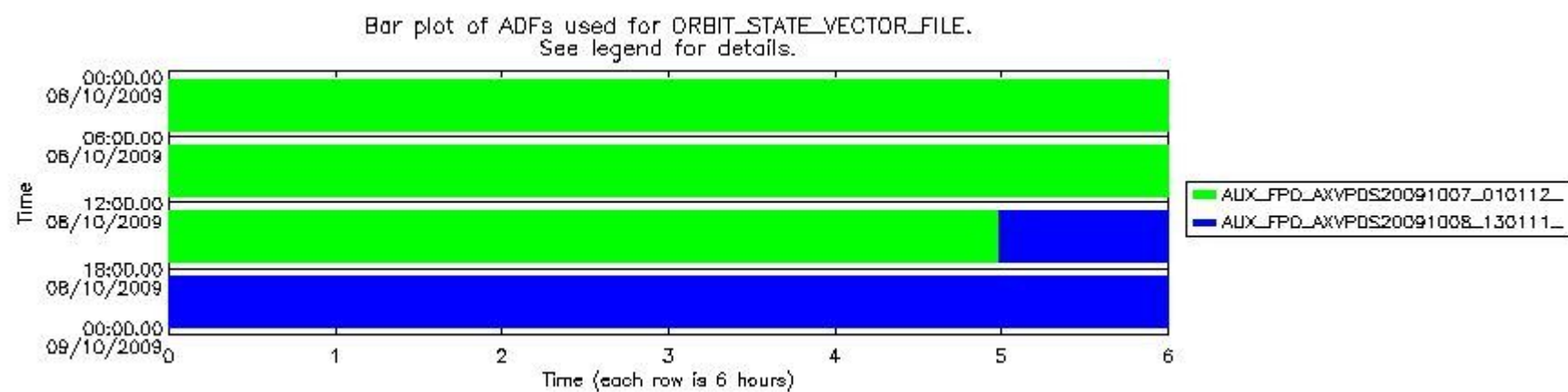
sciamachy_daily_report_level0_KSPT_L0_4303_N_20091008_7.PNG
