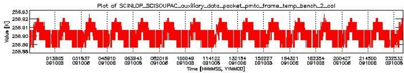
sciamachy_daily_report_level0_KSPT_L0_4303_N_20091008_1.PNG
