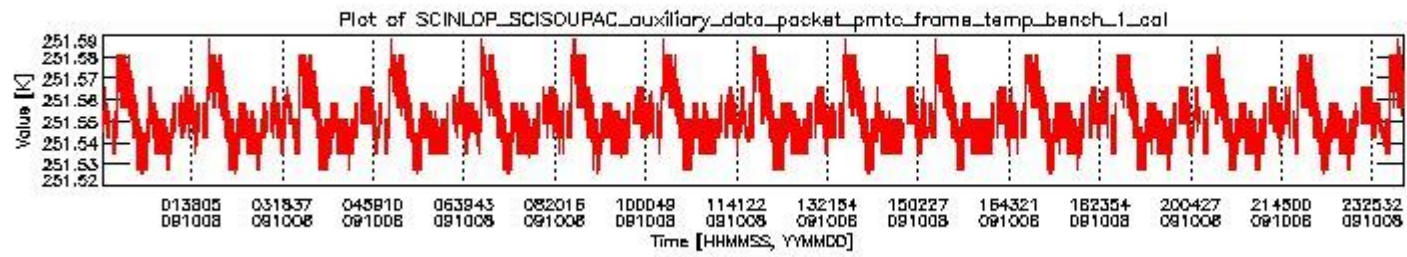
sciamachy_daily_report_level0_KSPT_L0_4303_N_20091008_0.PNG
